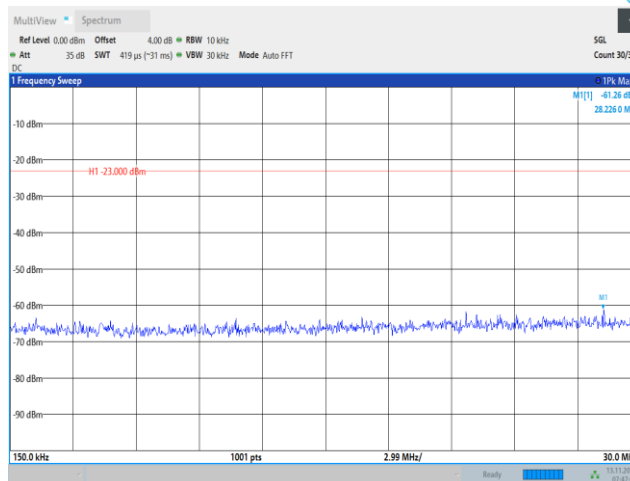
Band4-20MHz-QPSK-20050-1RB#0-Range2:0.15~30MHz
