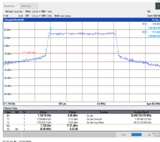
NTNV_N66_PC3_15_35_M_TID5_Ant14#1
