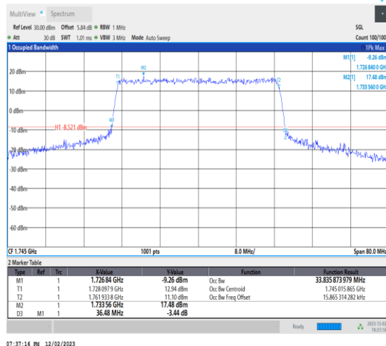
NTNV_N66_PC3_15_35_M_TID8_Ant14#1
