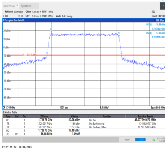
NTNV_N66_PC3_15_35_M_TID7_Ant14#1
