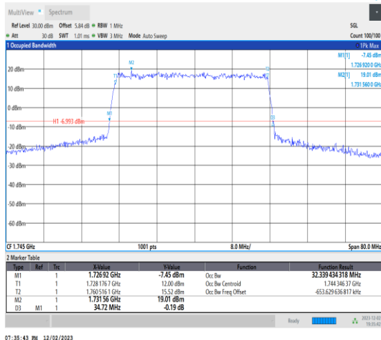
NTNV_N66_PC3_15_35_M_TID3_Ant14#1
