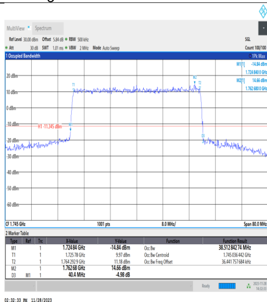
NTNV_N66_PC3_15_40_M_TID6_Ant14#1
