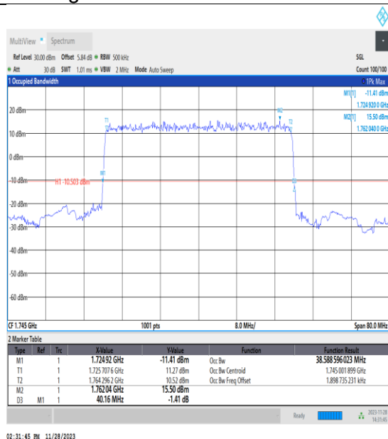
NTNV_N66_PC3_15_40_M_TID2_Ant14#1
