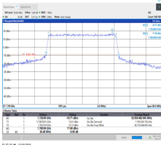
NTNV_N66_PC3_15_35_M_TID9_Ant14#1
