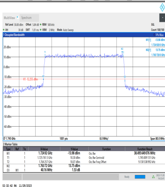
NTNV_N66_PC3_15_40_M_TID7_Ant14#1
