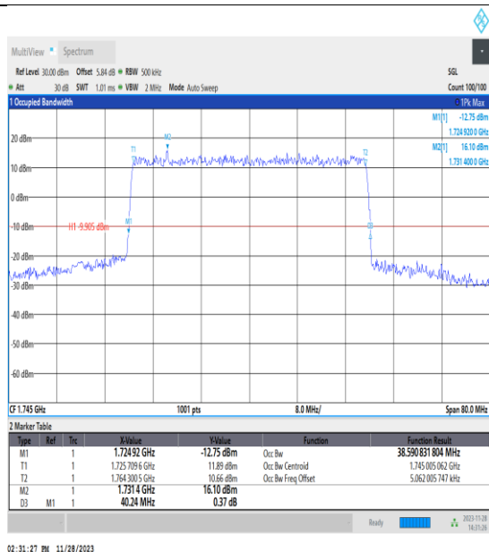
NTNV_N66_PC3_15_40_M_TID1_Ant14#1
