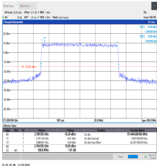
NTVN_N77-3700-3980_PC3_30_100_M_TID7_Ant13#1
