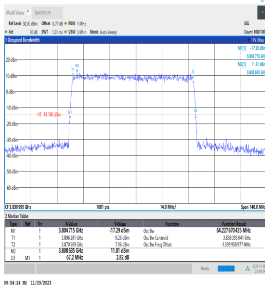
NTNV_N77-3700-3980_PC3_30_70_M_TID5_Ant13#1
