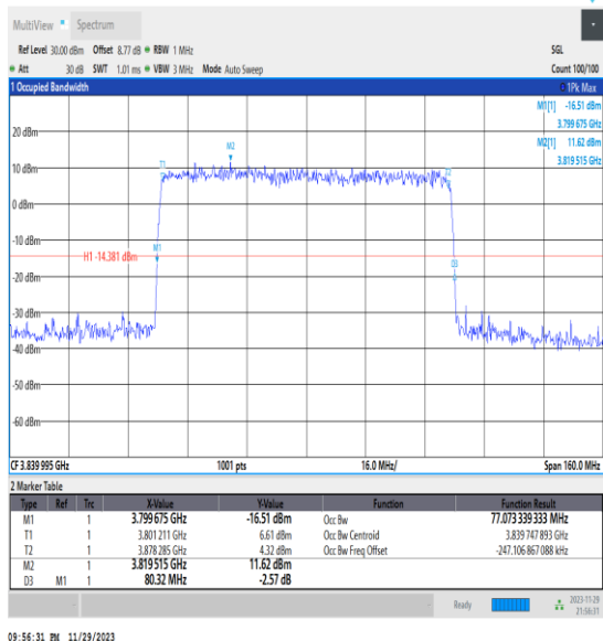
NTNV_N77-3700-3980_PC3_30_80_M_TID5_Ant13#1
