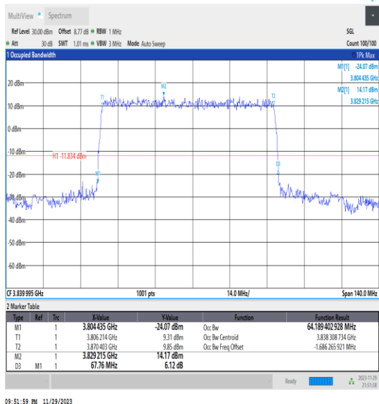
NTNV_N77-3700-3980_PC3_30_70_M_TID2_Ant13#1
