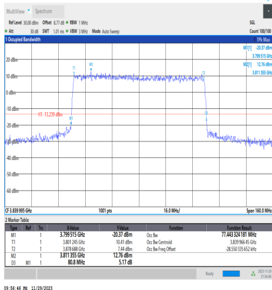
NTNV_N77-3700-3980_PC3_30_80_M_TID6_Ant13#1
