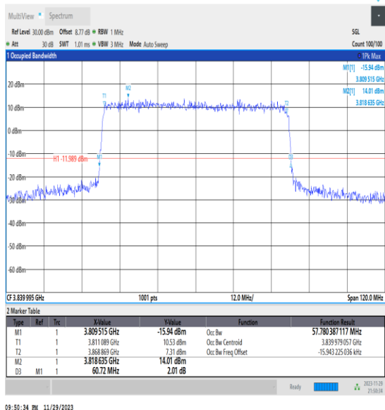
NTNV_N77-3700-3980_PC3_30_60_M_TID7_Ant13#1
