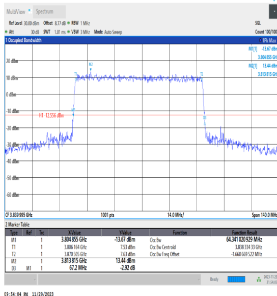
NTNV_N77-3700-3980_PC3_30_70_M_TID3_Ant13#1
