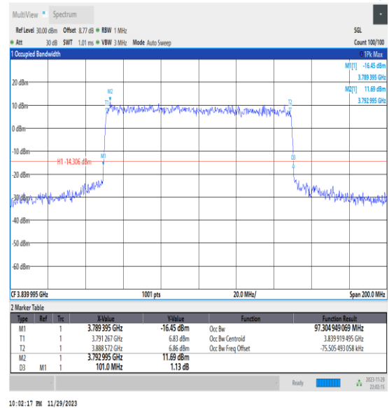
NTVN_N77-3700-3980_PC3_30_100_M_TID6_Ant13#1
