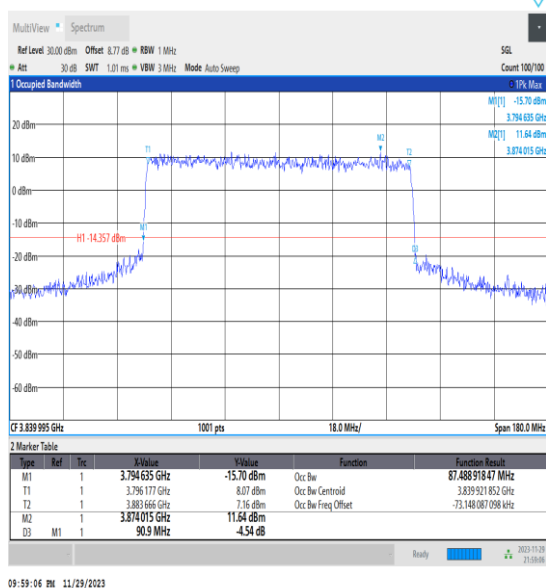
NTNV_N77-3700-3980_PC3_30_90_M_TID7_Ant13#1
