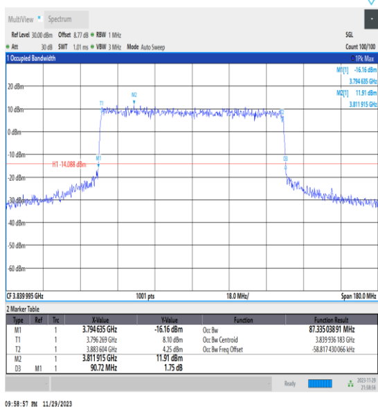
NTNV_N77-3700-3980_PC3_30_90_M_TID6_Ant13#1
