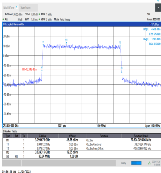
NTNV_N77-3700-3980_PC3_30_80_M_TID7_Ant13#1
