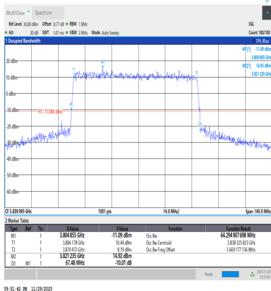
NTNV_N77-3700-3980_PC3_30_70_M_TID1_Ant13#1
