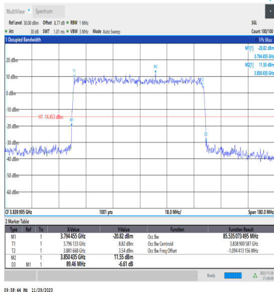
NTNV_N77-3700-3980_PC3_30_90_M_TID5_Ant13#1
