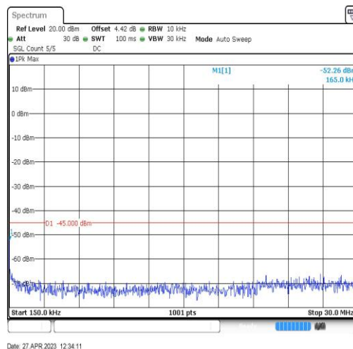
Band41-20MHz-QPSK-41490-1RB#0-Range2:0.15~30MHz
