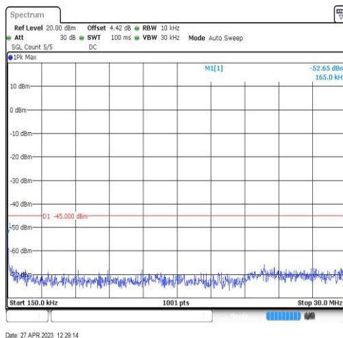
Band41-20MHz-QPSK-39750-1RB#0-Range2:0.15~30MHz
