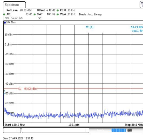
Band41-20MHz-QPSK-40620-1RB#0-Range2:0.15~30MHz
