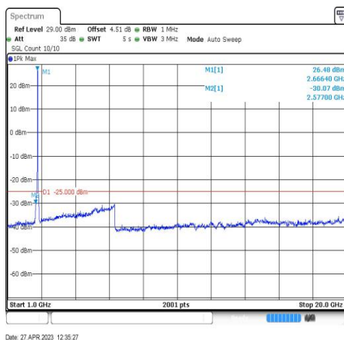
Band41-20MHz-QPSK-41490-1RB#0-Range4:1000~20000MHz
