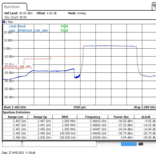
Band41-10MHz-QPSK-39700-50RB#0
