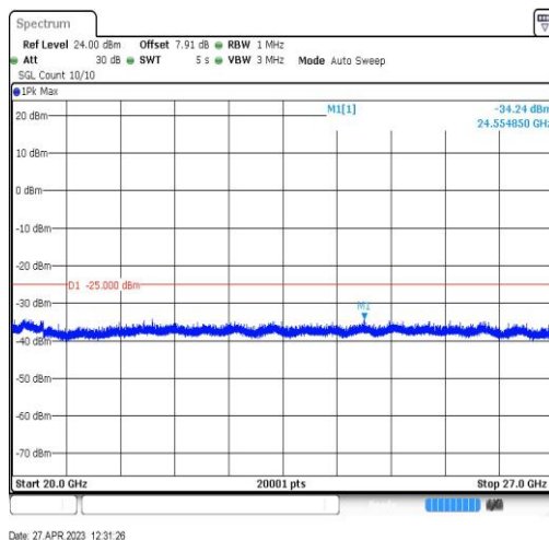
Band41-20MHz-QPSK-39750-1RB#0-Range5:20000~27000MHz
