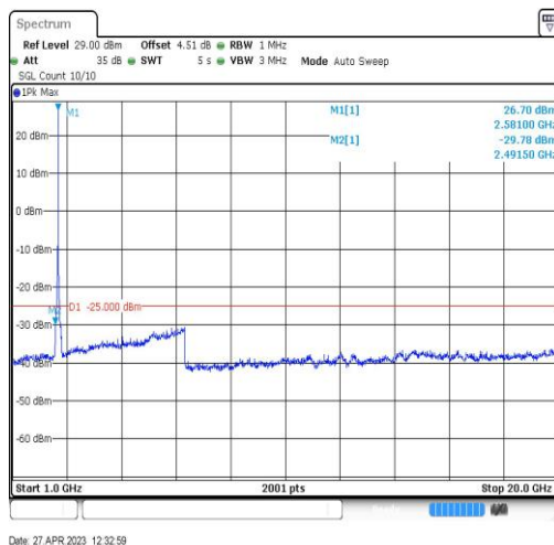
Band41-20MHz-QPSK-40620-1RB#0-Range4:1000~20000MHz
