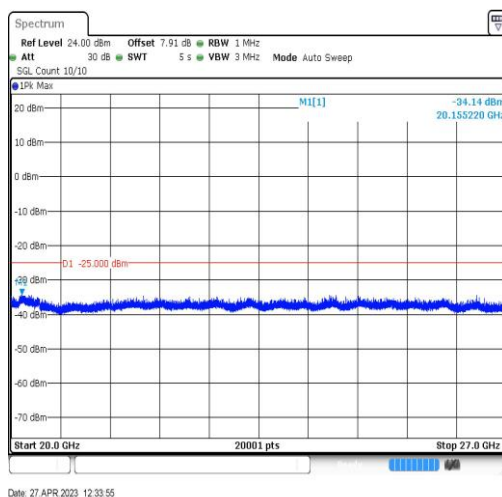
Band41-20MHz-QPSK-40620-1RB#0-Range5:20000~27000MHz
