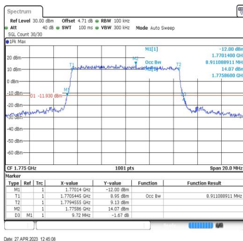
Band66-10MHz-QPSK-132622-50RB#0-8.911
