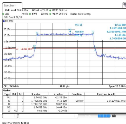
Band66-10MHz-QPSK-132322-50RB#0-8.951
