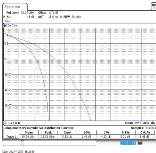
Band66-20MHz-QPSK-132572-100RB#0
