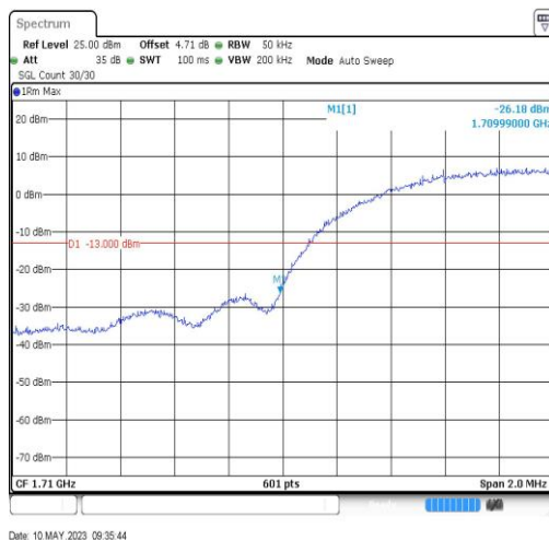
BandIV-1312-1709.99
