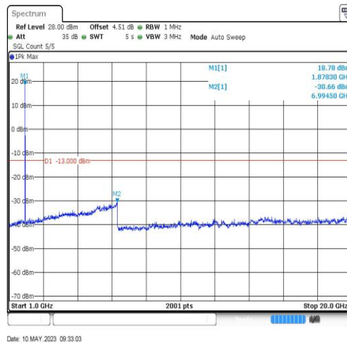
BandII-9400-1000~20000MHz-6994.5
