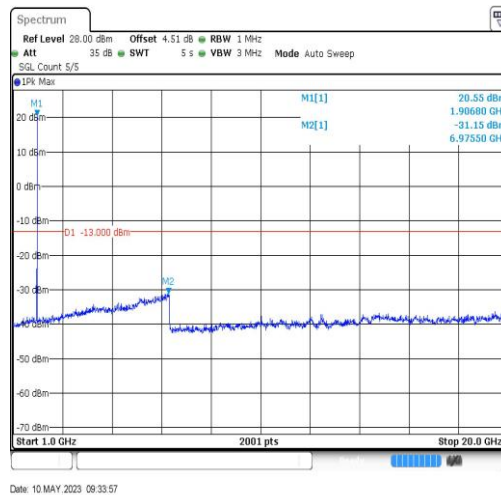
BandII-9538-1000~20000MHz-6975.5
