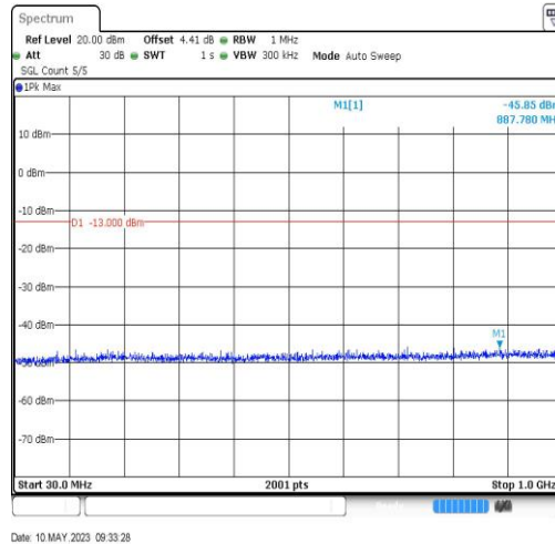
BandII-9538-30~1000MHz-887.78
