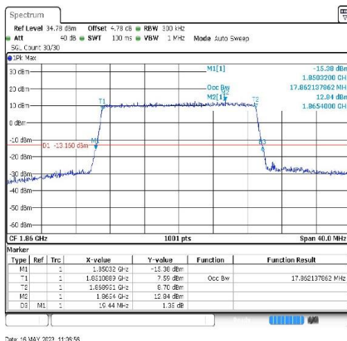
Band2-20MHz-16QAM-18700-100RB#0-18.062
