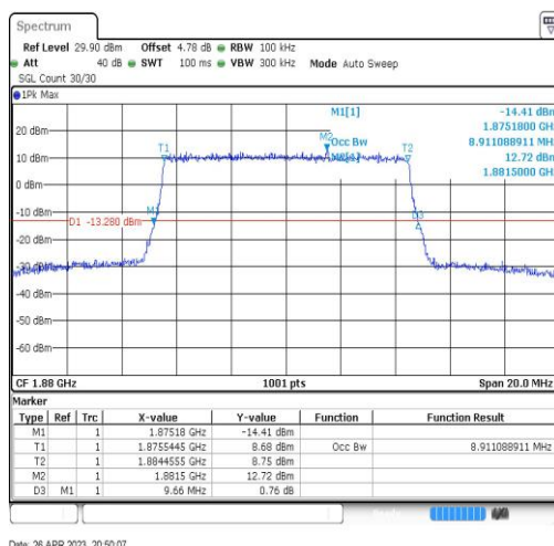
Band2-10MHz-16QAM-18900-50RB#0-8.911
