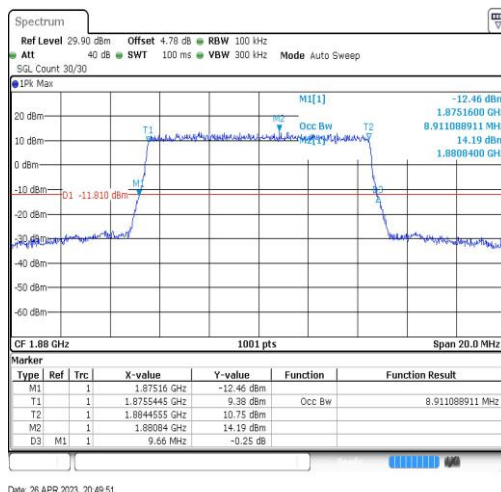
Band2-10MHz-QPSK-18900-50RB#0-8.911
