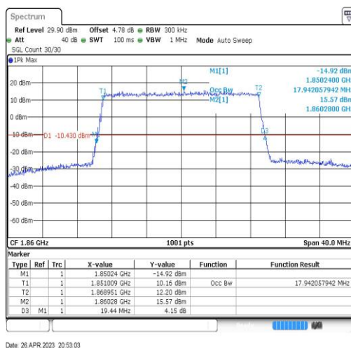
Band2-20MHz-QPSK-18700-100RB#0-17.942
