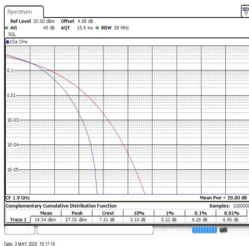
Band2-20MHz-16QAM-19100-100RB#0
