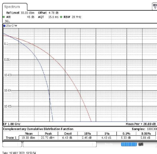
Band2-20MHz-QPSK-18900-100RB#0
