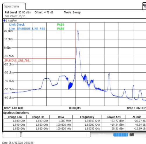
Band2-5MHz-QPSK-18625-1RB#0
