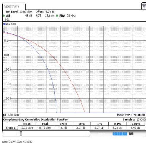
Band2-20MHz-16QAM-18900-100RB#0
