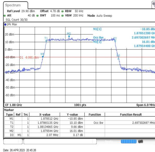
Band2-3MHz-QPSK-18900-15RB#0-2.697
