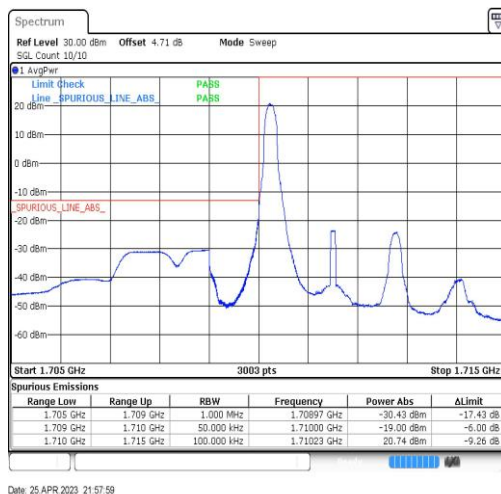
Band4-3MHz-QPSK-19965-1RB#0
