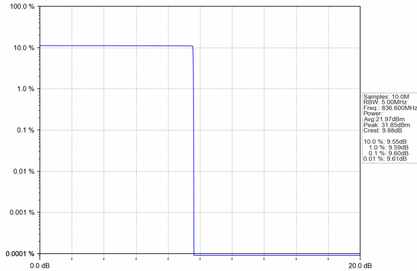
GSM850_GSM_MCH_836.6MHz_GSM_NTNV
