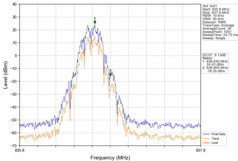
GSM850_GSM_MCH_836.6MHz_GSM_NTNV
