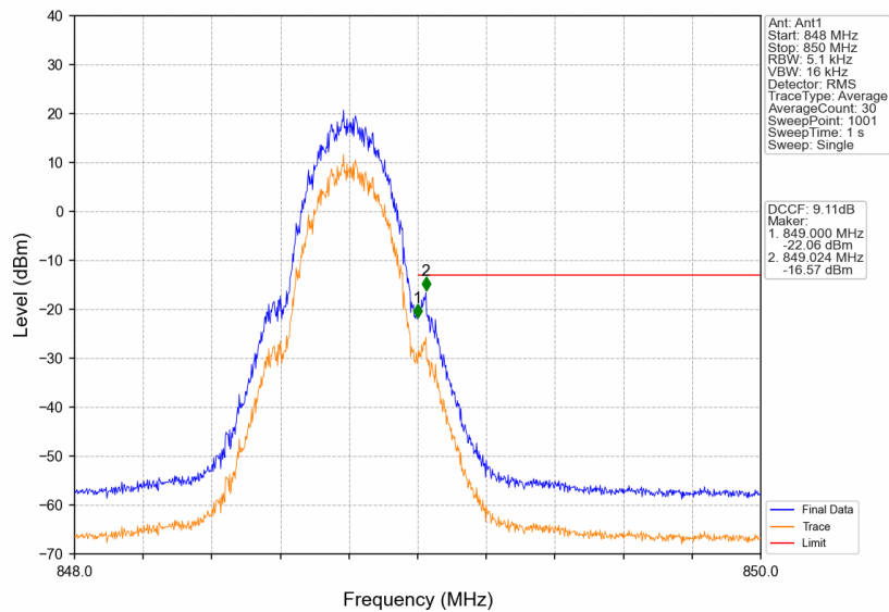
GSM850_GSM_HCH_848.8MHz_GSM_NTNV
