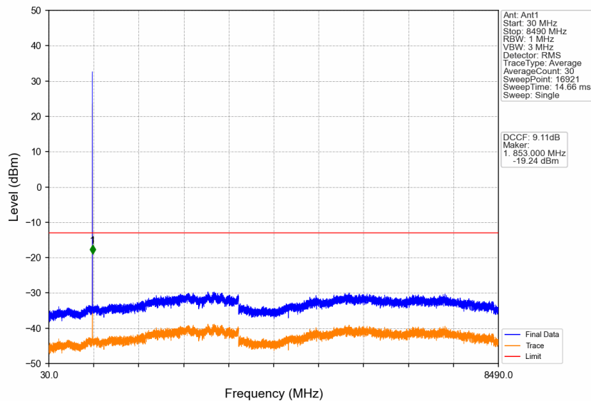
GSM850_GSM_HCH_848.8MHz_GSM_NTNV
