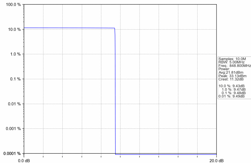
GSM850_GSM_HCH_848.8MHz_GSM_NTNV
