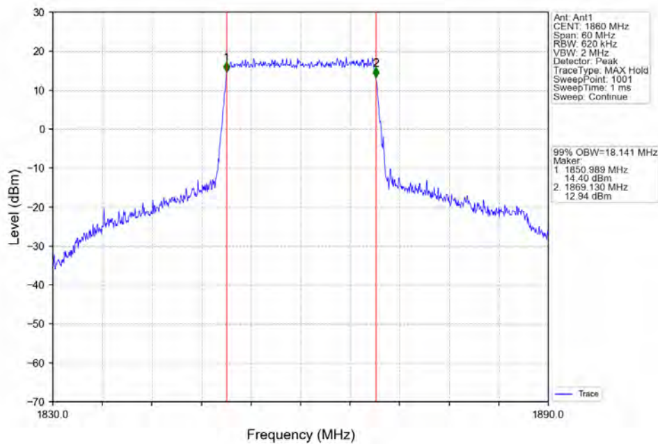
Band2_20MHz_QPSK_LCH_1860MHz_RB_100_0_NTNV
