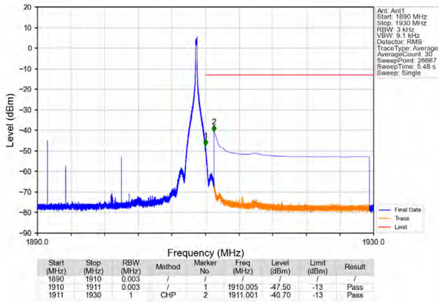
Band2_20MHz_64QAM_HCH_1900MHz_RB_1_99_NTNV
