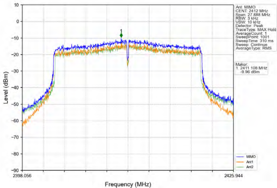
802.11ax(HEW20) LCH 2412MHz RU242 Left MIMO NTN
