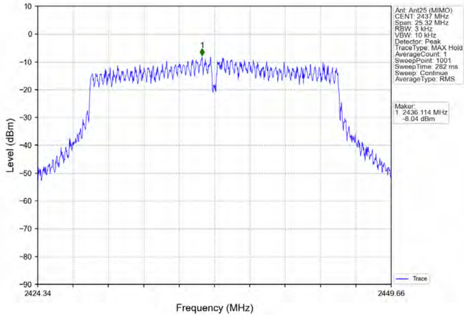
802.11ac(VHT20)_MCH_2437MHz_MIMO_NTNV
