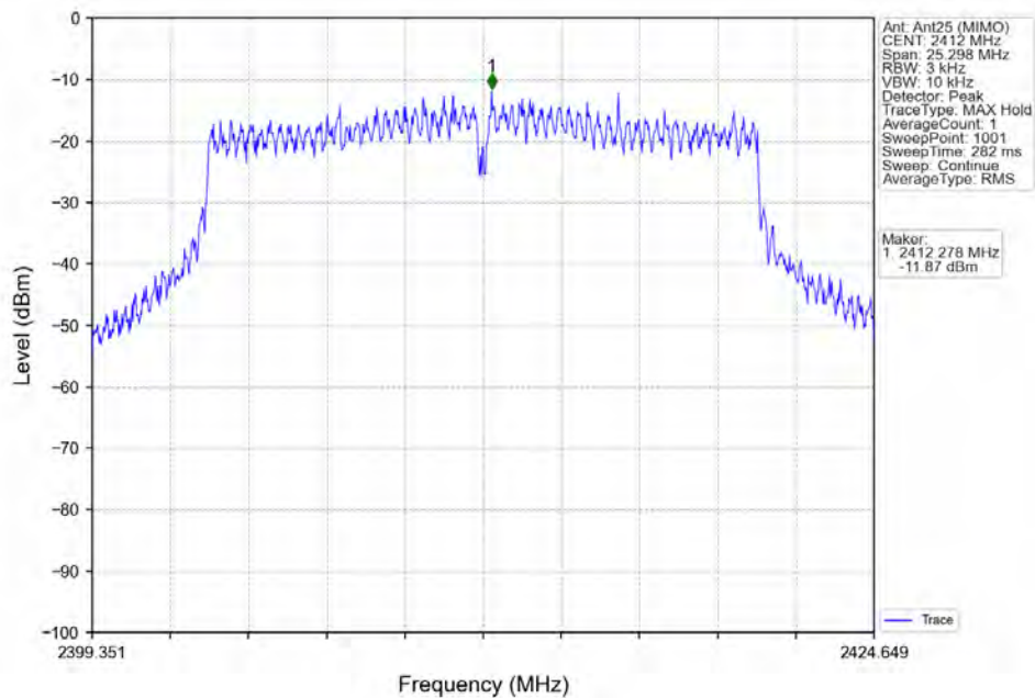
802.11n(HT20) LCH 2412MHz Ant25 (MIMO) NTV
