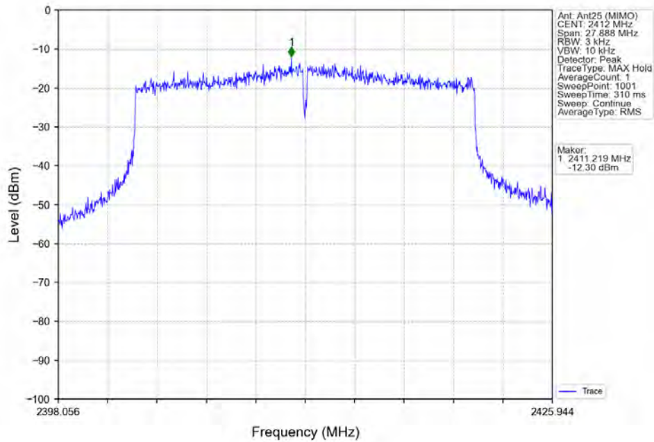
802.11ax(HEW20) LCH 2412MHz RU242 Left MIMO NTN
