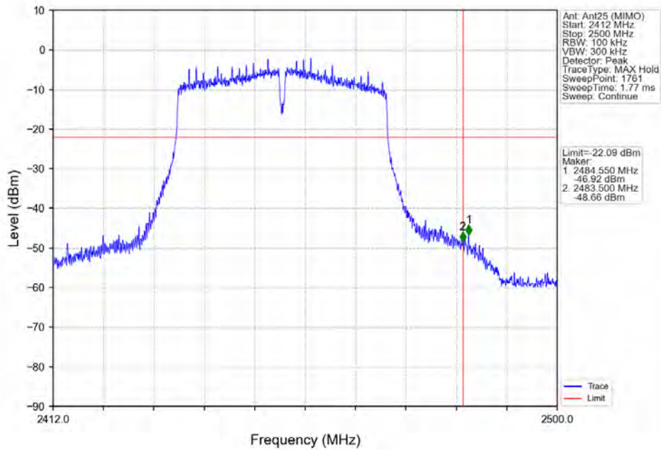
802.11ac(VHT40) HCH 2452MHz Ant25 (MIMO) NTNV
