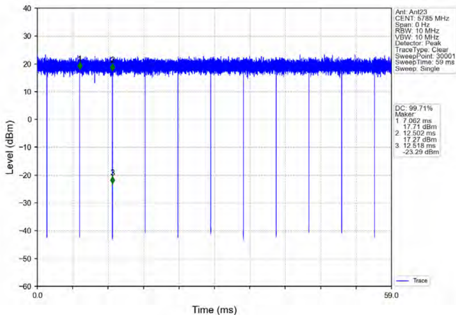
802.11ax(HE20) MCH 5785MHz RU242 Left Ant23 NTNV
