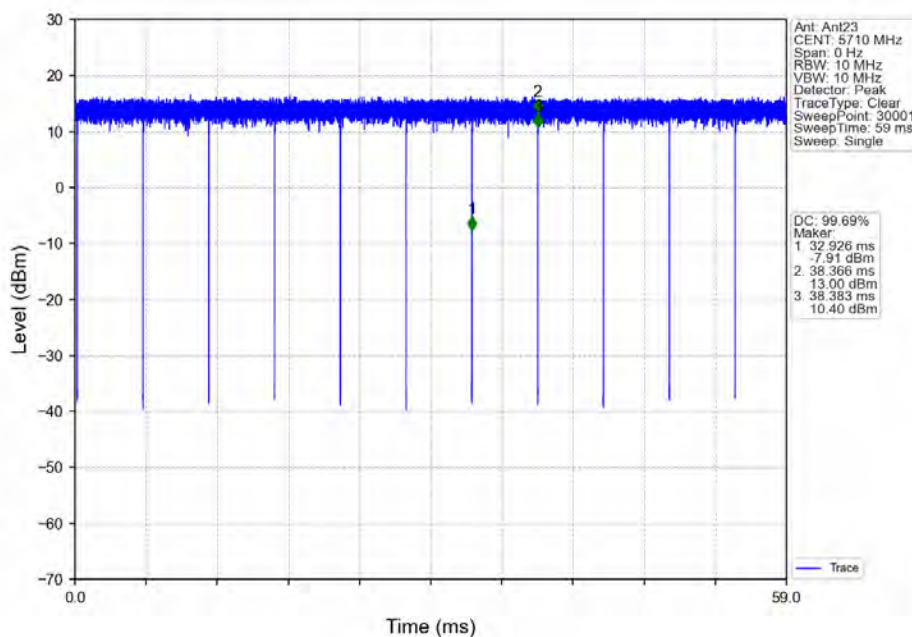
802.11ax(HE40) HCH 5710MHz RU484 Left Ant23 NTNV
