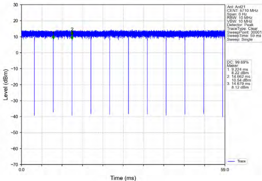
802.11ax(HE40) HCH 5710MHz RU484 Left Ant21 NTN
