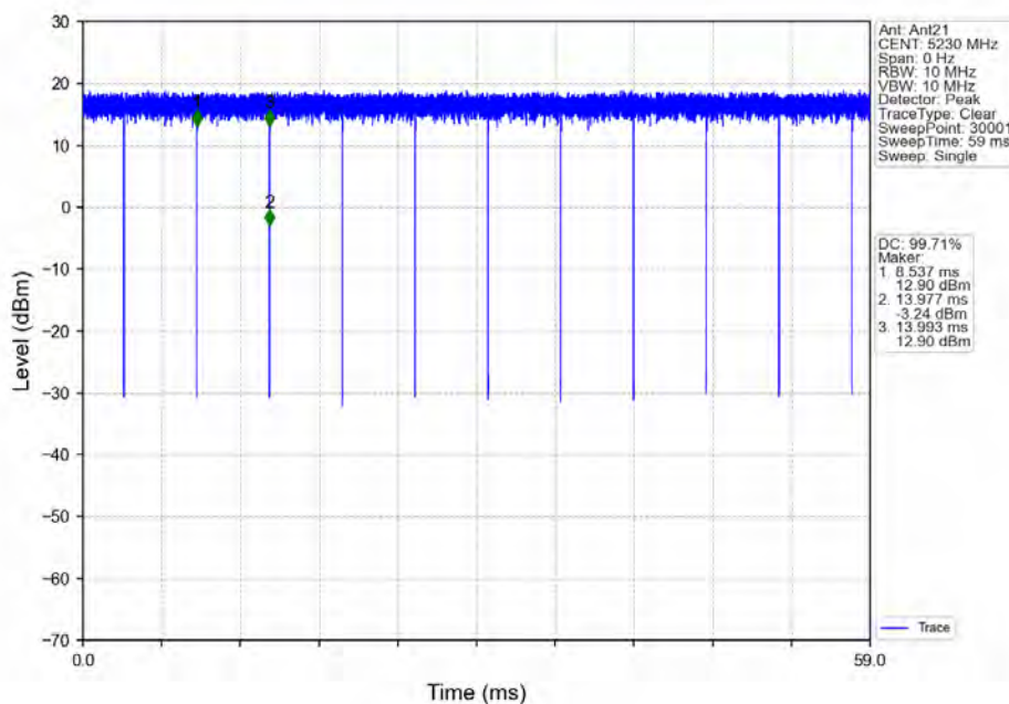
802.11ax(HE40) HCH 5230MHz RU484 Left Ant21 NTN
