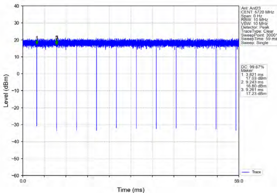
802.11n(HT20) HCH 5720MHz Ant23 NTN
