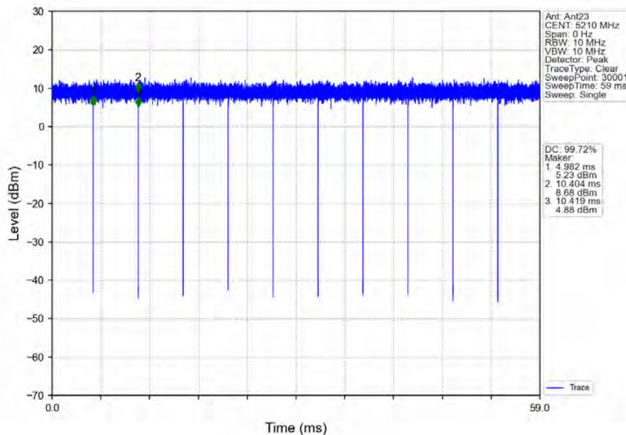
802.11ac(VHT80)_MCH_5210MHz_Ant23_NTNV
