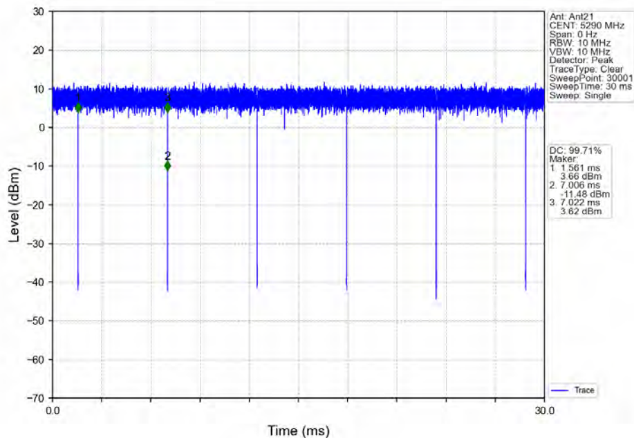
802.11ax(HE80) MCH 5290MHz RU996 Left Ant21 NTNV
