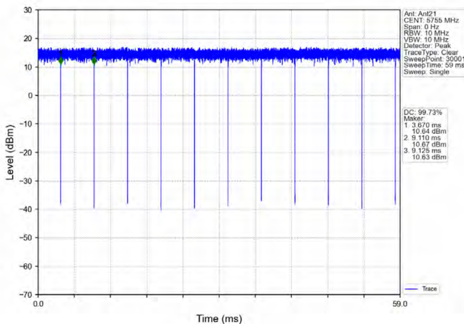
802.11ax(HE40) LCH 5755MHz RU484 Left Ant21 NTNV
