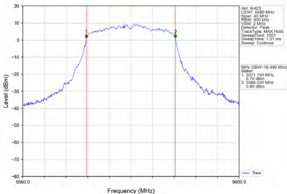
802.11a MCH_5580MHz_Ant23_NTNV
