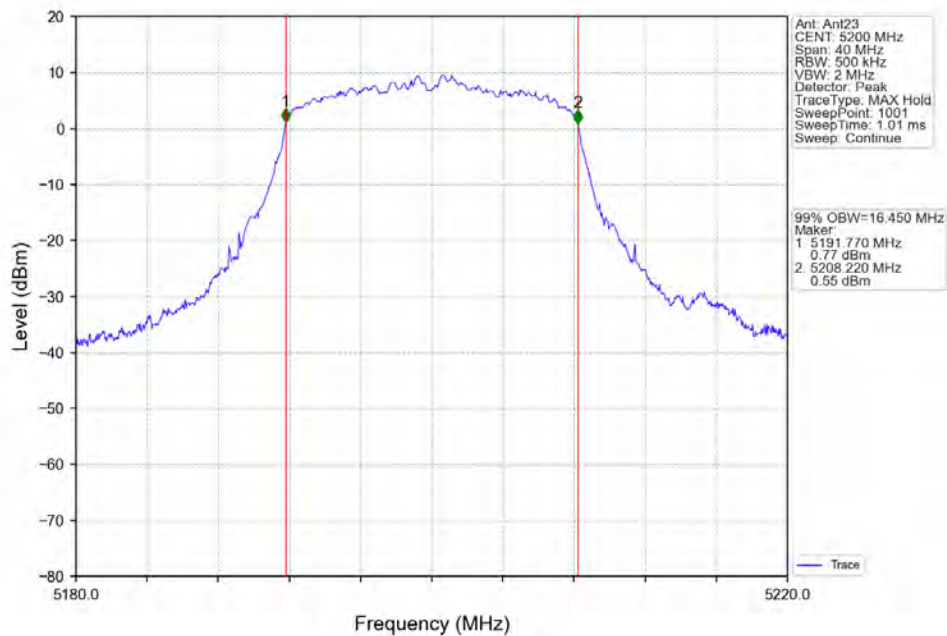
802.11a MCH_5200MHz_Ant23_NTNV
