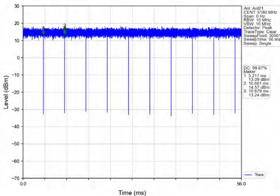
802.11ax(HE20)_LCH_5180MHz_RU242_Left Ant21_NTNV
