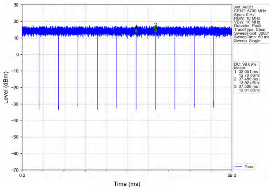
802.11ax(HE20) HCH 5700MHz RU242 Left Ant21 NTN
