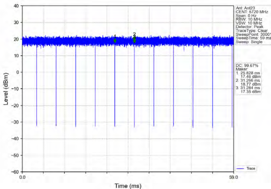
802.11ax(HE20) HCH 5720MHz RU242 Left Ant23 NTNV
