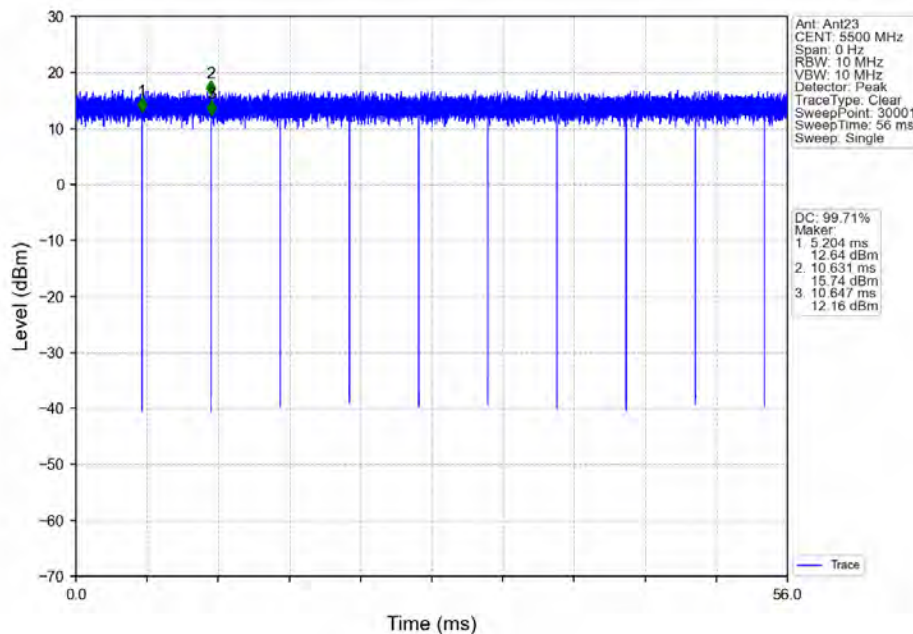
802.11n(HT20) LCH_5500MHz_Ant23_NTNV
