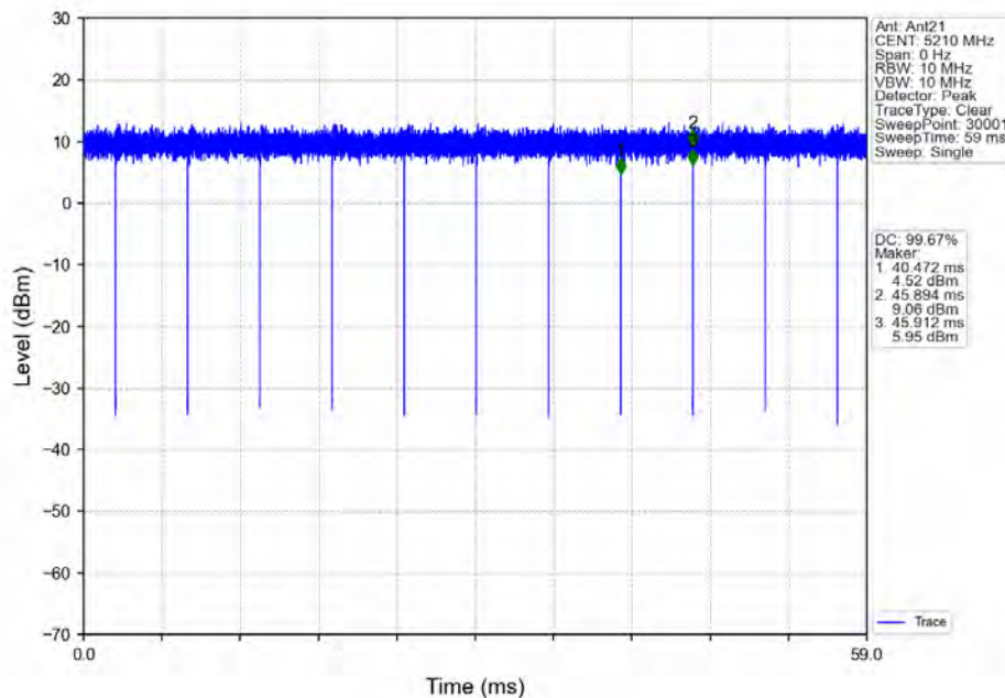
802.11ac(VHT80)_MCH_5210MHz_Ant21_NTNV
