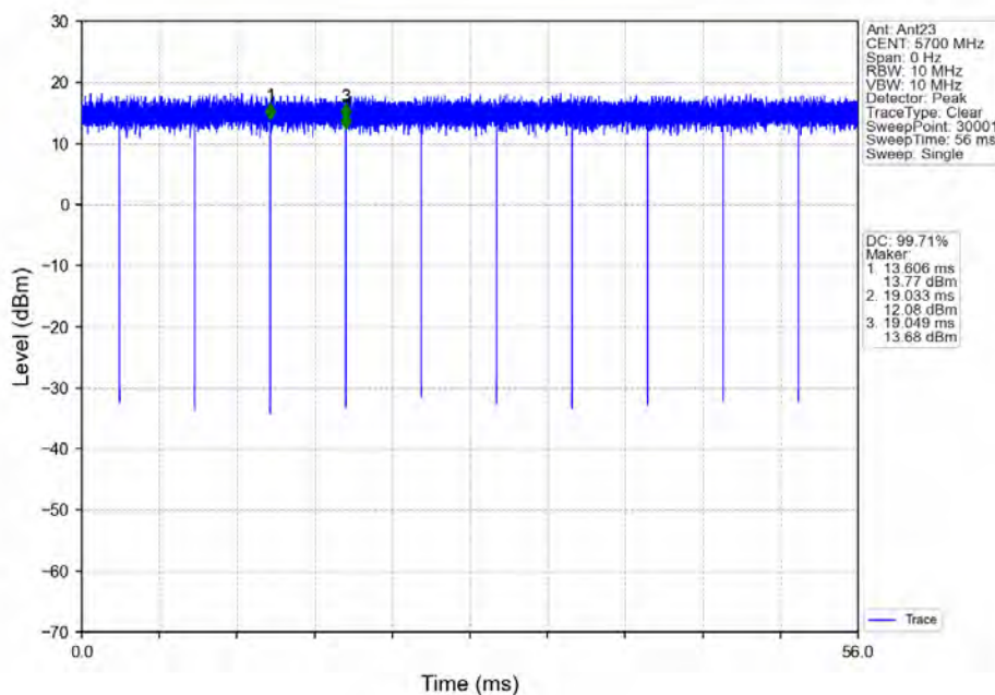
802.11n(HT20) HCH 5700MHz Ant23 NTN
