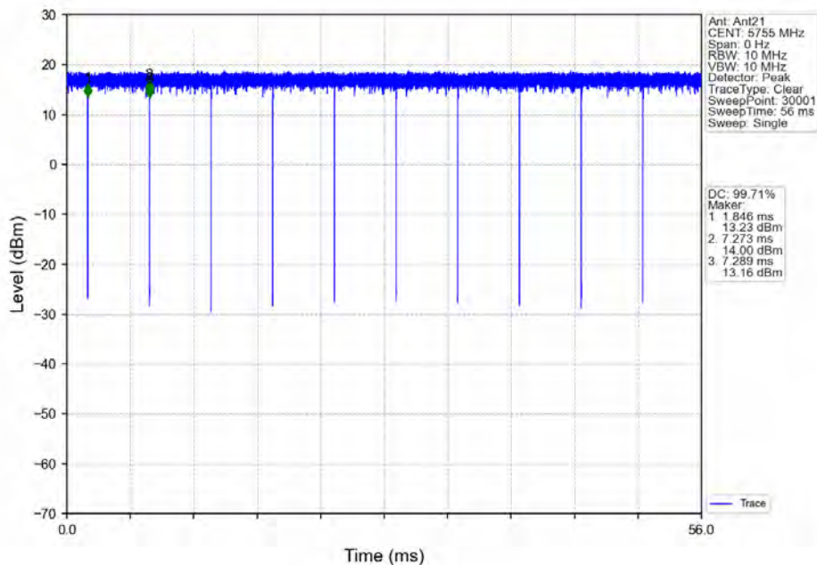
802.11n(HT40) LCH 5755MHz Ant21 NTN
