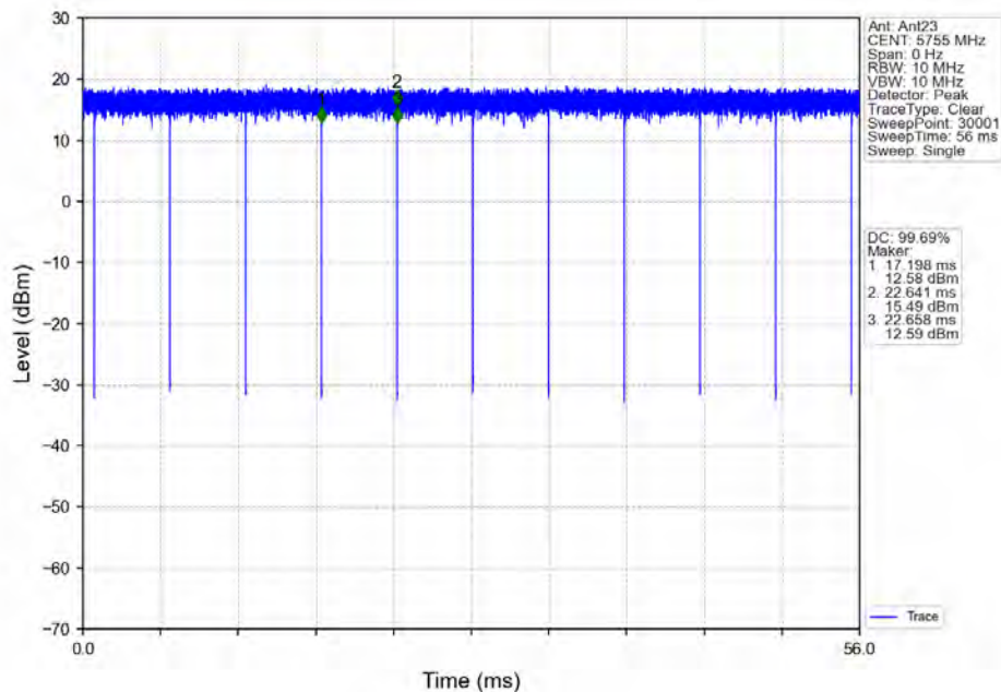
802.11ax(HE40) LCH 5755MHz RU484 Left Ant23 NTN
