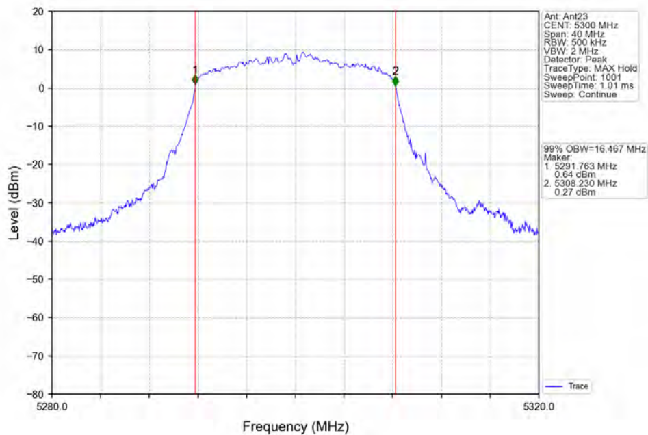
802.11a MCH_5300MHz_Ant23_NTNV
