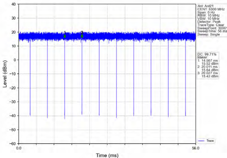
802.11ax(HE20) MCH 5300MHz RU242 Left Ant21 NTN
