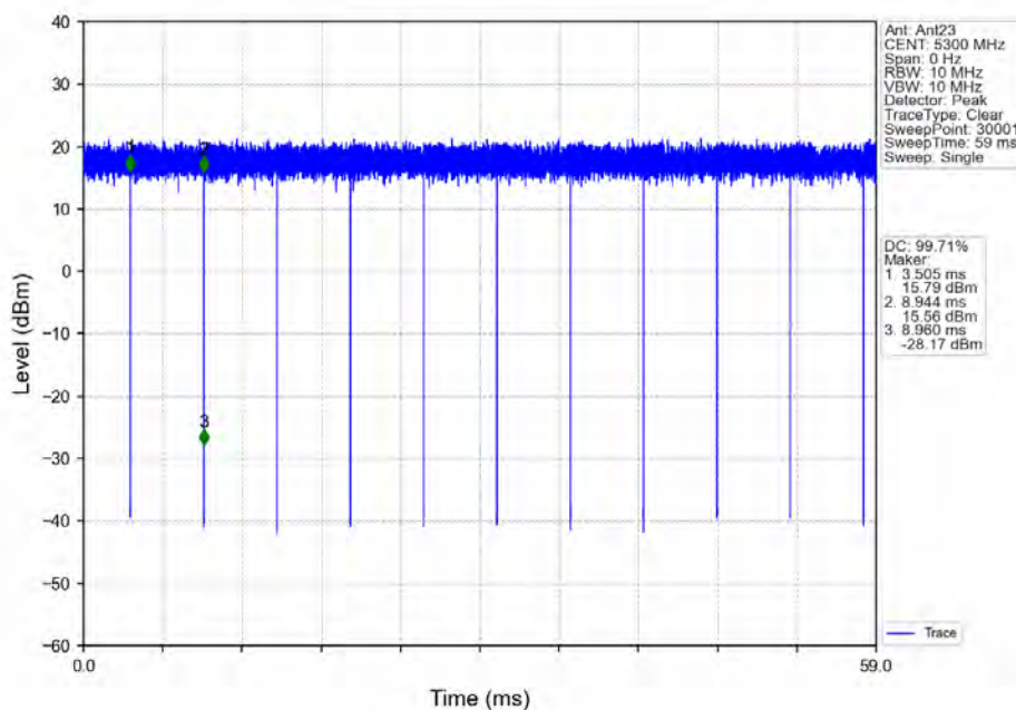
802.11ax(HE20) MCH 5300MHz RU242 Left Ant23 NTVN
