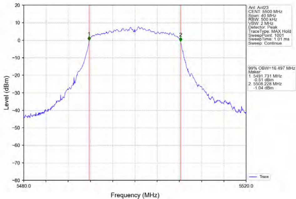
802.11a_LCH_5500MHz_Ant23_NTNV
