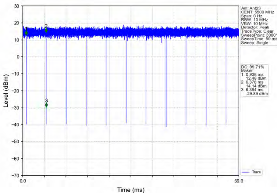
802.11ax(HE20) LCH 5500MHz RU242 Left Ant23 NTNV
