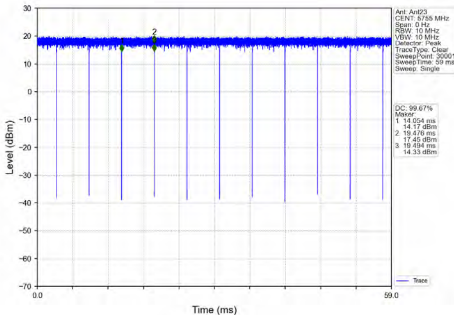
802.11n(HT40) LCH_5755MHz_Ant23_NTNV
