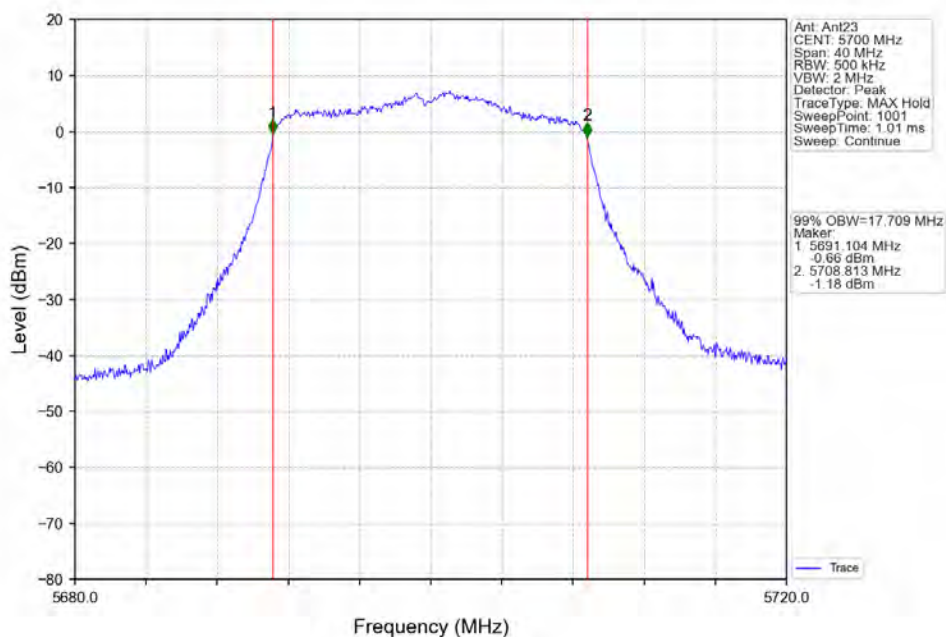
802.11n(HT20) HCH 5700MHz Ant23 NTNV
