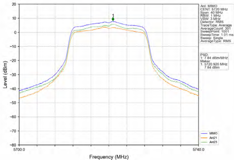
802.11a_HCH_5720MHz_MIMO_NTNV
