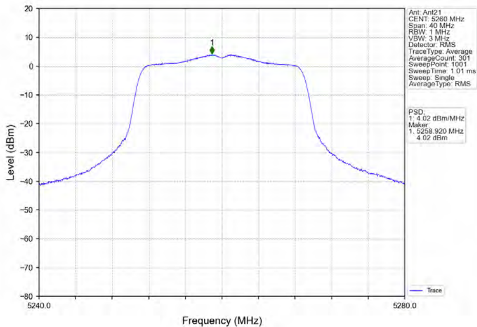
802.11n(HT20) LCH_5260MHz Ant21 NTN
