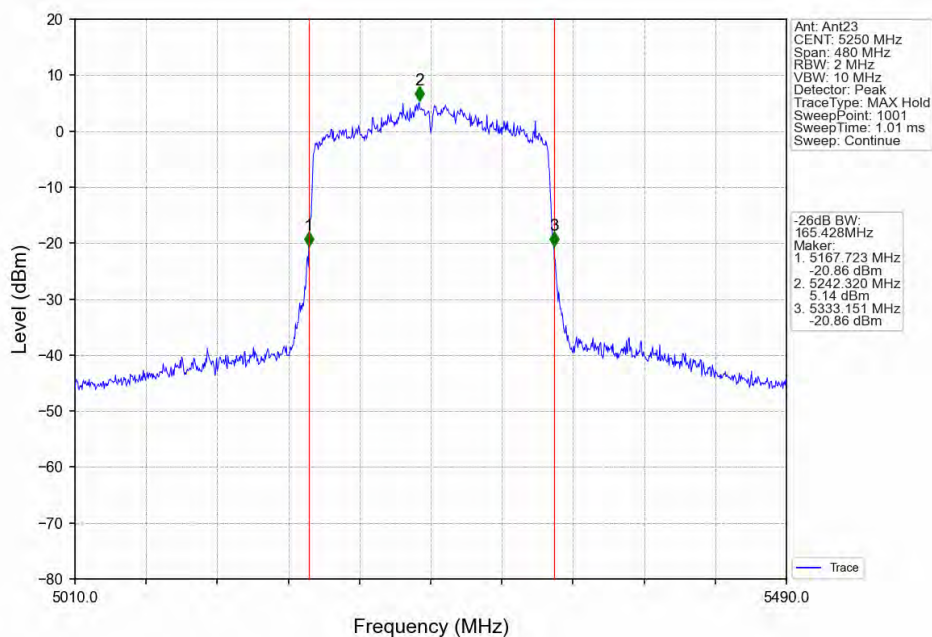
802.11ax(HE160) MCH_5250MHz_2xRU996 Left_Ant23_NTNV
