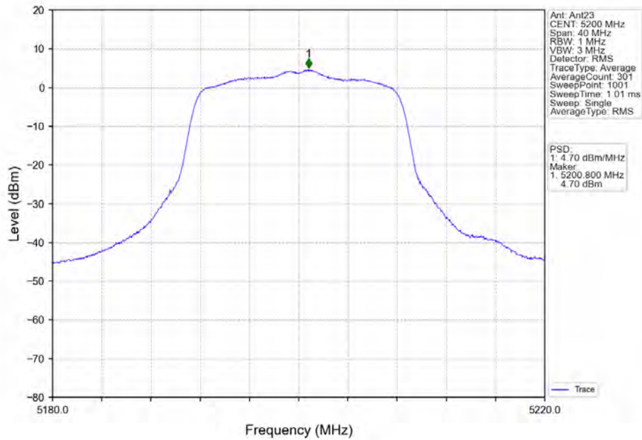
802.11a_MCH_5200MHz_MIMO_NTNV
