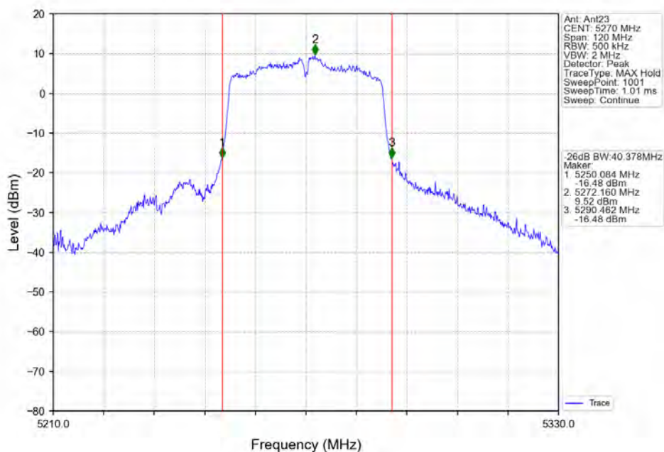
802.11n(HT40) LCH_5270MHz_Ant23_NTNV
