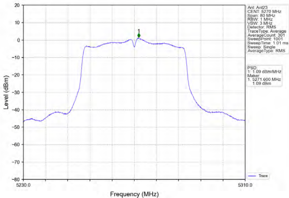
802.11n(HT40) LCH_5270MHz_Ant23_NTNV
