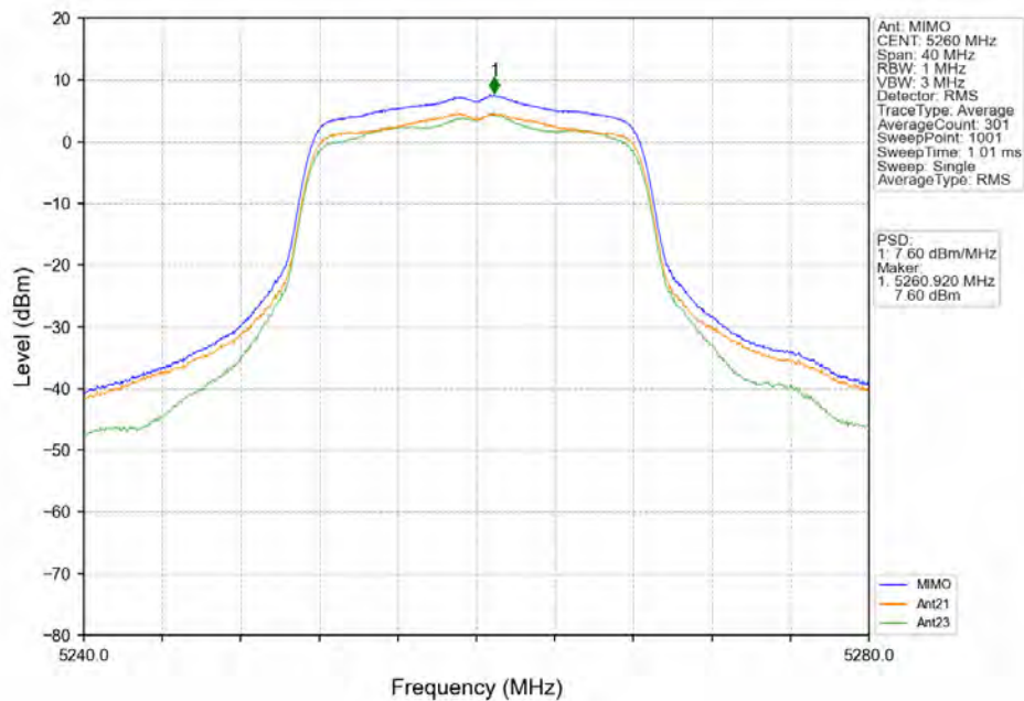
802.11a_LCH_5260MHz_MIMO_NTNV
