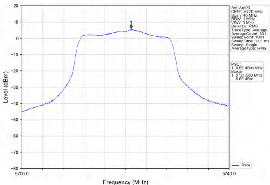
802.11n(HT20) HCH 5720MHz MIMO NTN
