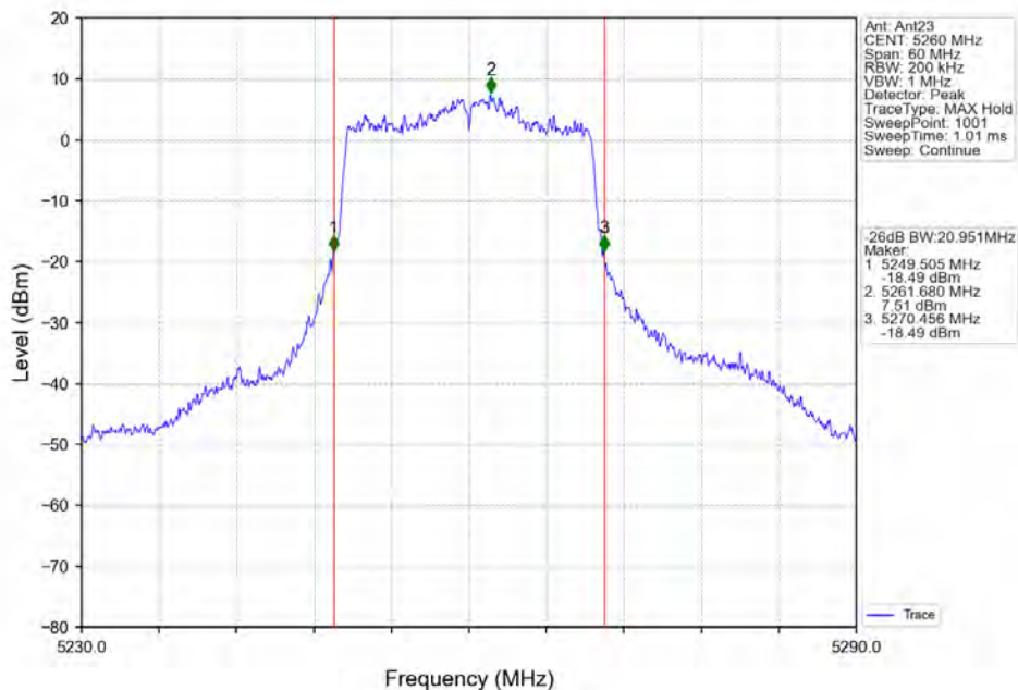
802.11ax(HE20) LCH_5260MHz_RU242_Left_Ant23_NTNV
