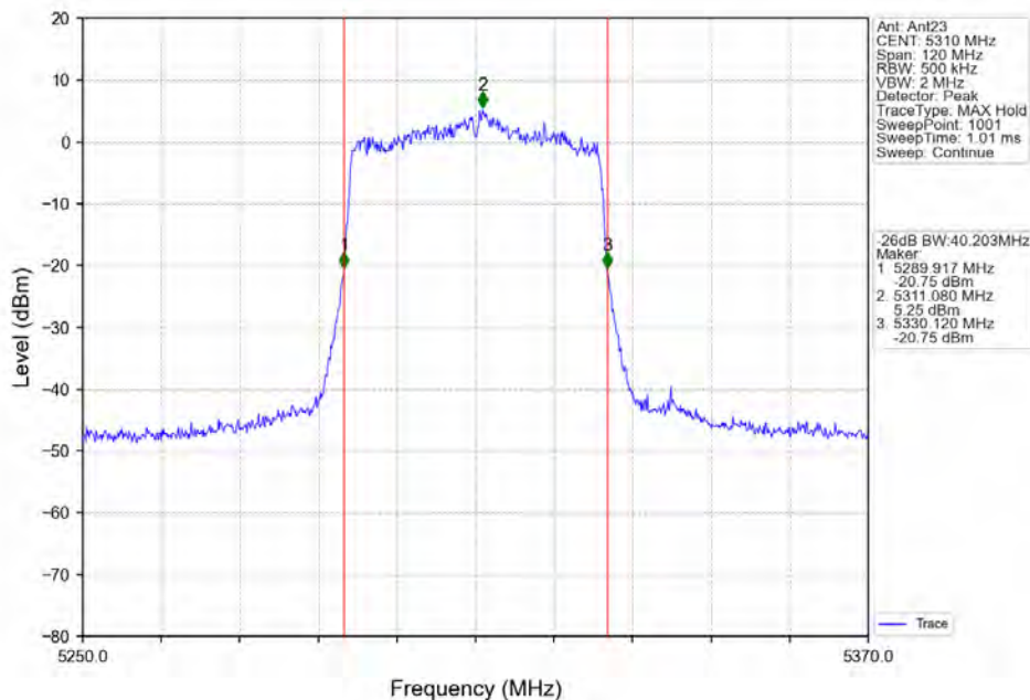
802.11ax(HE40) HCH 5310MHz RU484 Left Ant23 NTNV
