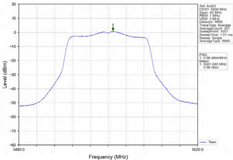
802.11n(HT20) LCH_5500MHz_Ant23_NTNV
