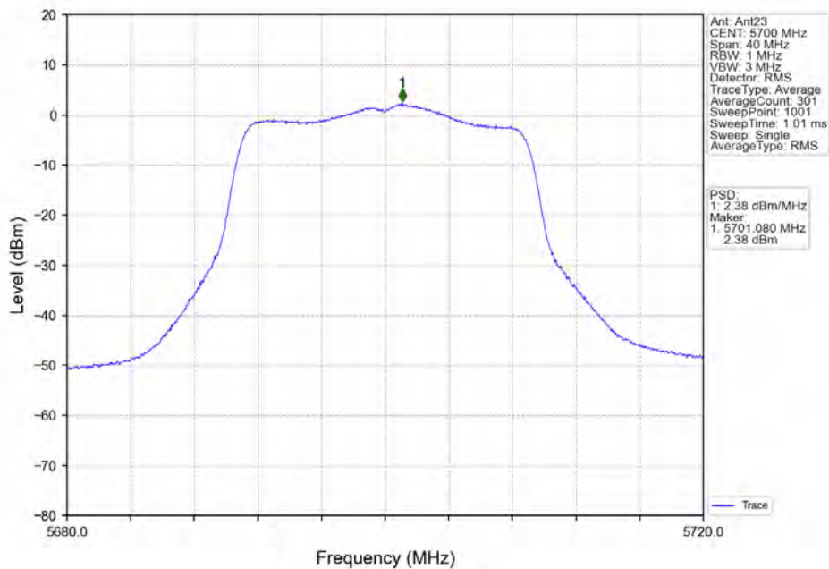
802.11n(HT20) HCH 5700MHz Ant23 NTNV
