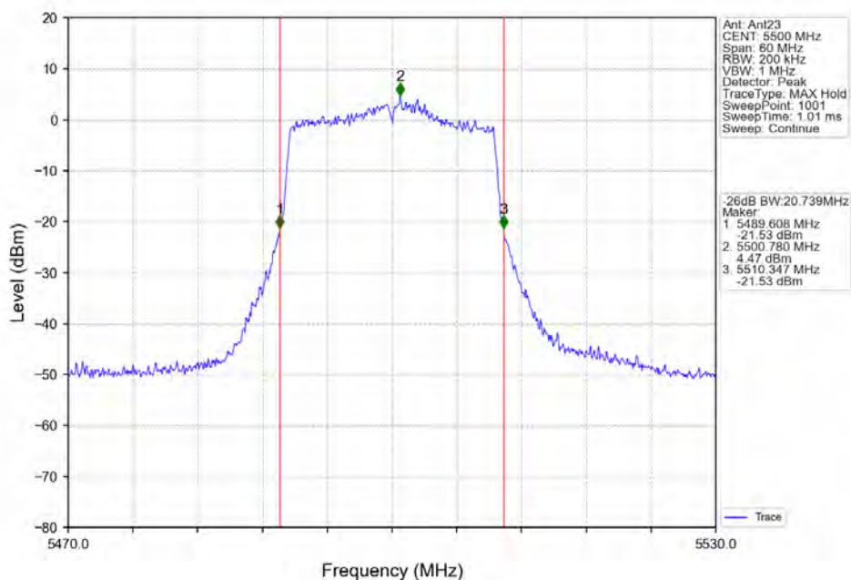
802.11ax(HE20) LCH_5500MHz_RU242_Left_Ant23_NTNV
