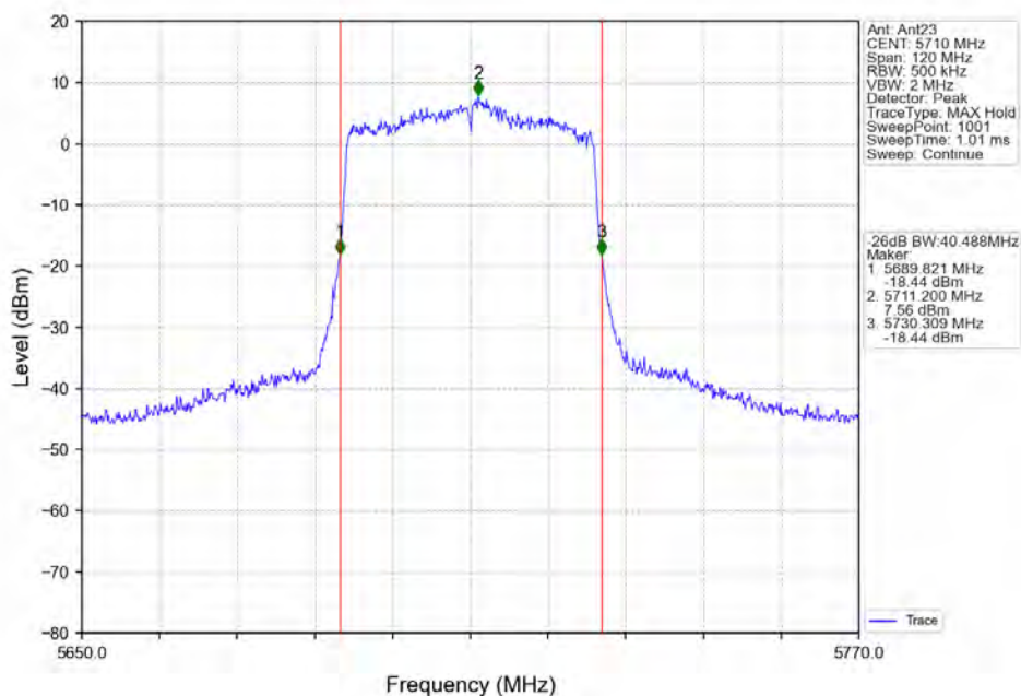
802.11ax(HE40) HCH 5710MHz RU484 Left Ant23 NTN
