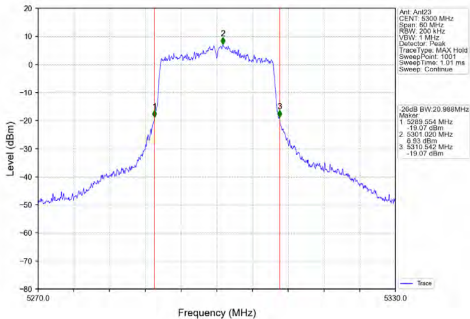
802.11ax(HE20) MCH 5300MHz RU242 Left Ant23 NTVN
