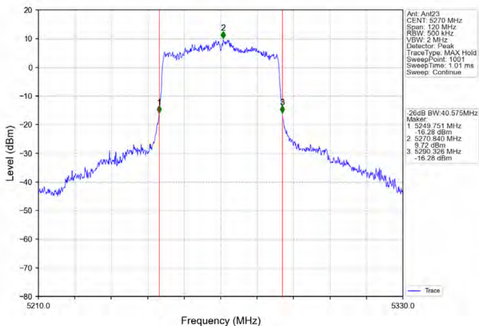
802.11ax(HE40) LCH_5270MHz RU484 Left Ant23_NTNV
