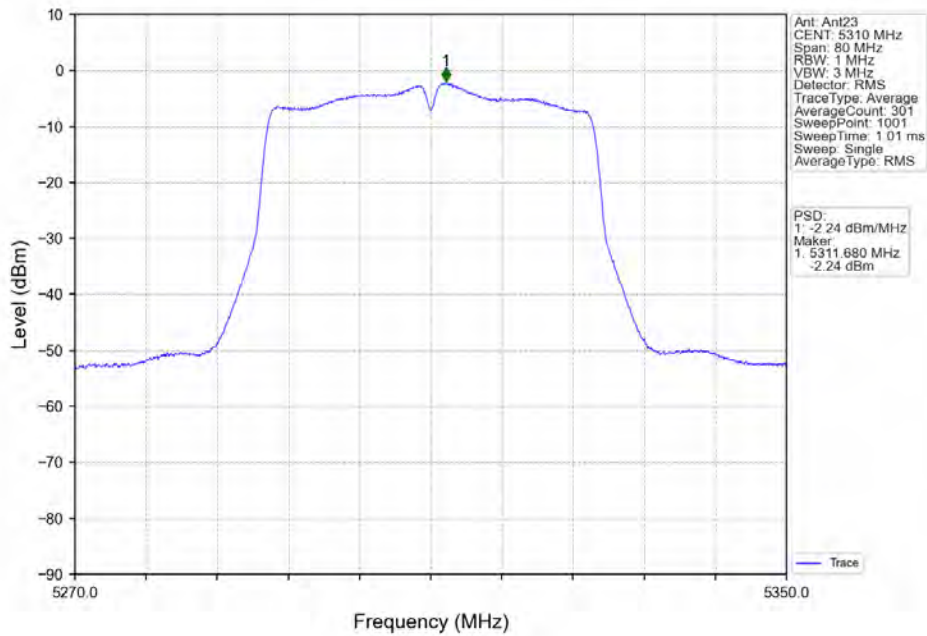
802.11n(HT40) HCH_5310MHz_MIMO_NTNV
