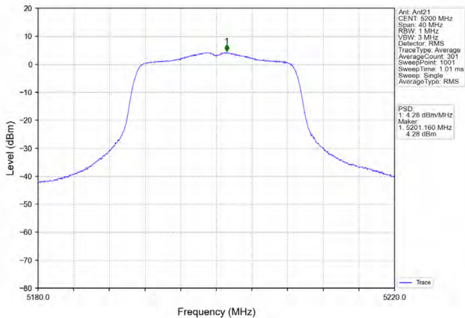
802.11n(HT20) MCH_5200MHz_Ant21_NTNV
