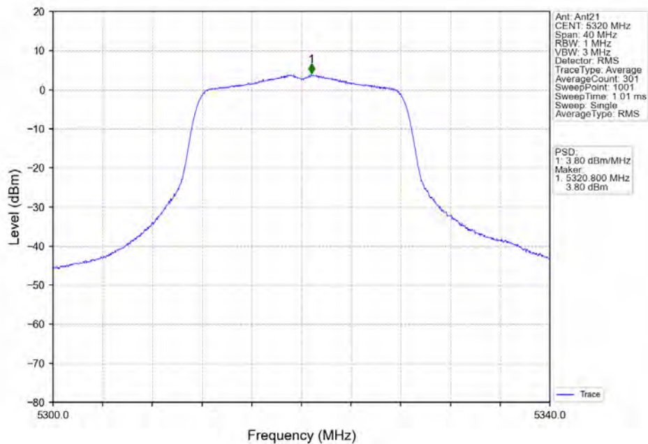
802.11a HCH 5320MHz Ant21 NTN
