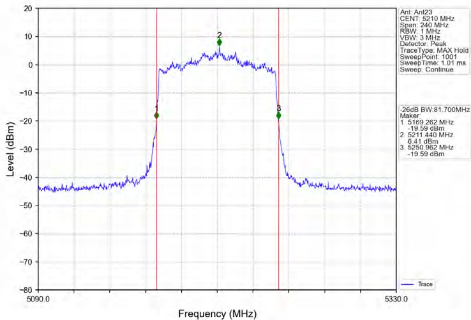
802.11ax(HE80) MCH 5210MHz RU996 Left Ant23 NTVN
