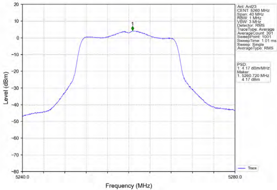
802.11n(HT20) LCH_5260MHz_MIMO_NTNV
