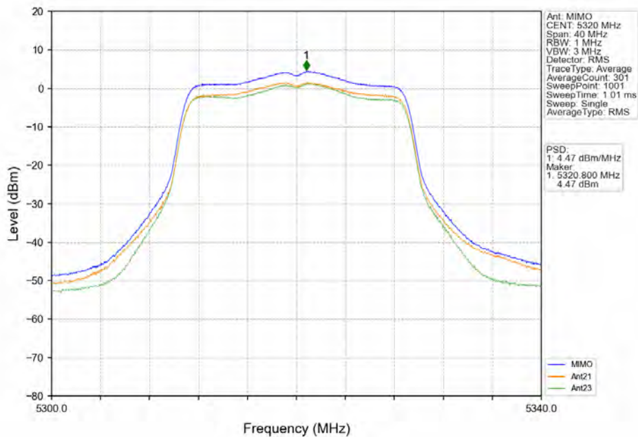
802.11n(HT20) HCH 5320MHz MIMO NTN
