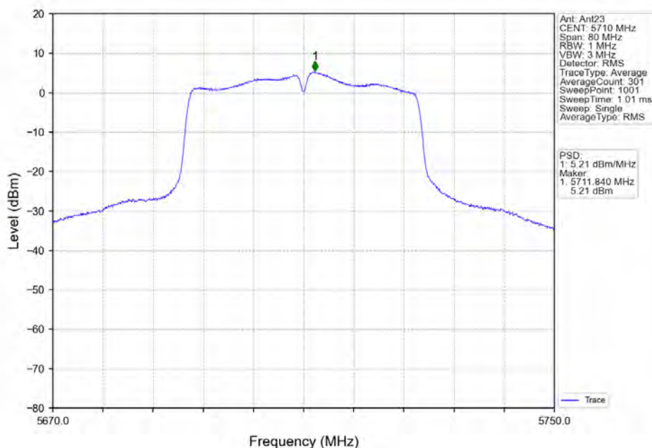
802.11n(HT40) HCH 5710MHz MIMO NTNV
