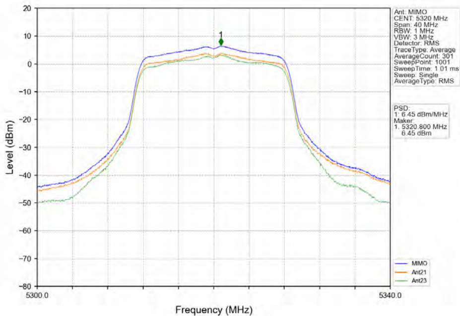
802.11a_HCH_5320MHz_MIMO_NTNV
