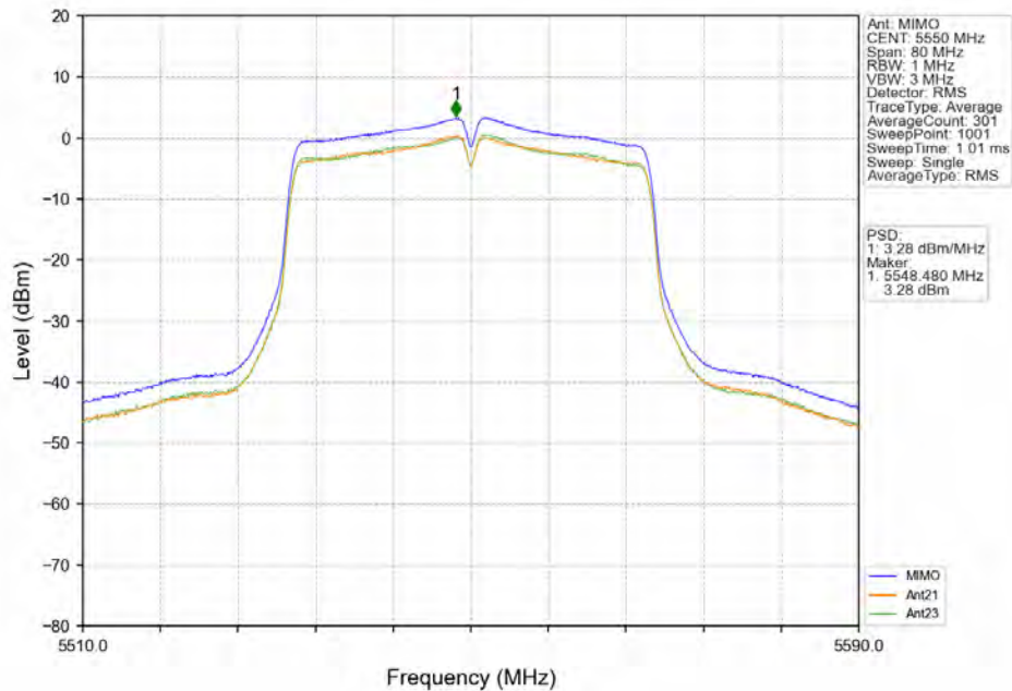
802.11n(HT40)_MCH_5550MHz_MIMO_NTNV
