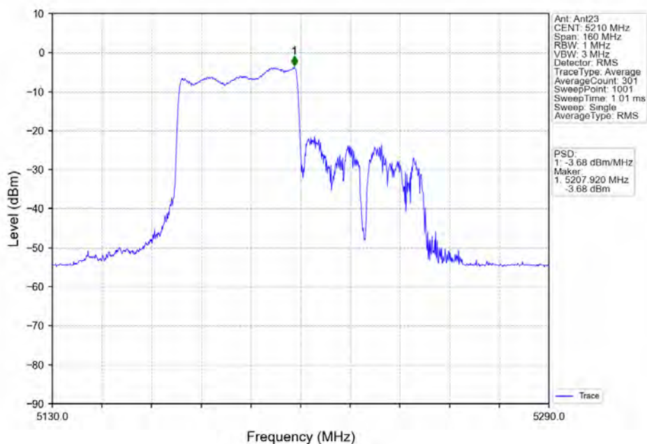
802.11ax(HE80) MCH 5210MHz RU484 Left Ant23 NTVN
