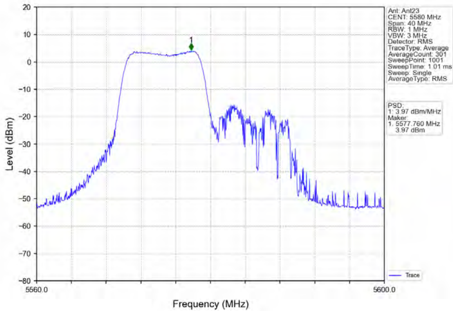
802.11ax(HE20) MCH 5580MHz RU106 Left MIMO NTN
