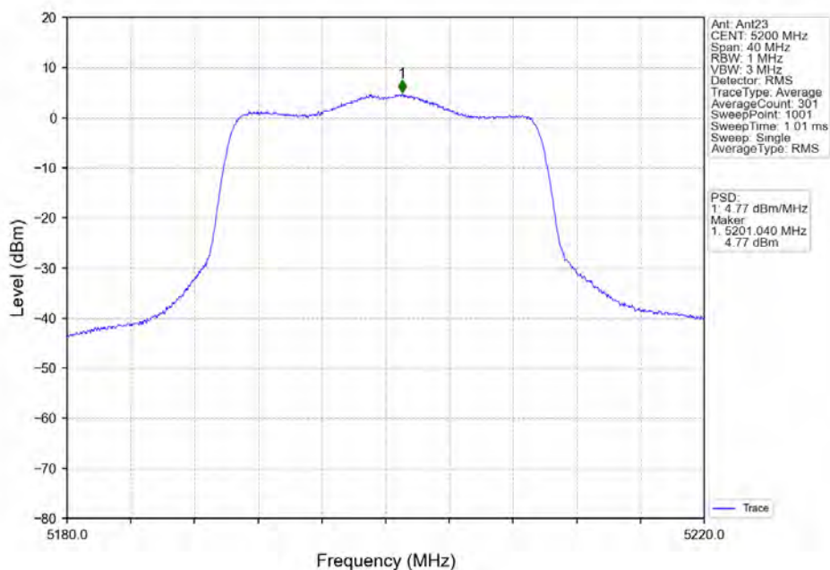
802.11ax(HE20) MCH 5200MHz RU242 Left Ant23 NTVN
