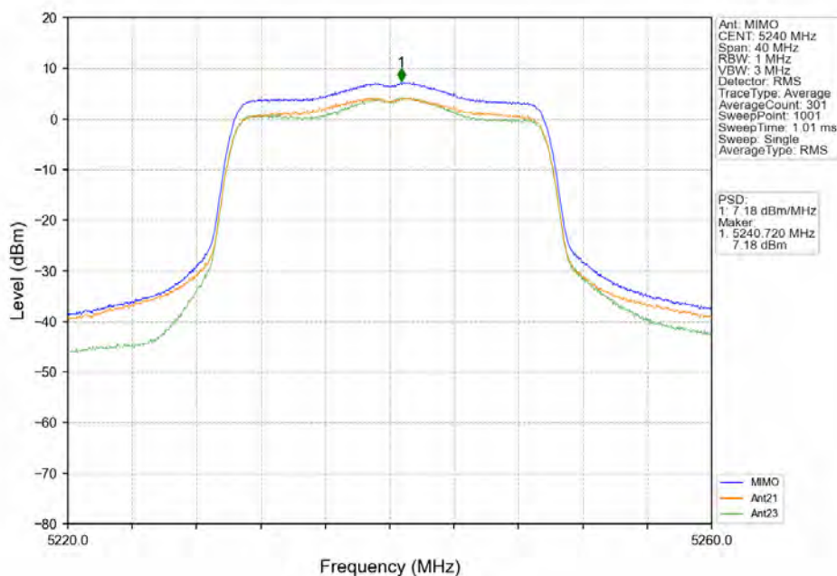
802.11ax(HE20) HCH 5240MHz RU242 Left MIMO NTNV
