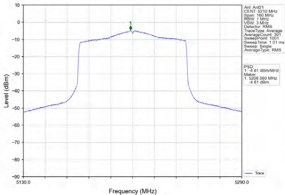
802.11ax(HE80) MCH 5210MHz RU996 Left Ant21 NTVN
