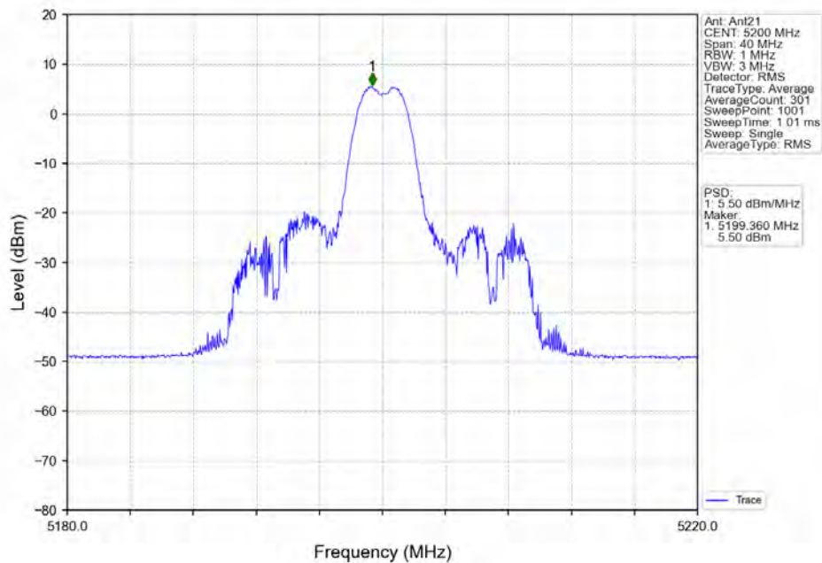
802.11ax(HE20) MCH 5200MHz RU26 Mid Ant21 NTNV
