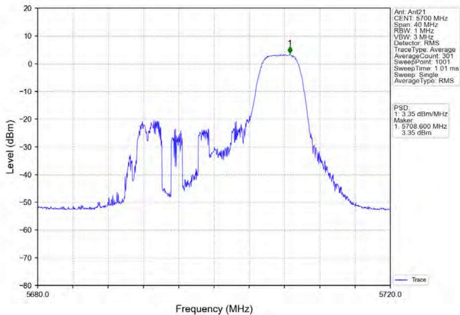
802.11ax(HE20) HCH_5700MHz RU52_Right Ant21 NTN
