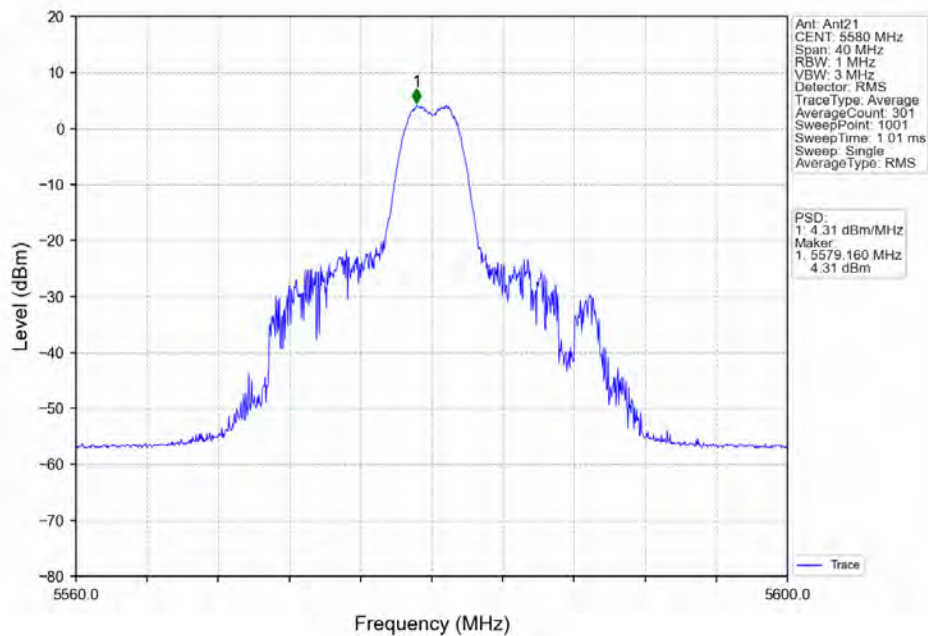
802.11ax(HE20) MCH 5580MHz RU26 Mid Ant21 NTNV
