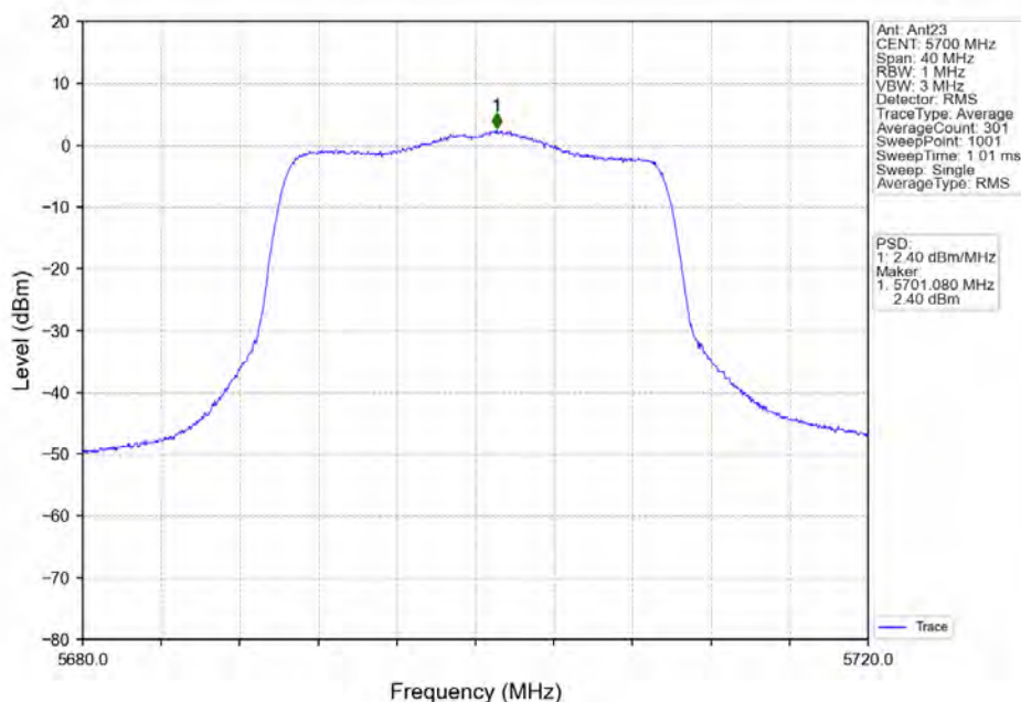
802.11ax(HE20) HCH 5700MHz RU242 Left MIMO NTVN
