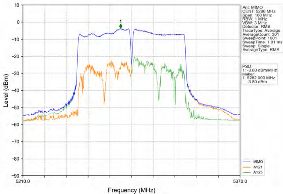
802.11ax(HE80) MCH 5290MHz RU484 Right MIMO NTN
