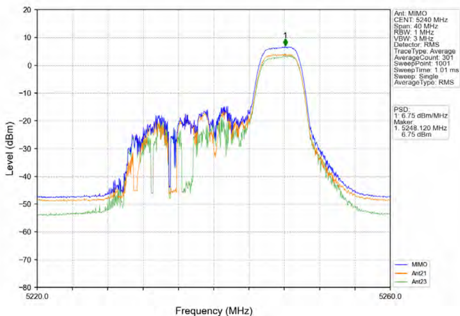
802.11ax(HE20) HCH 5240MHz RU52 Right MIMO NTNV
