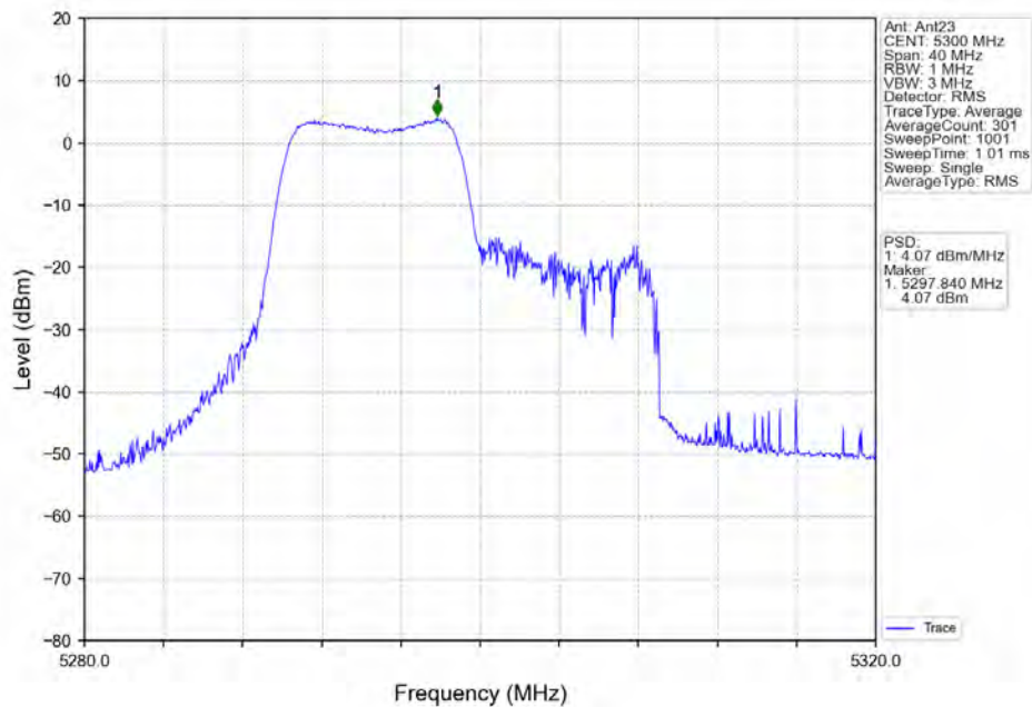
802.11ax(HE20) MCH 5300MHz RU106 Left Ant23 NTVN
