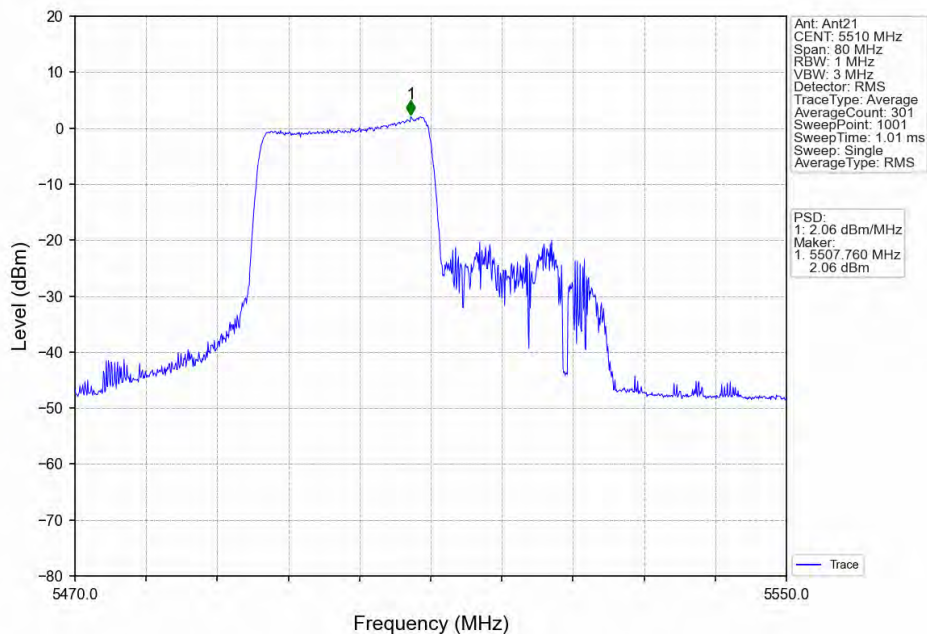
802.11ax(HE40) LCH 5510MHz RU242 Left Ant21 NTN
