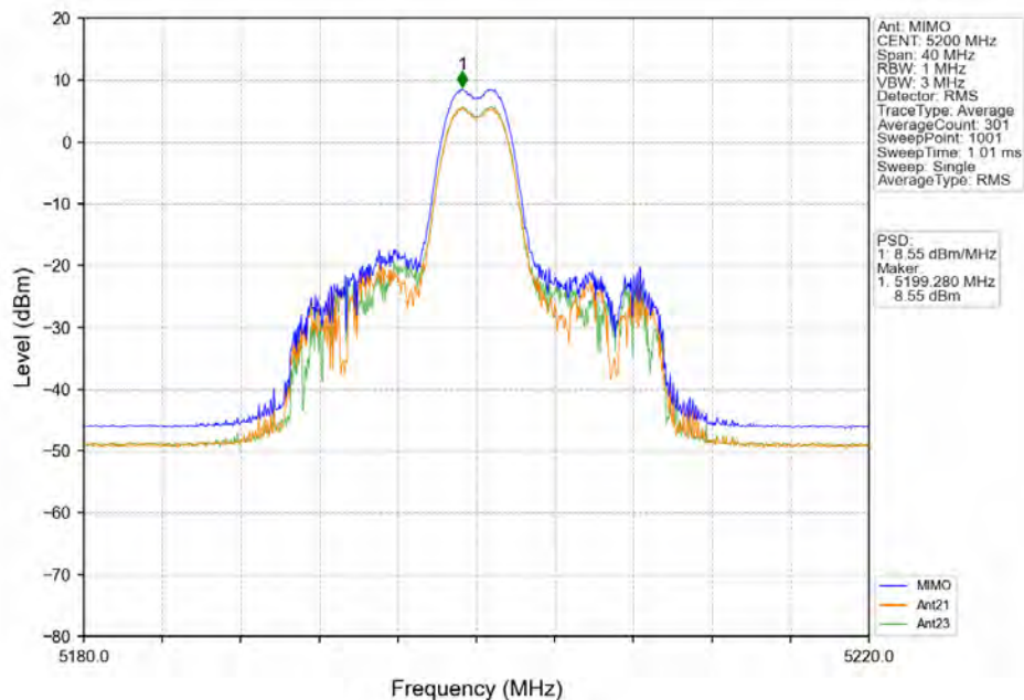
802.11ax(HE20) MCH 5200MHz RU26 Mid MIMO NTN
