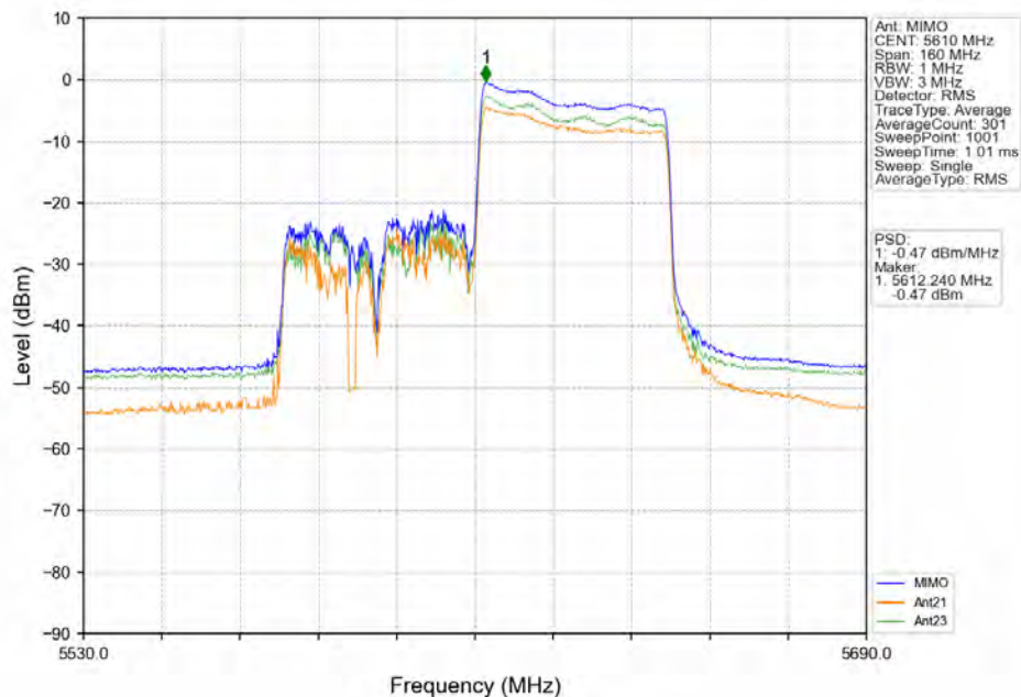
802.11ax(HE80) HCH 5610MHz RU484 Right MIMO NTN
