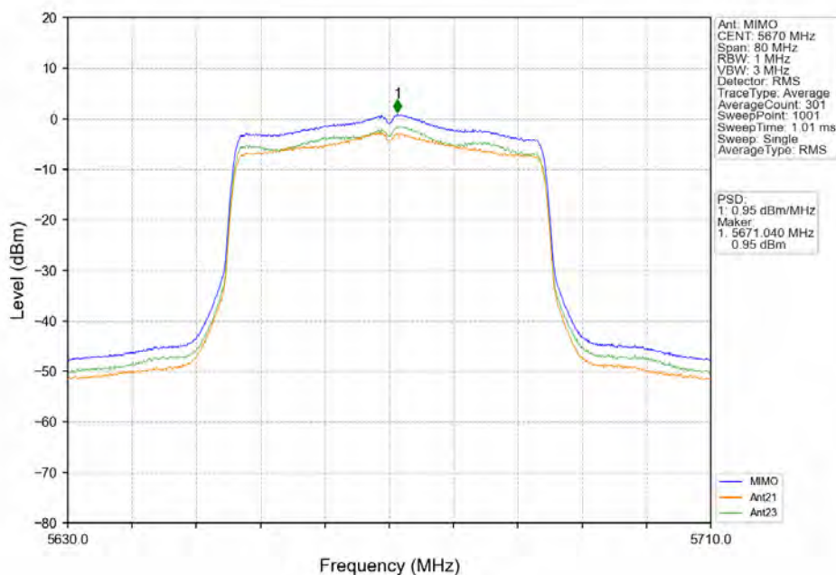
802.11ax(HE40) HCH 5670MHz RU484 Left MIMO NTNV
