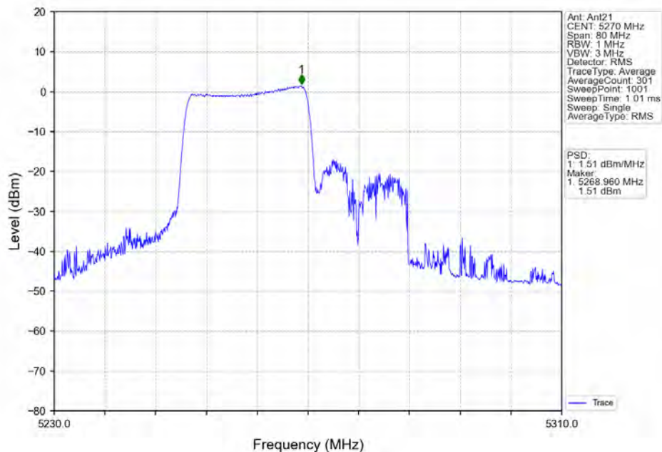
802.11ax(HE40) LCH 5270MHz RU242 Left Ant21 NTN
