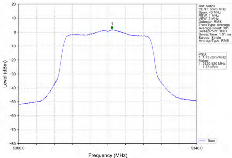
802.11ax(HE20) HCH 5320MHz RU242 Left Ant23 NTNV
