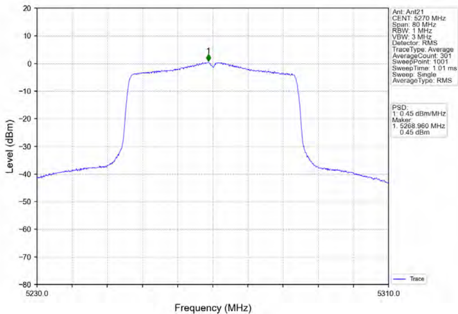
802.11ax(HE40) LCH 5270MHz RU484 Left Ant21 NTN
