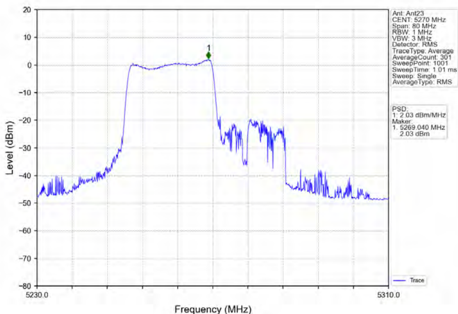
802.11ax(HE40) LCH_5270MHz RU242 Left MIMO_NTNV
