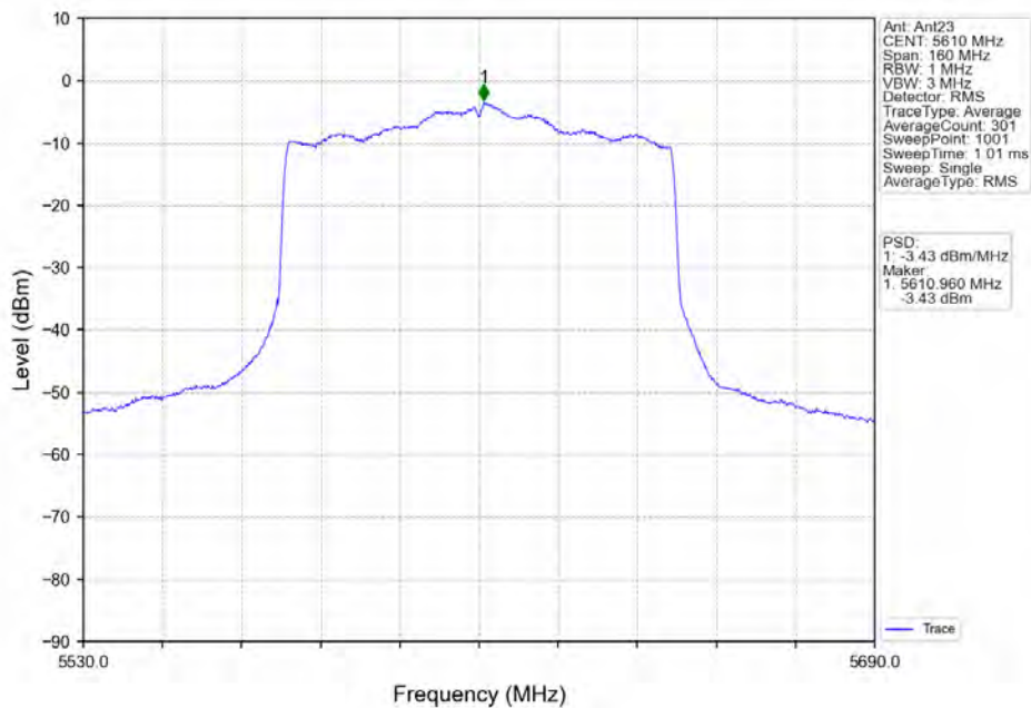
802.11ax(HE80) HCH 5610MHz RU996 Left Ant23 NTNV
