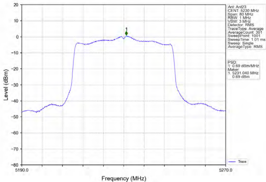
802.11ax(HE40) HCH 5230MHz RU484 Left Ant23 NTNV
