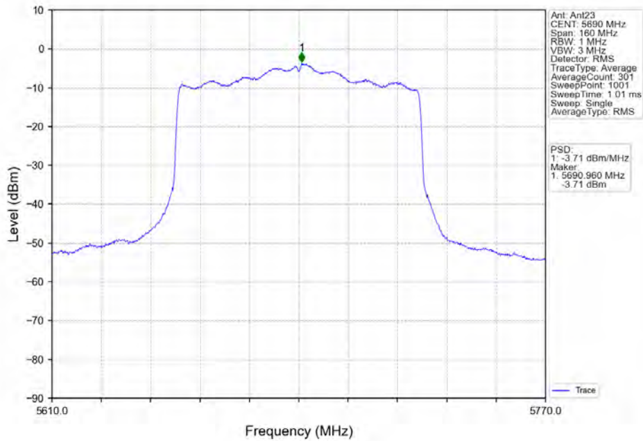
802.11ax(HE80) HCH 5690MHz RU996 Left MIMO NTVN
