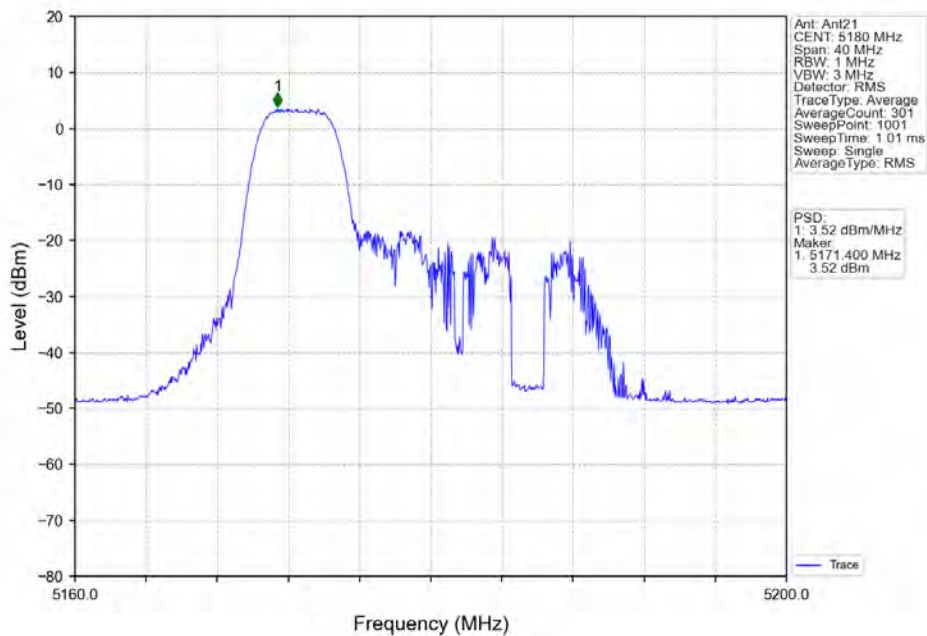
802.11ax(HE20) LCH 5180MHz RU52 Left Ant21 NTN
