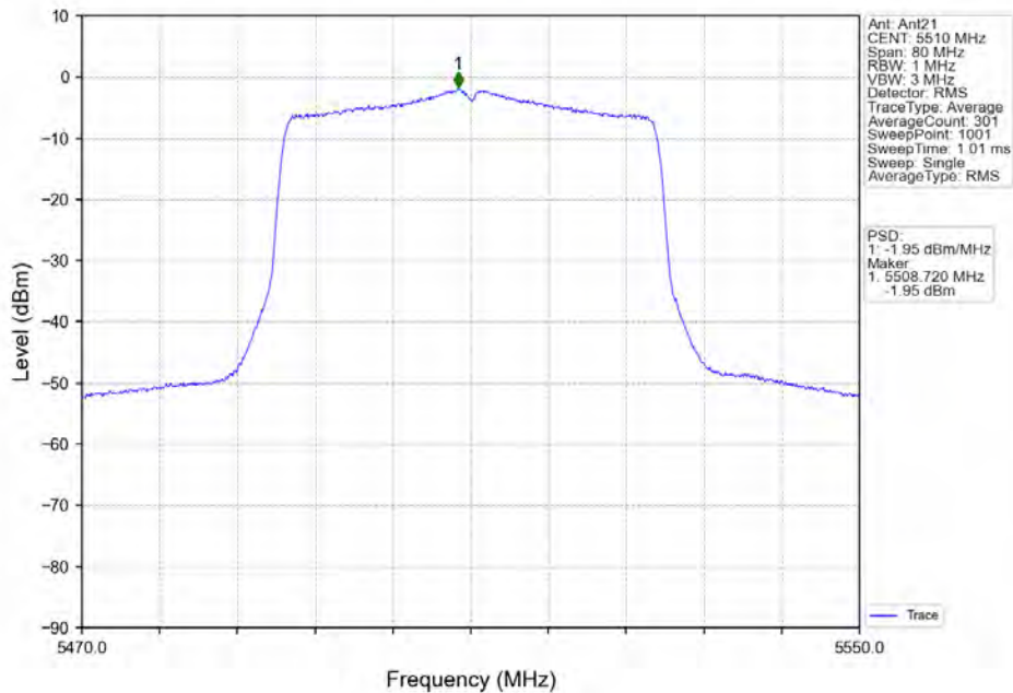
802.11ax(HE40) LCH_5510MHz RU484 Left Ant21 NTN
