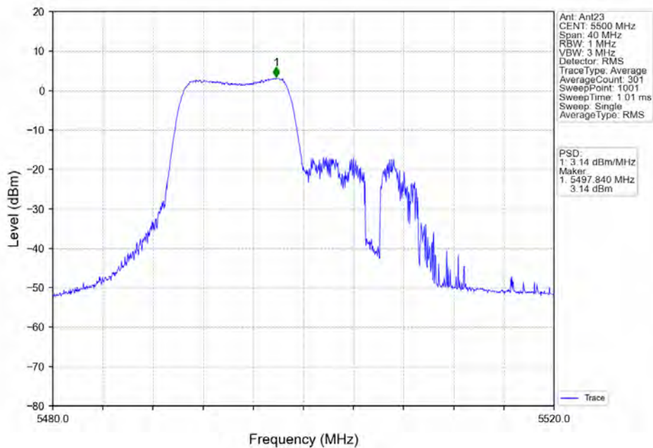
802.11ax(HE20) LCH_5500MHz_RU106_Left_Ant23_NTNV
