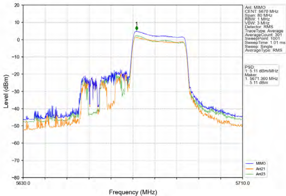
802.11ax(HE40) HCH 5670MHz RU242 Right MIMO NTN
