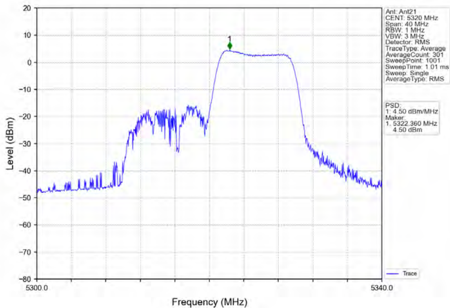
802.11ax(HE20) HCH 5320MHz RU106 Right Ant21 NTN
