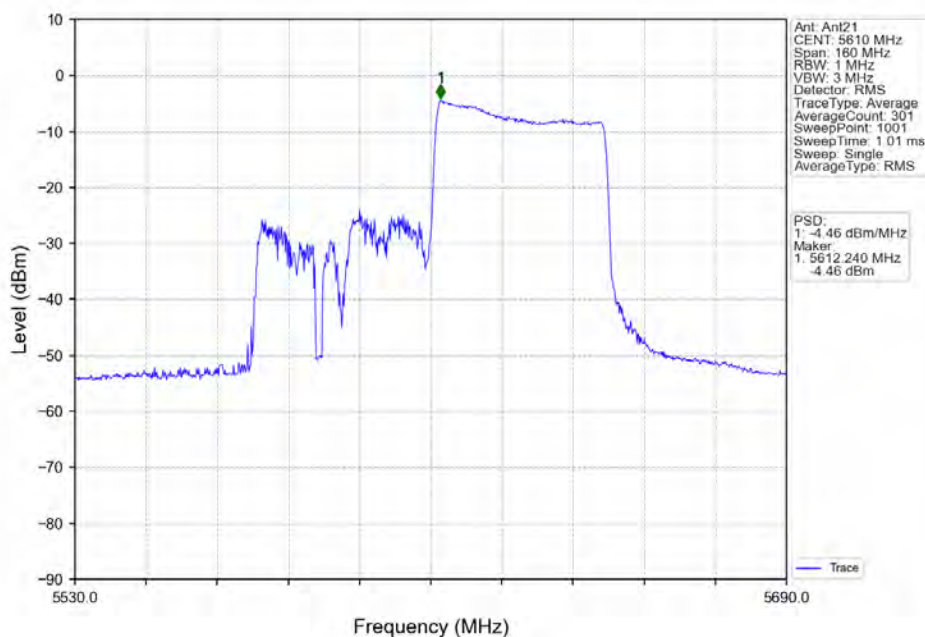
802.11ax(HE80) HCH 5610MHz RU484 Right Ant21 NTN
