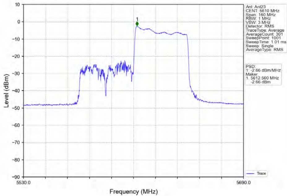
802.11ax(HE80) HCH 5610MHz RU484 Right MIMO NTN
