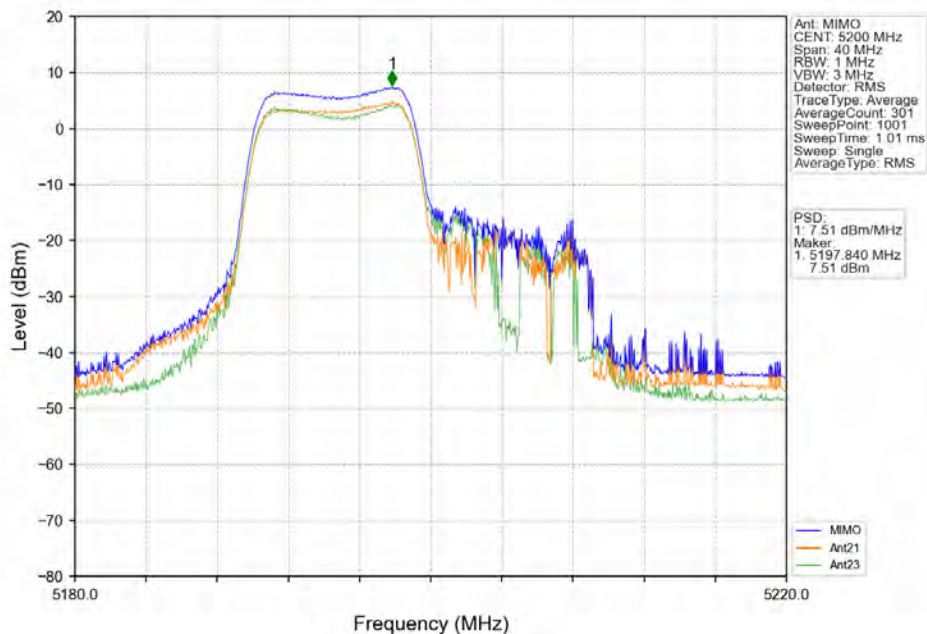
802.11ax(HE20) MCH 5200MHz RU106 Left MIMO NTNV
