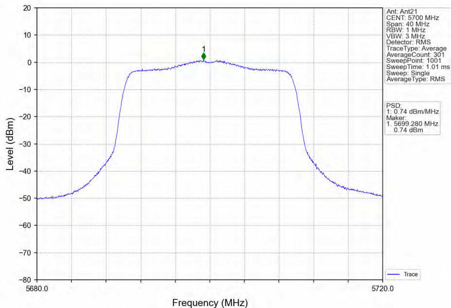
802.11ax(HE20) HCH 5700MHz RU242 Left Ant21 NTN
