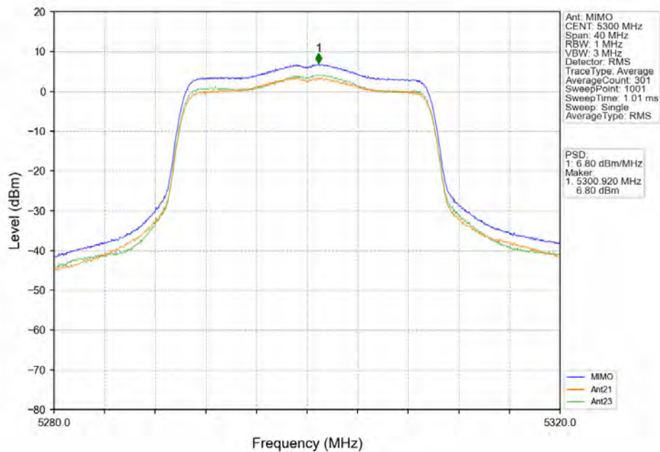
802.11ax(HE20) MCH 5300MHz RU242 Left MIMO NTNV
