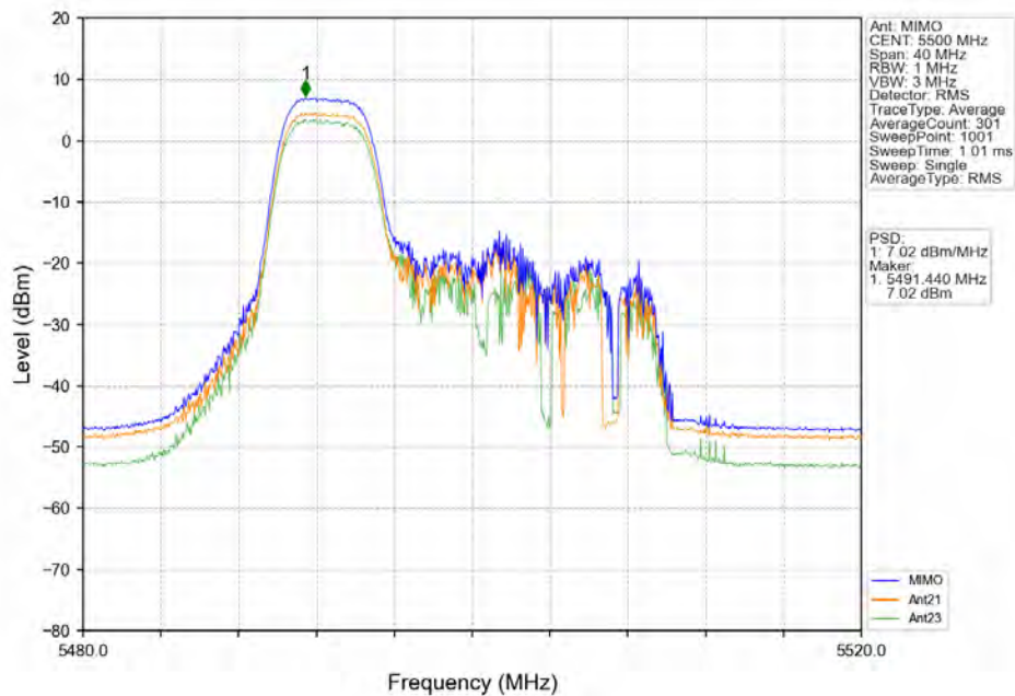
802.11ax(HE20) LCH 5500MHz RU52 Left MIMO NTNV
