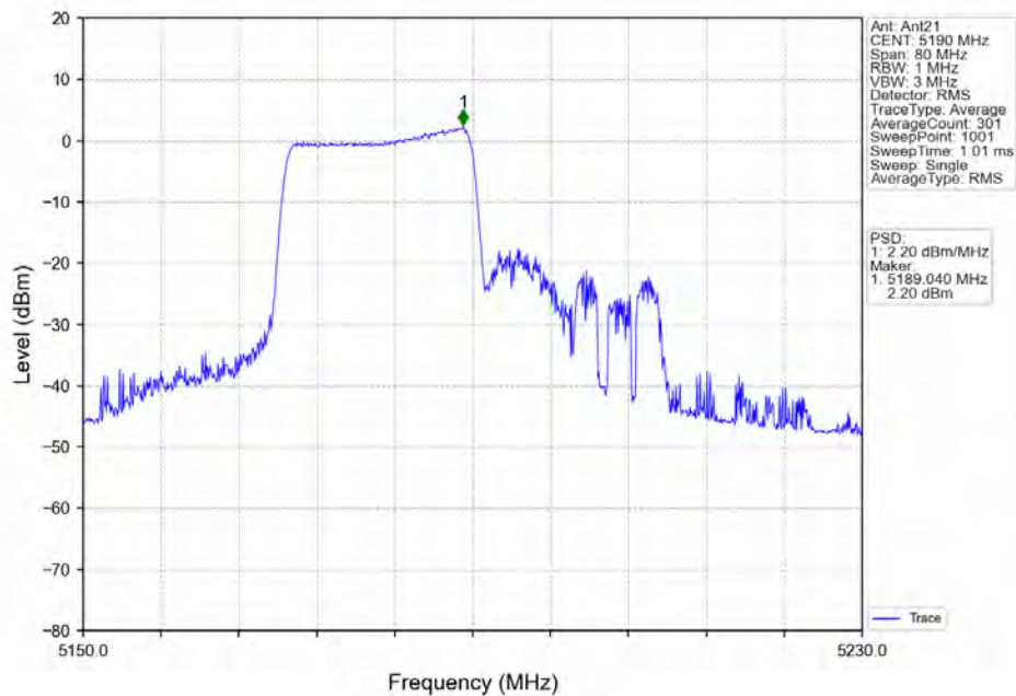
802.11ax(HE40) LCH 5190MHz RU242 Left Ant21 NTN
