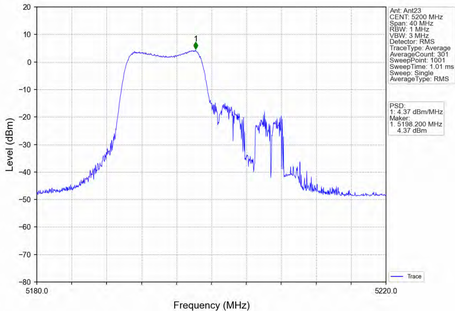
802.11ax(HE20) MCH 5200MHz RU106 Left MIMO NTNV
