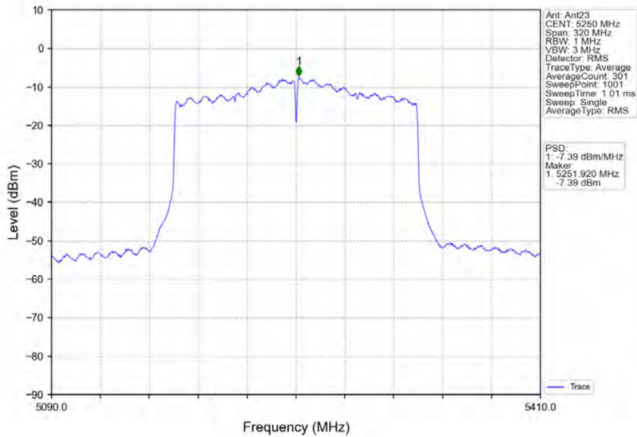
802.11ax(HE160) MCH 5250MHz 2xRU996 Left MIMO NTN
