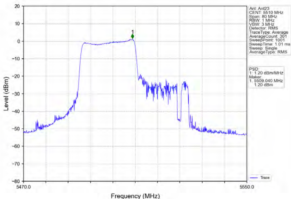
802.11ax(HE40) LCH_5510MHz_RU242_Left_MIMO_NTNV
