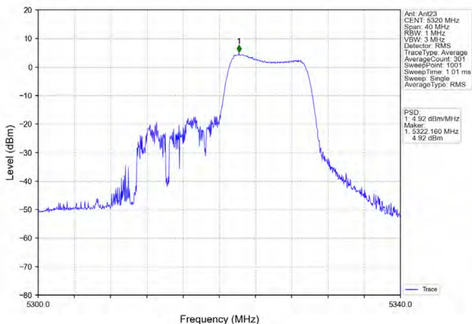
802.11ax(HE20) HCH 5320MHz RU106 Right MIMO NTN
