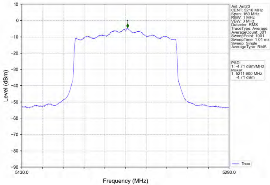
802.11ax(HE80) MCH 5210MHz RU996 Left MIMO NTNV
