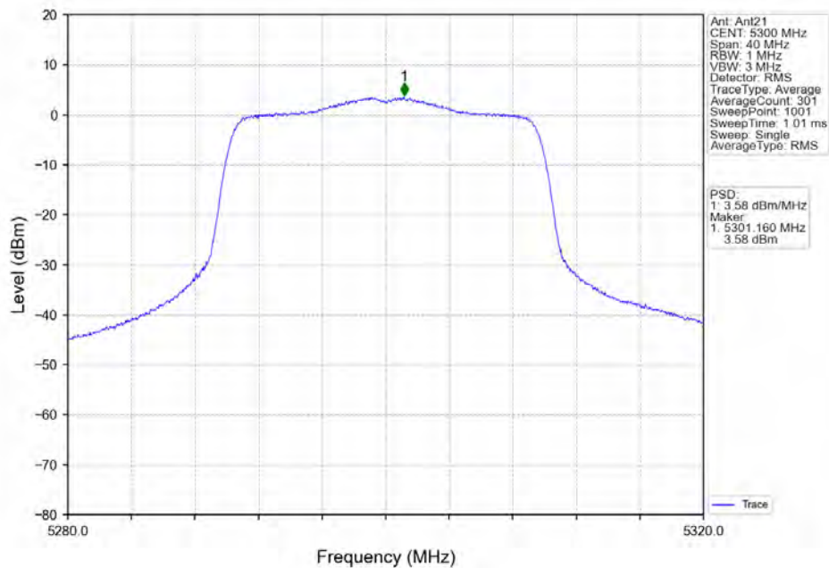
802.11ax(HE20) MCH 5300MHz RU242 Left Ant21 NTNV
