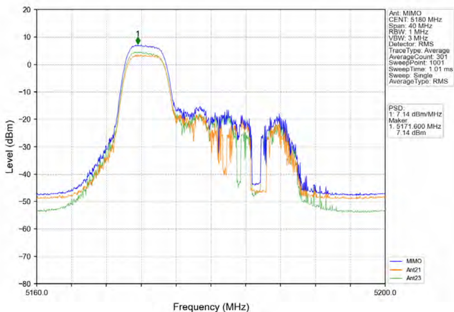
802.11ax(HE20) LCH 5180MHz RU52 Left MIMO NTNV
