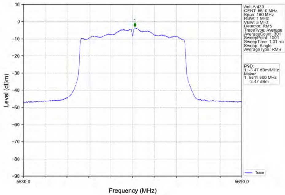
802.11ac(VHT80)_HCH_5610MHz_MIMO_NTNV
