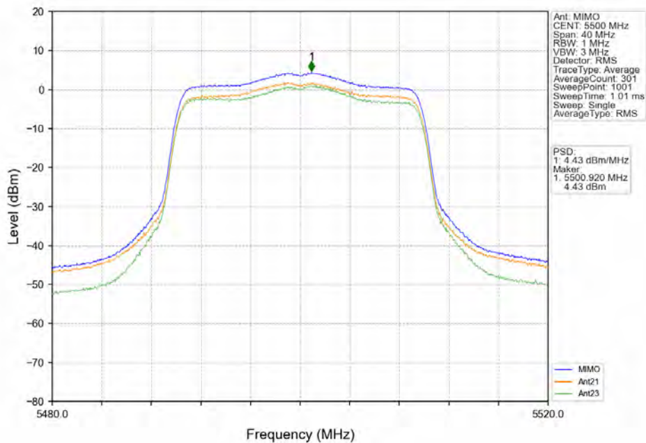
802.11ax(HE20) LCH_5500MHz_RU242_Left_MIMO_NTNV
