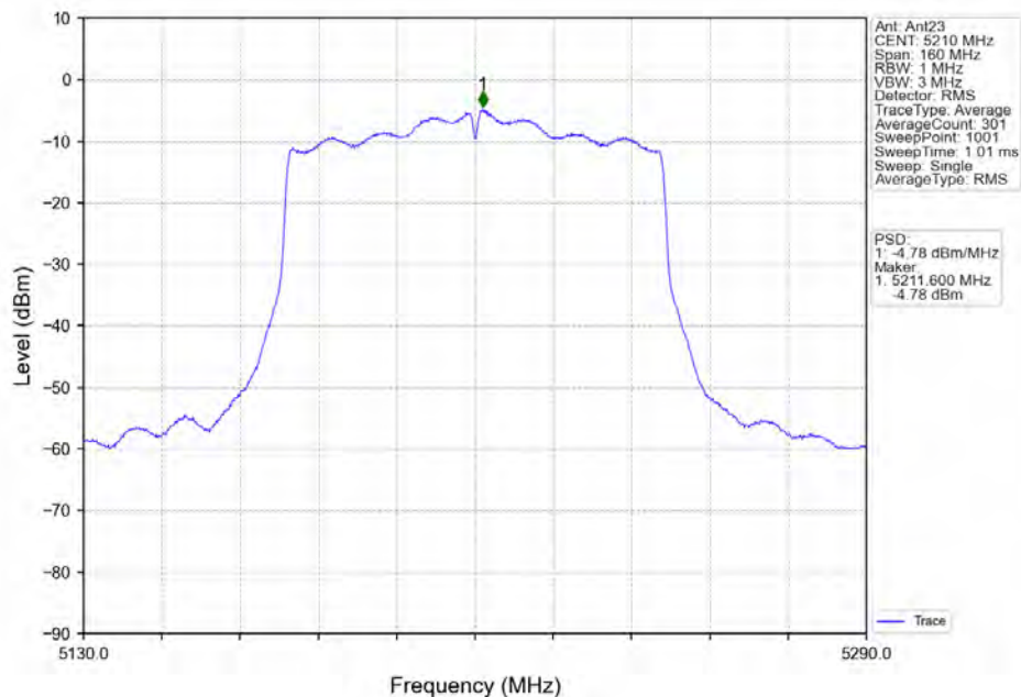
802.11ac(VHT80)_MCH_5210MHz_Ant23_NTNV
