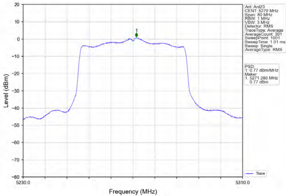
802.11ax(HE40) LCH_5270MHz RU484 Left MIMO_NTNV
