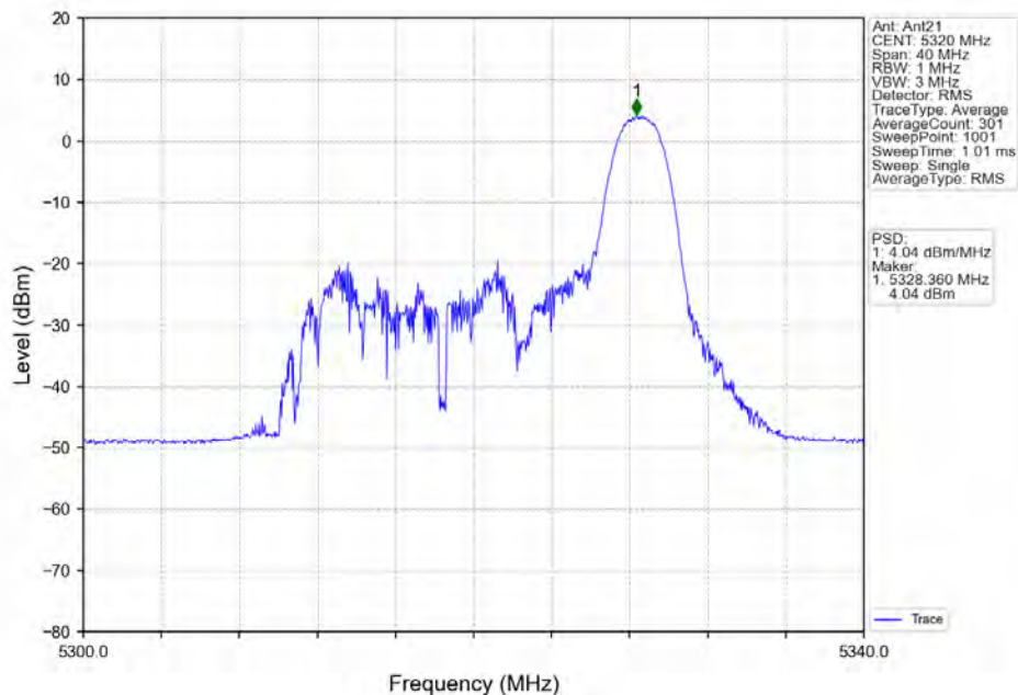
802.11ax(HE20) HCH 5320MHz RU26 Right Ant21 NTN
