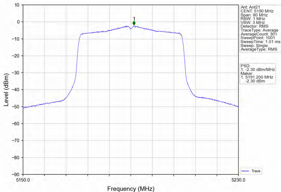
802.11ax(HE40) LCH 5190MHz RU484 Left Ant21 NTN
