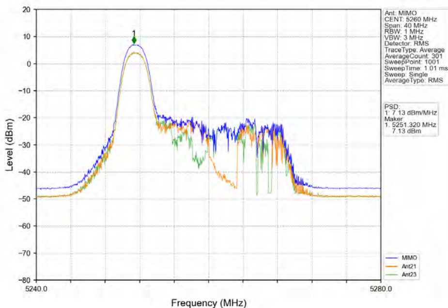
802.11ax(HE20) LCH 5260MHz RU26 Left MIMO NTNV
