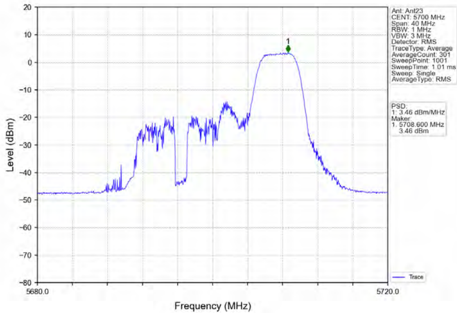
802.11ax(HE20) HCH 5700MHz RU52 Right MIMO NTNV
