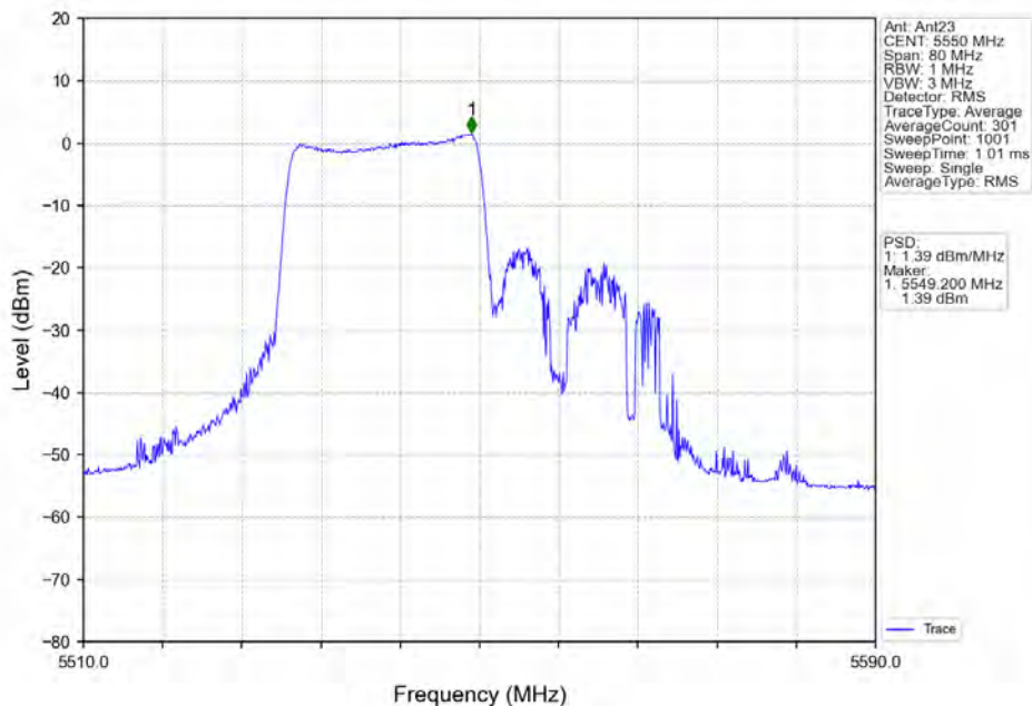
802.11ax(HE40) MCH 5550MHz RU242 Left Ant23 NTVN
