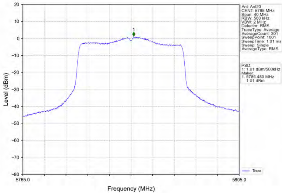
802.11ax(HE20) MCH 5785MHz RU242 Left MIMO NTNV
