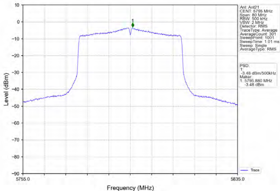
802.11ax(HE40) HCH 5795MHz RU484 Left Ant21 NTNV
