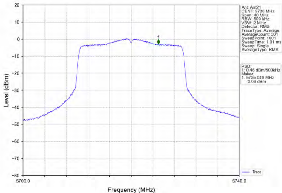
802.11ax(HE20) HCH 5720MHz RU242 Left Ant21 NTN
