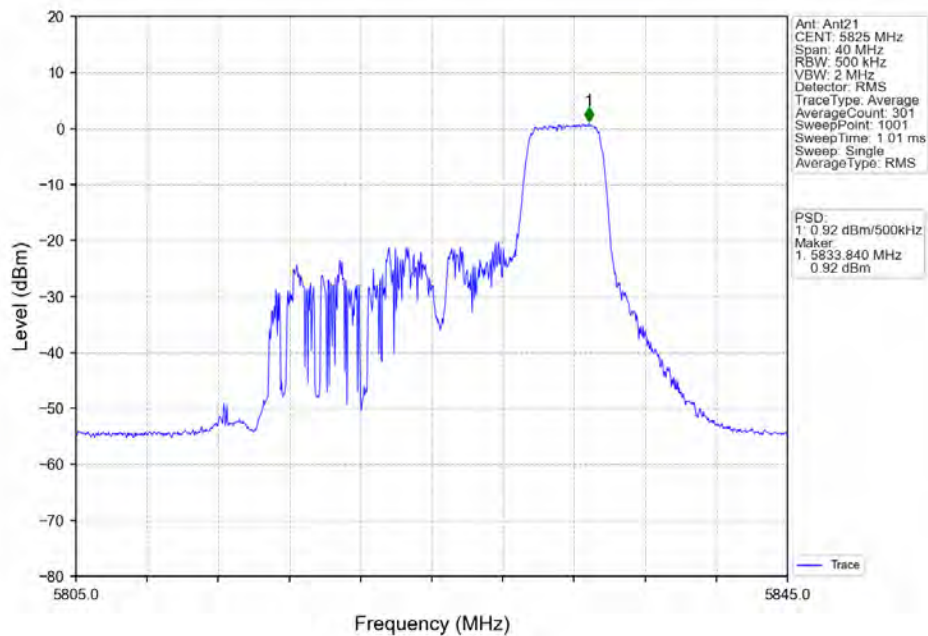
802.11ax(HE20) HCH_5825MHz_RU52_Right Ant21 NTN
