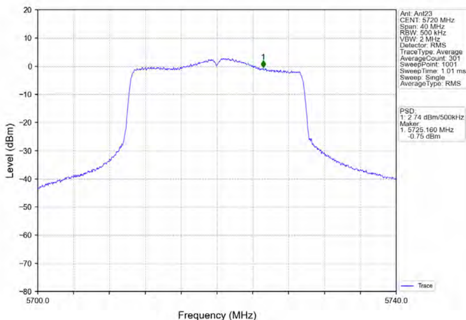
802.11ax(HE20) HCH 5720MHz RU242 Left MIMO NTNV
