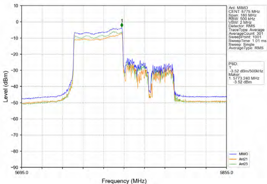
802.11ax(HE80) MCH 5775MHz RU484 Left MIMO NTNV
