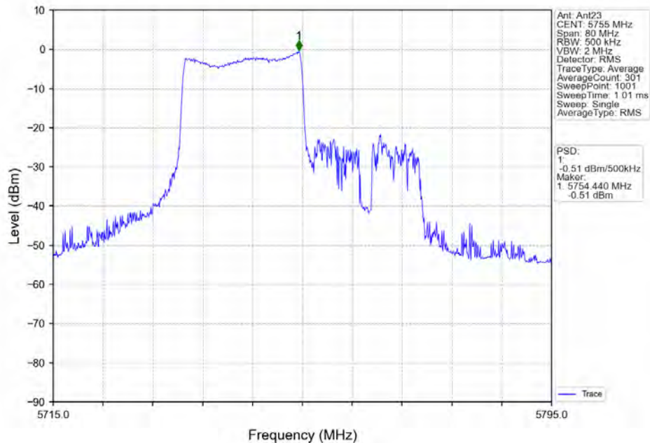
802.11ax(HE40) LCH_5755MHz_RU242_Left_MIMO_NTNV
