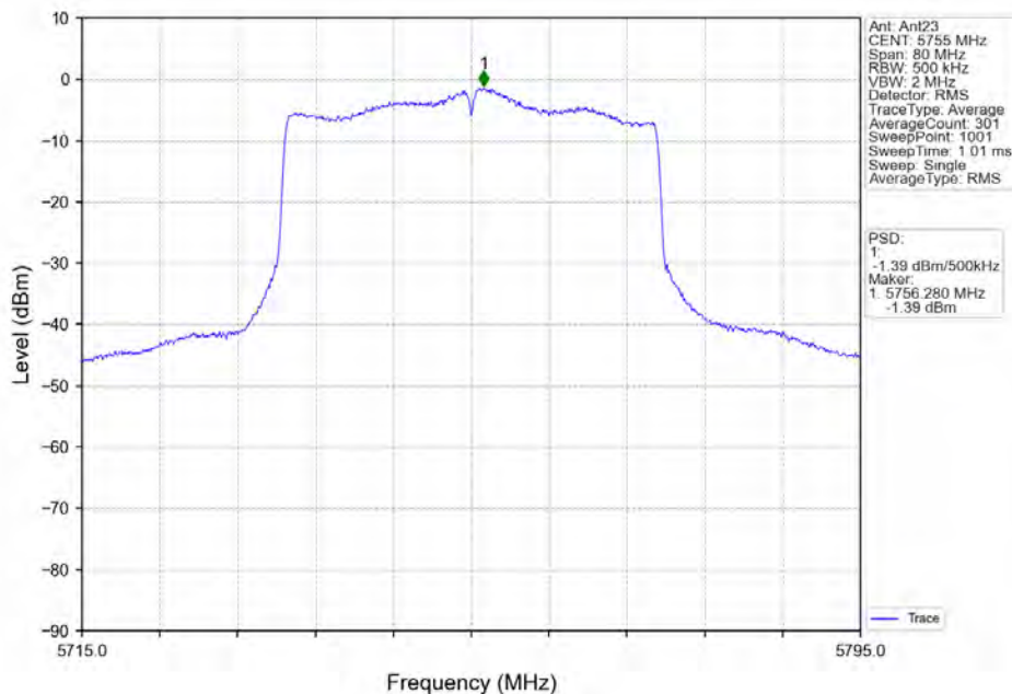
802.11ax(HE40) LCH_5755MHz RU484 Left Ant23_NTNV
