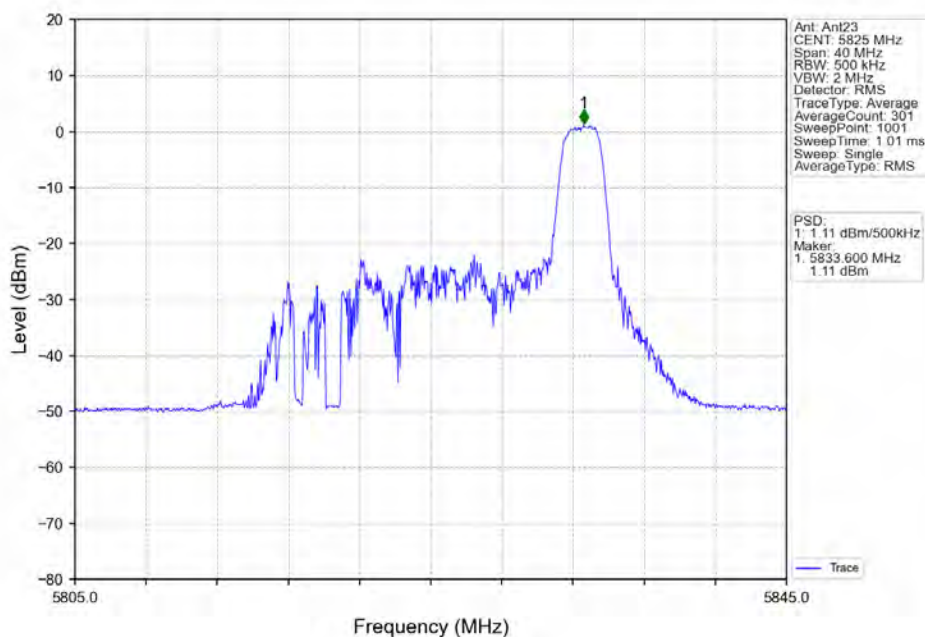
802.11ax(HE20) HCH_5825MHz_RU26_Right_Ant23_NTNV
