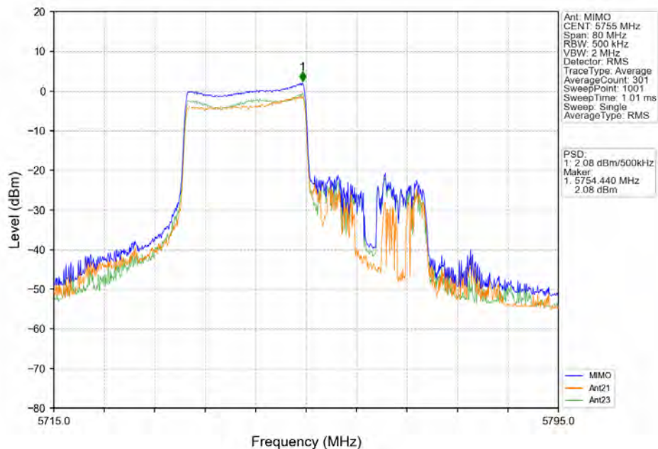
802.11ax(HE40) LCH_5755MHz_RU242_Left_MIMO_NTNV
