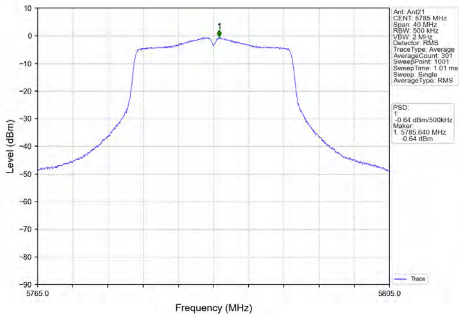
802.11n(HT20) MCH_5785MHz_Ant21_NTNV
