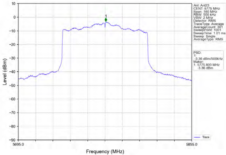
802.11ax(HE80) MCH 5775MHz RU996 Left MIMO NTN
