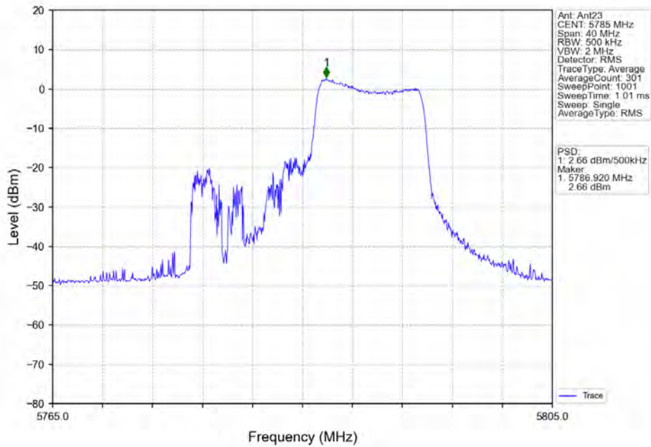
802.11ax(HE20) MCH 5785MHz RU106 Left MIMO NTNV
