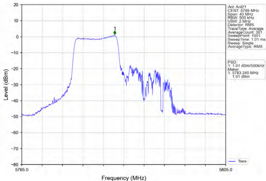
802.11ax(HE20) MCH 5785MHz RU106 Left Ant21_NTNV
