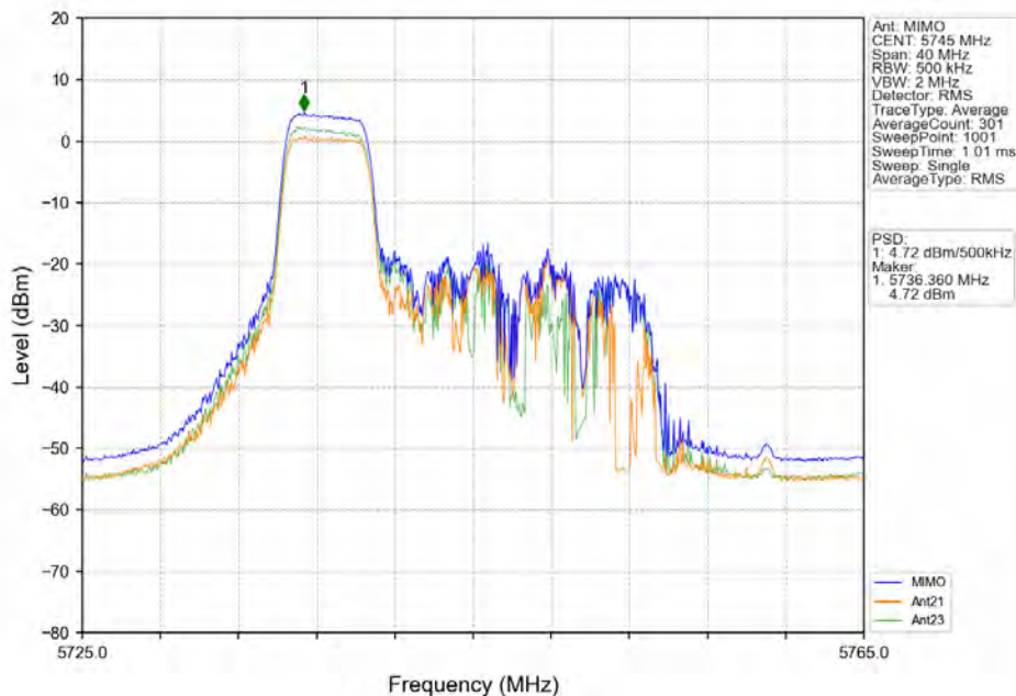
802.11ax(HE20) LCH 5745MHz RU52 Left MIMO NTV
