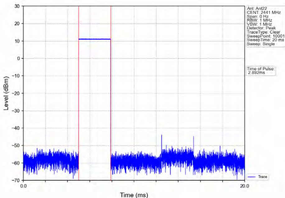
GFSK_DH5_HOPP_Ant22_NTNV
