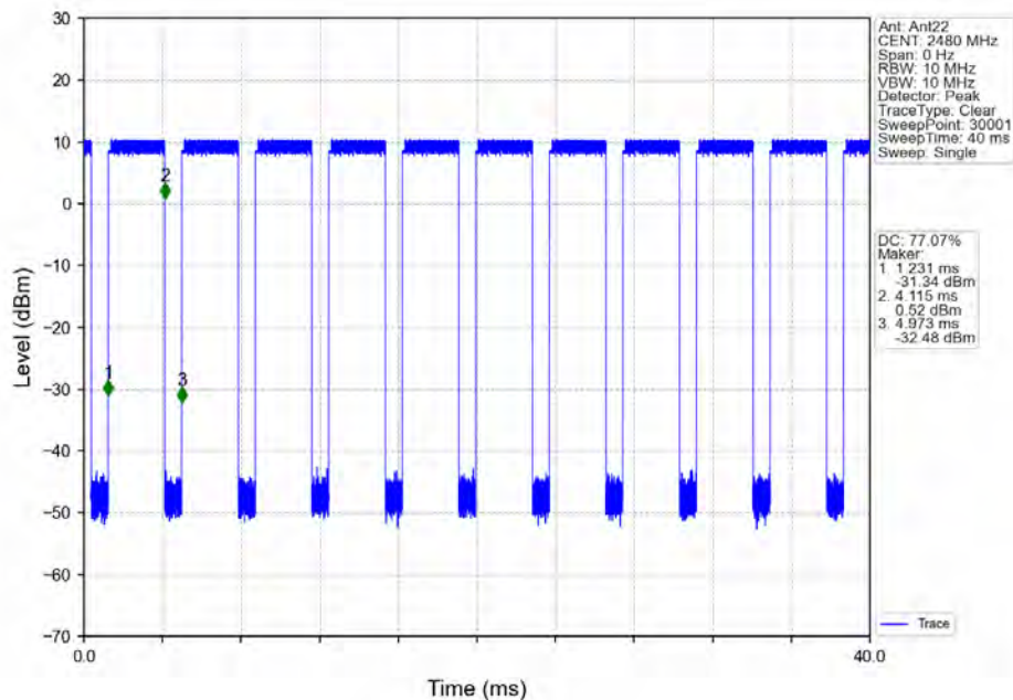
Pi/4DQPSK 2DH5 HCH 2480MHz Ant22 NTN
