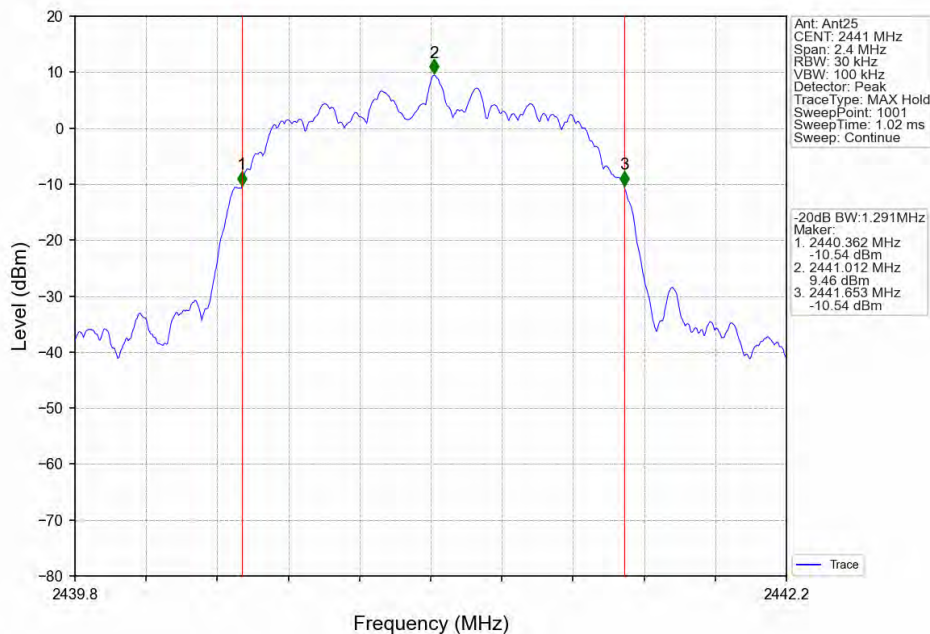
Pi/4DQPSK 2DH5 MCH 2441MHz Ant25 NTN
