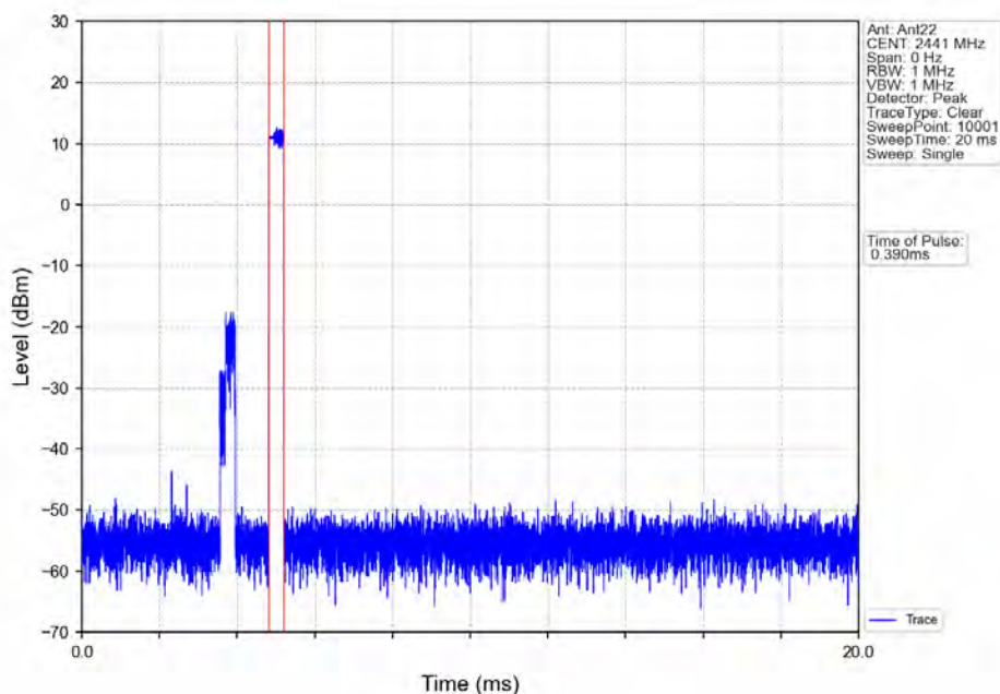
8DPSK_3DH1_HOPP_Ant22_NTNV
