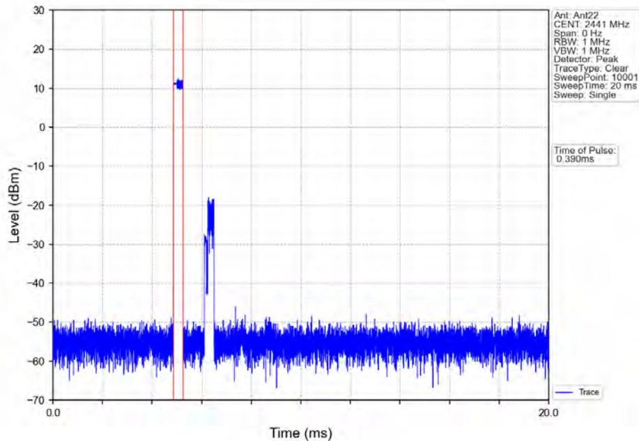
Pi/4DQPSK_2DH1_HOPP_Ant22_NTNV
