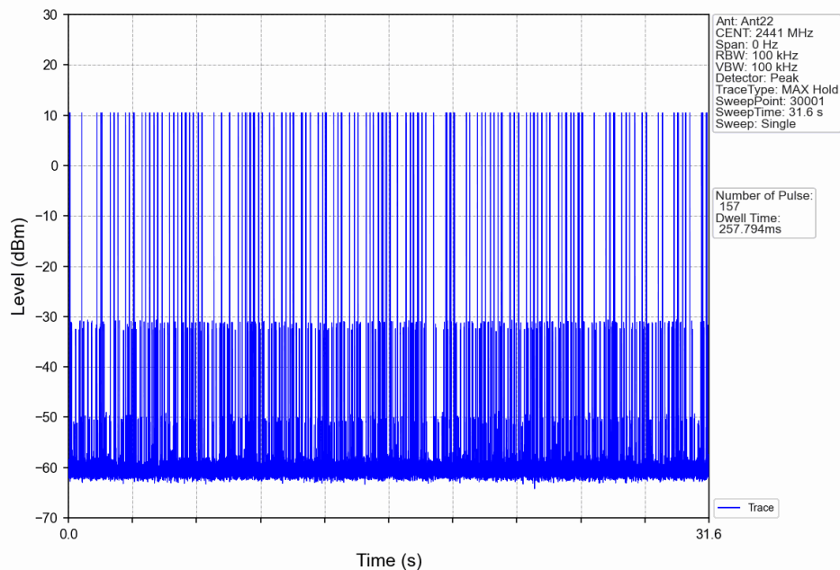
8DPSK_3DH3_HOPP_Ant22_NTNV
