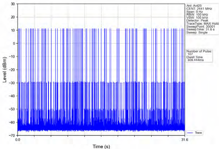
GFSK_DH5_HOPP_Ant25_NTNV
