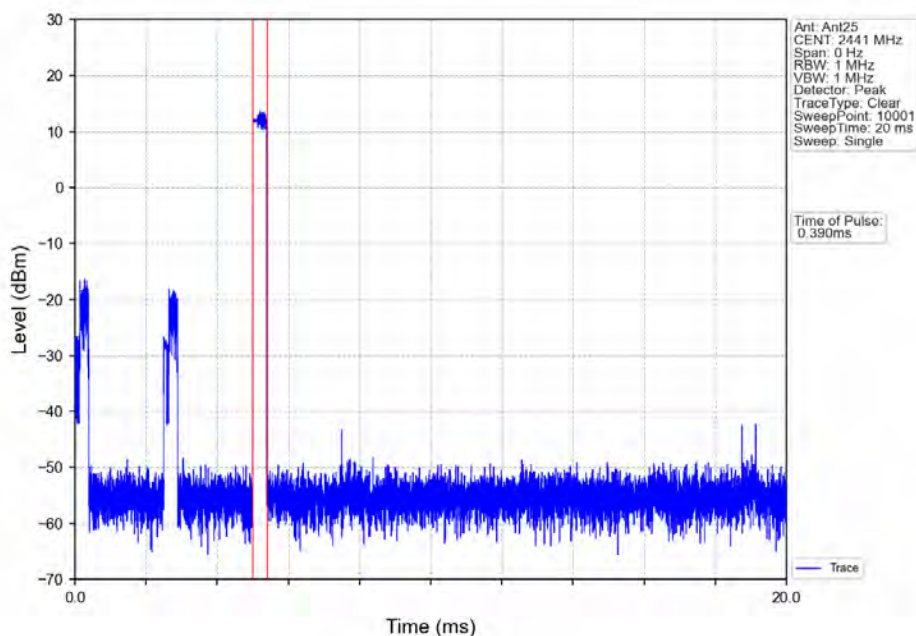
8DPSK_3DH1_HOPP_Ant25_NTNV
