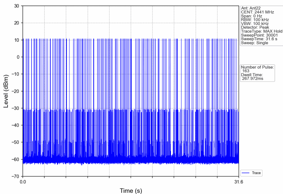
Pi/4DQPSK_2DH3_HOPP_Ant22_NTNV
