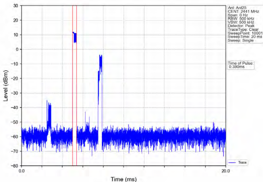
Pi/4DQPSK_2DH1_HOPP_Ant25_NTNV
