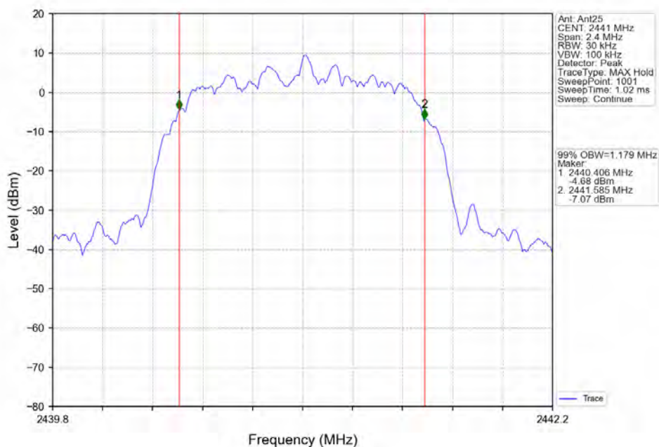
Pi/4DQPSK 2DH5 MCH 2441MHz Ant25 NTN
