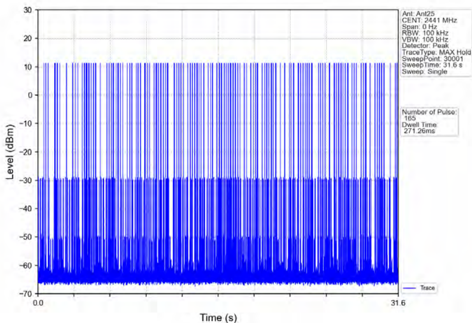
GFSK_DH3_HOPP_Ant25_NTNV
