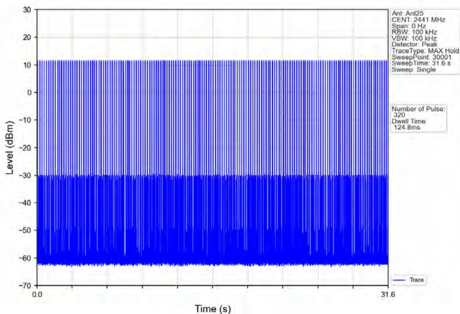
8DPSK_3DH1_HOPP_Ant25_NTNV
