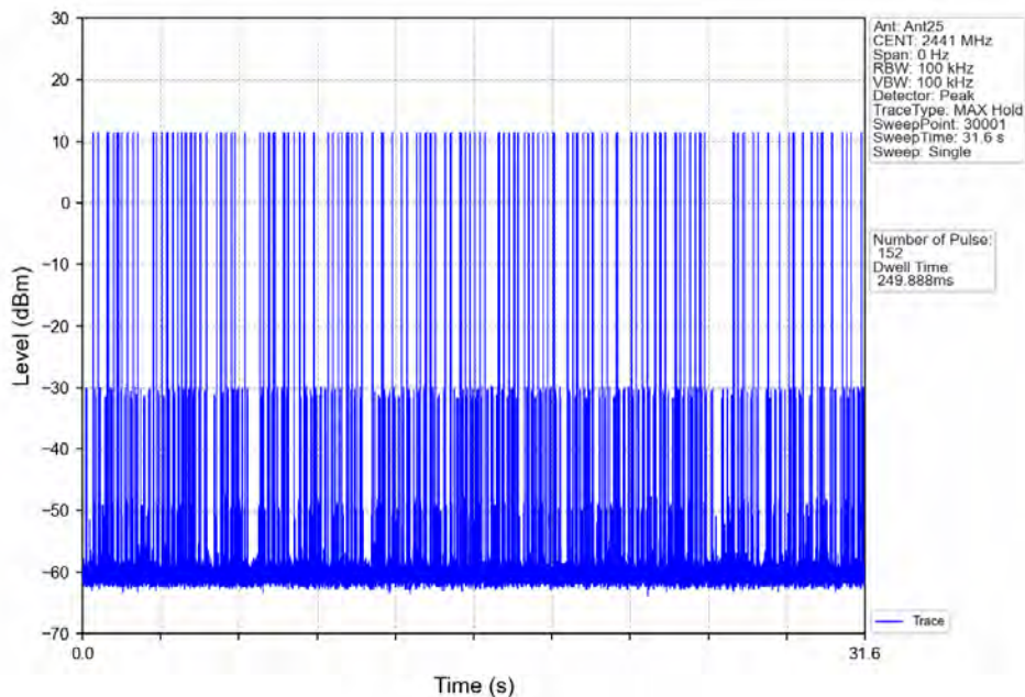
Pi/4DQPSK_2DH3_HOPP_Ant25_NTNV
