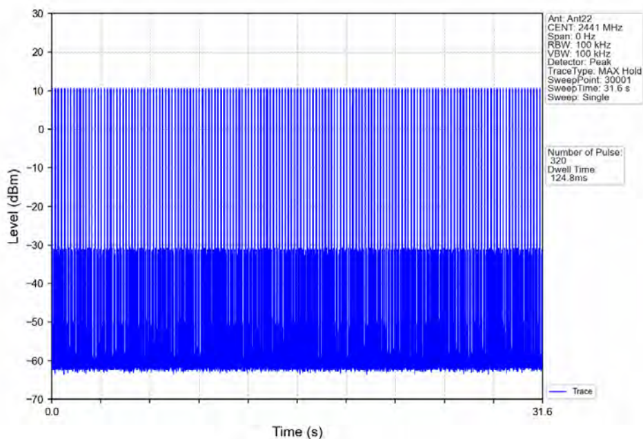
8DPSK_3DH1_HOPP_Ant22_NTNV
