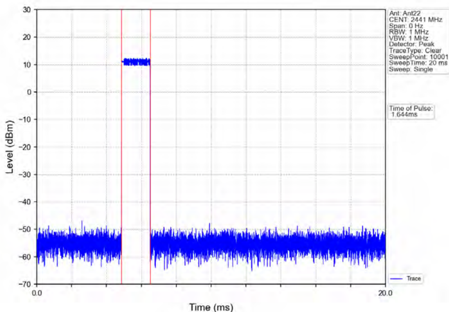
Pi/4DQPSK_2DH3_HOPP_Ant22_NTNV
