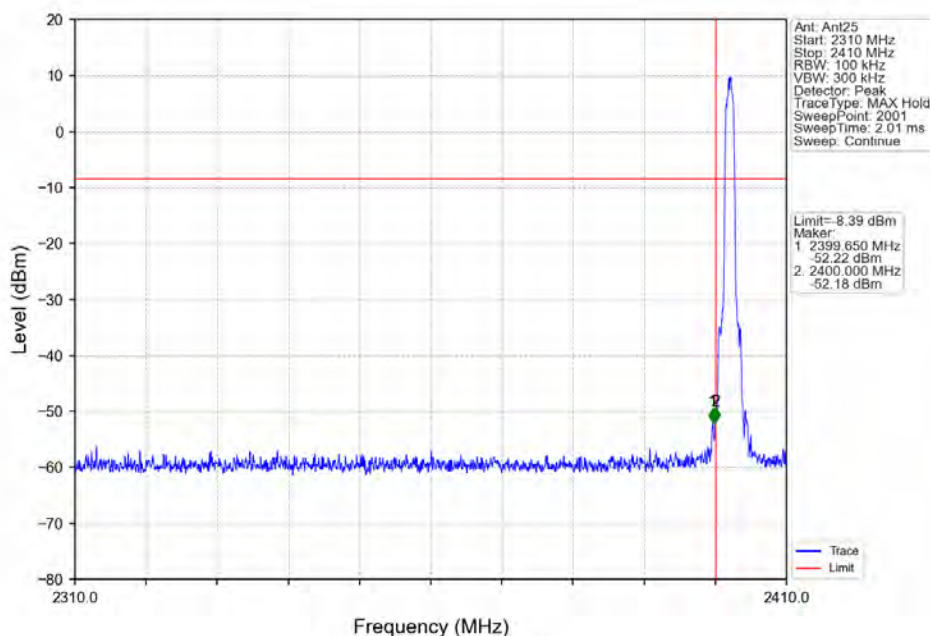
Pi/4DQPSK 2DH5 LCH 2402MHz Ant25 NTNV
