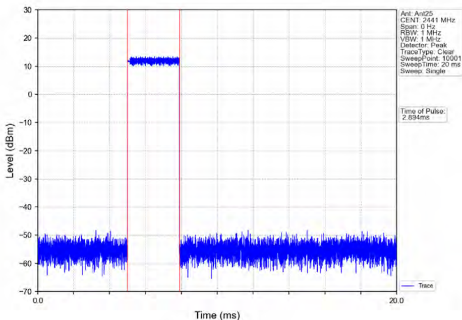
8DPSK_3DH5_HOPP_Ant25_NTNV
