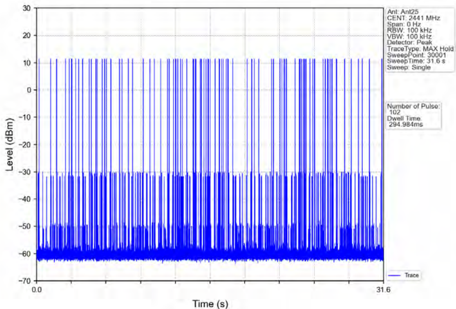
Pi/4DQPSK 2DH5 HOPP Ant25 NTN
