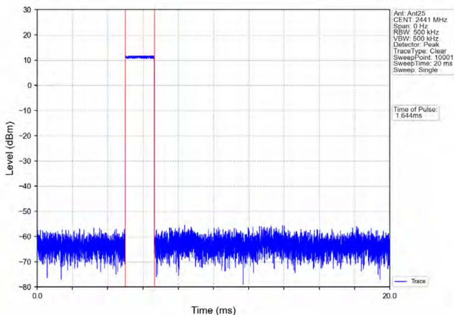
GFSK_DH3_HOPP_Ant25_NTNV
