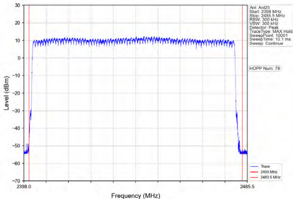
8DPSK_3DH5_HOPP_Ant25_NTNV
