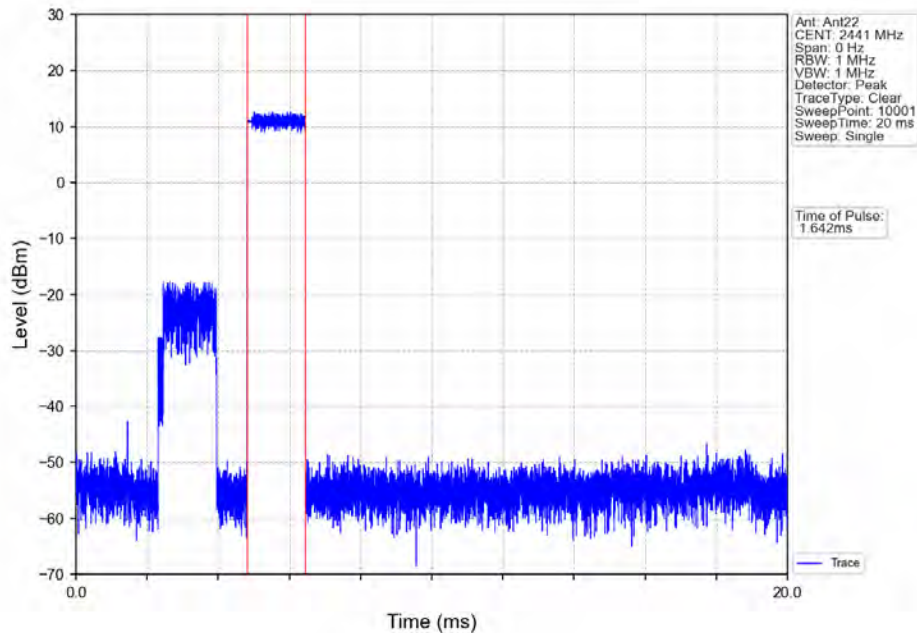
8DPSK_3DH3_HOPP_Ant22_NTNV
