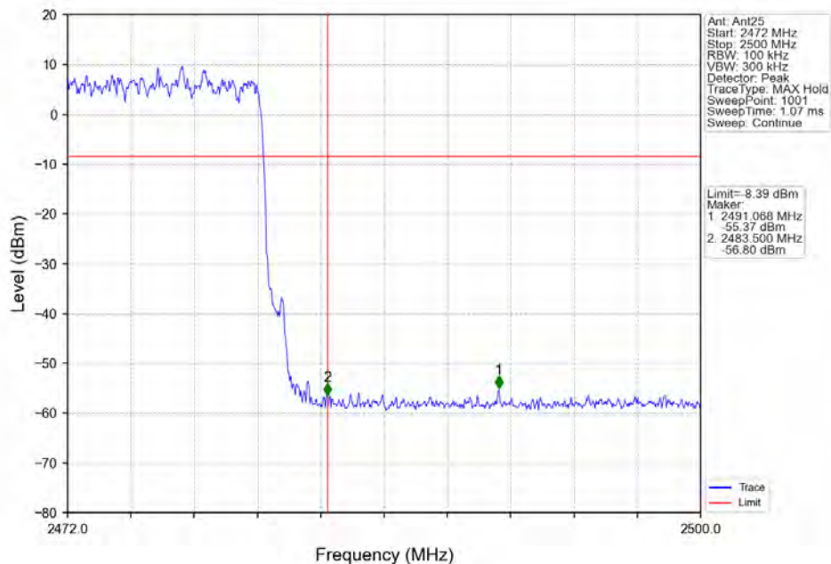
Pi/4DQPSK_2DH5_HOPP_Ant25_NTNV
