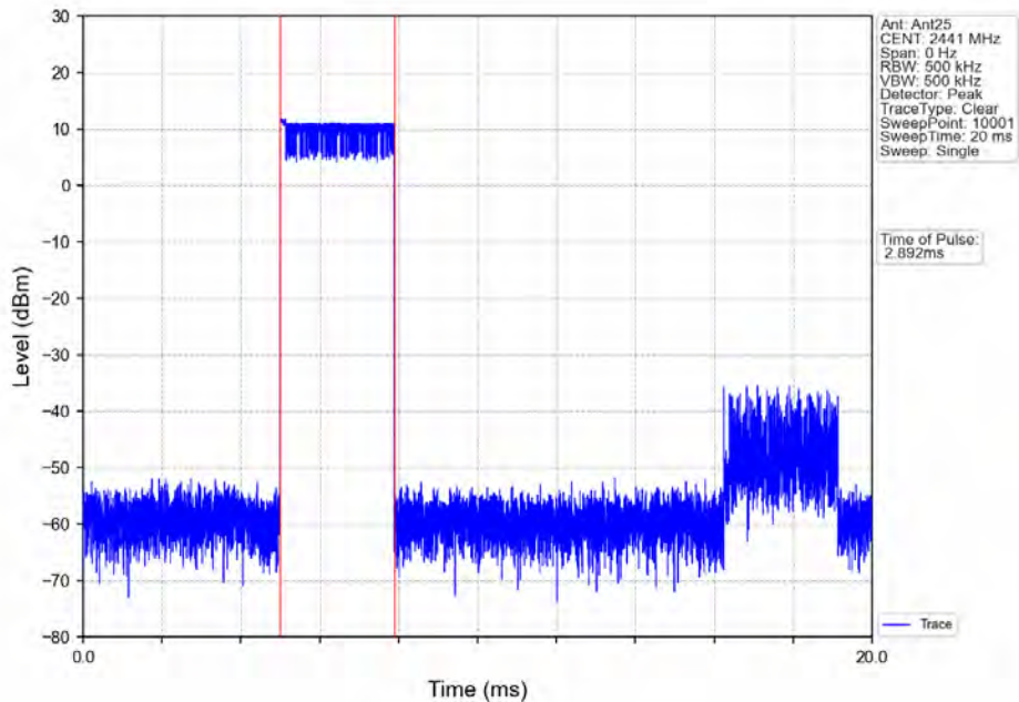
Pi/4DQPSK 2DH5 HOPP Ant25 NTN
