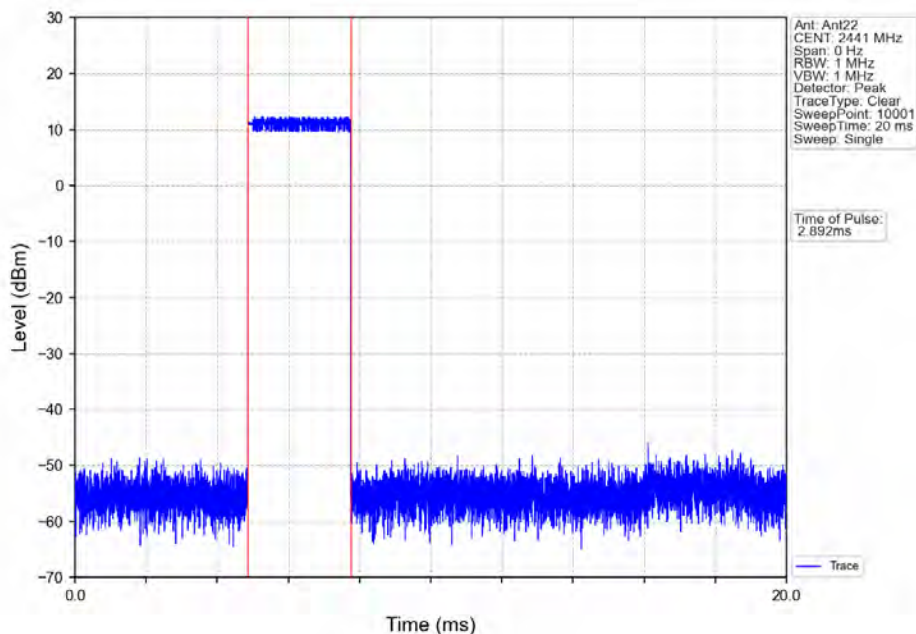
Pi/4DQPSK_2DH5_HOPP_Ant22_NTNV
