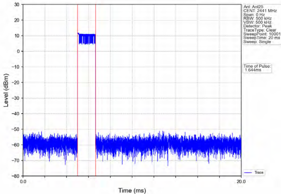
Pi/4DQPSK_2DH3_HOPP_Ant25_NTNV
