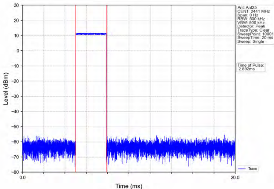
GFSK_DH5_HOPP_Ant25_NTNV
