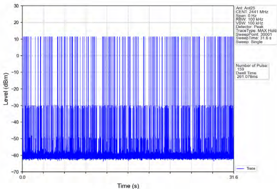
8DPSK_3DH3_HOPP_Ant25_NTNV
