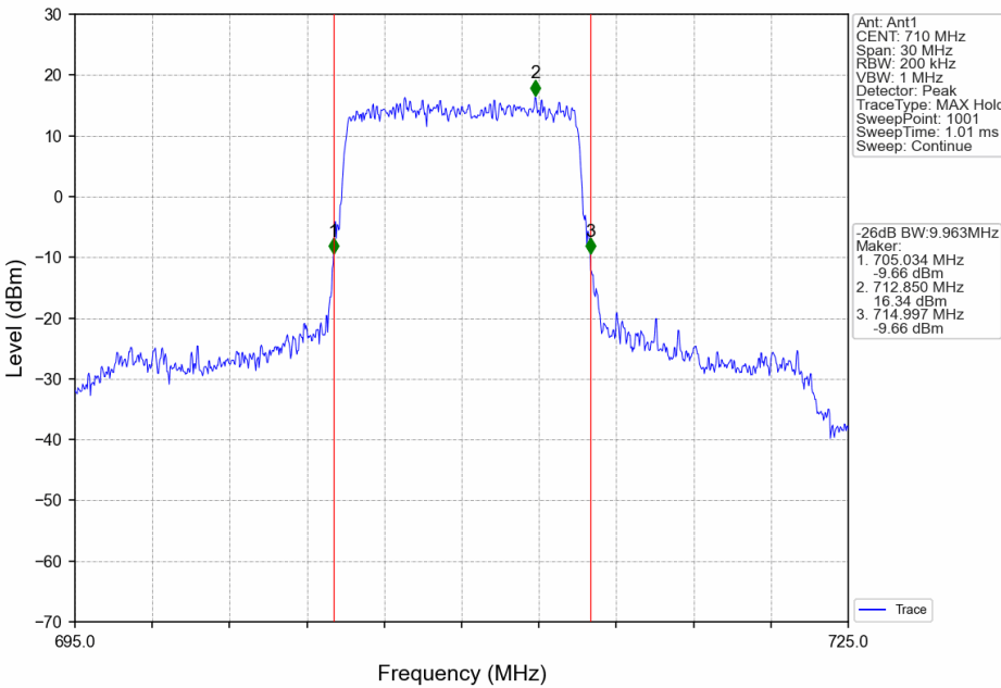
Band17_10MHz_QPSK_MCH_710MHz_RB_50_0_NTNV
