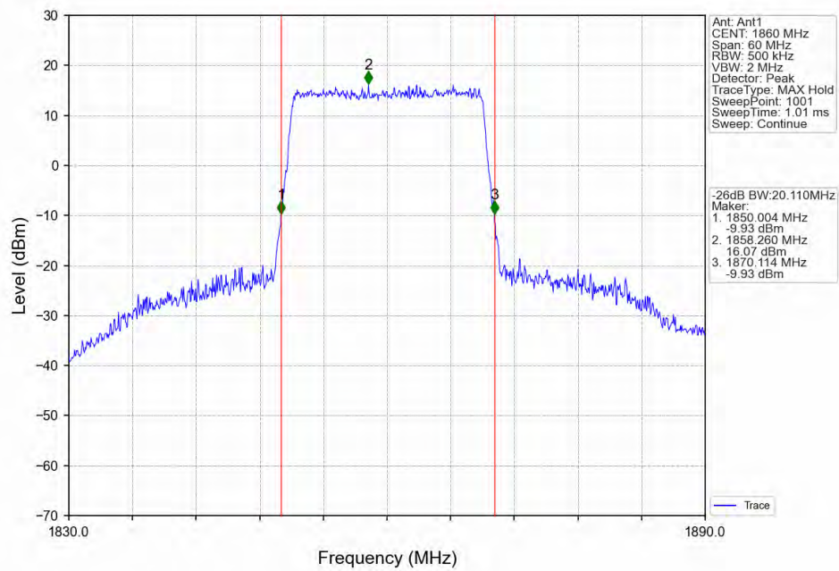
Band2_20MHz_256QAM_LCH_1860MHz_RB_100_0_NTNV
