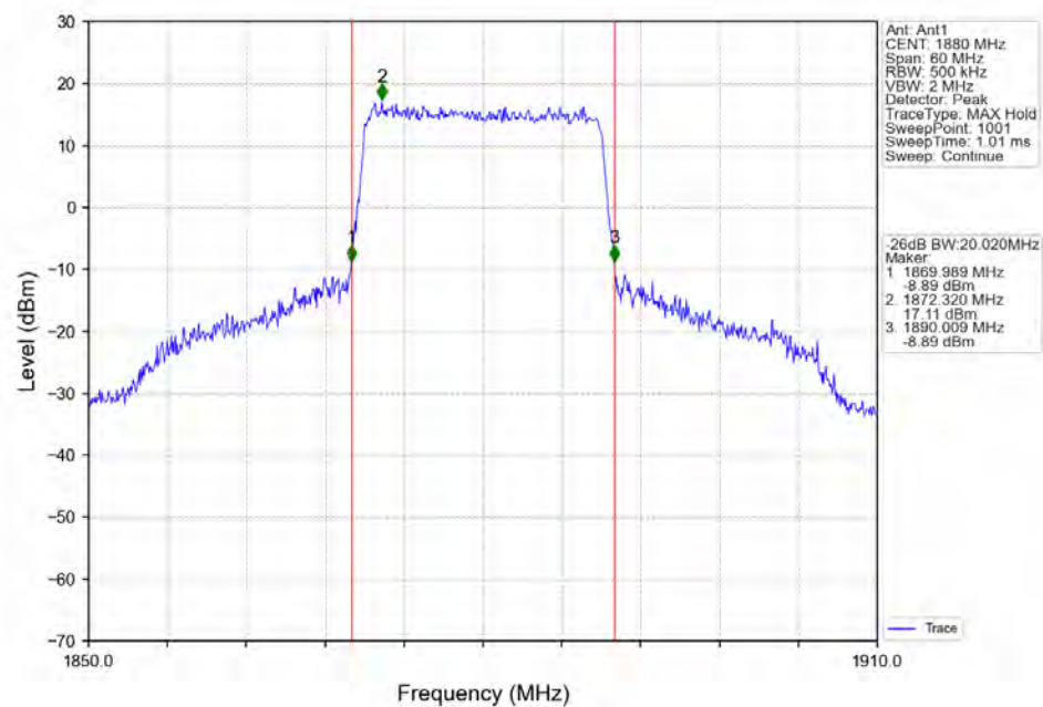
Band2_20MHz_64QAM_MCH_1880MHz_RB_100_0_NTNV
