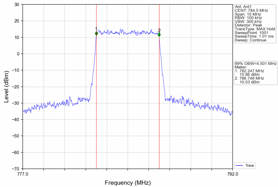
Band13 5MHz 16QAM HCH 784.5MHz RB 25 0 NTN
