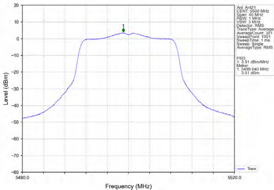
802.11n(HT20)_LCH_5500MHz_Ant21_NTNV
