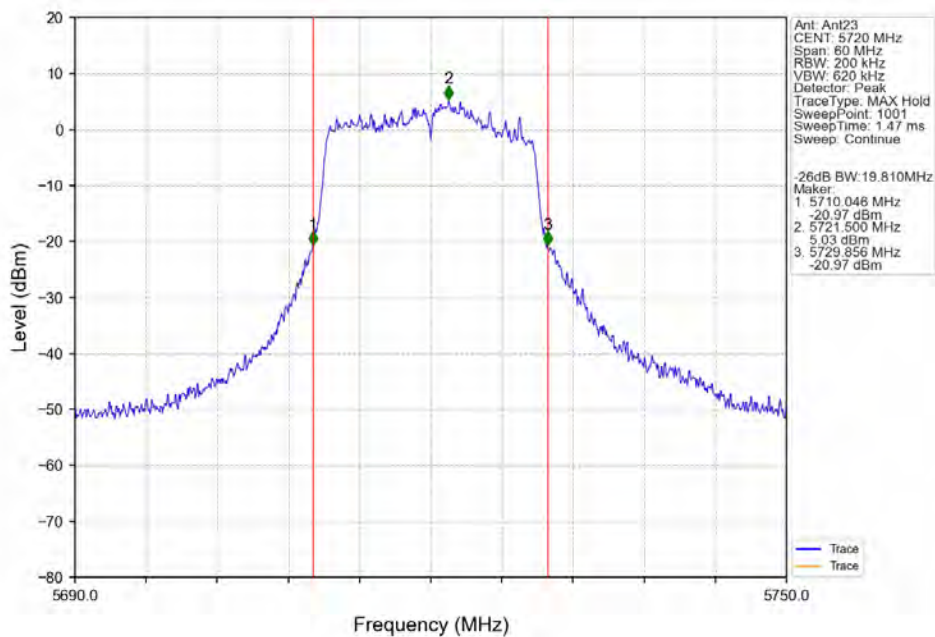
802.11n(HT20)_HCH_5720MHz_Ant23_NTNV
