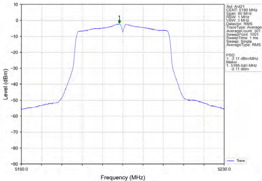
802.11n(HT40)_LCH_5190MHz_Ant21_NTNV
