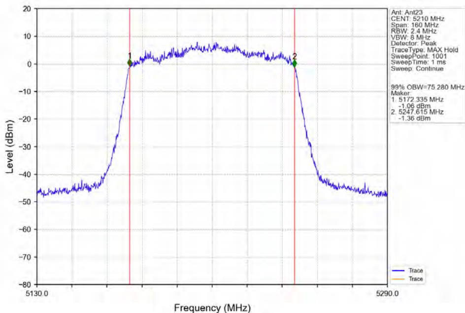
802.11ac(VHT80)_MCH_5210MHz_Ant23_NTNV
