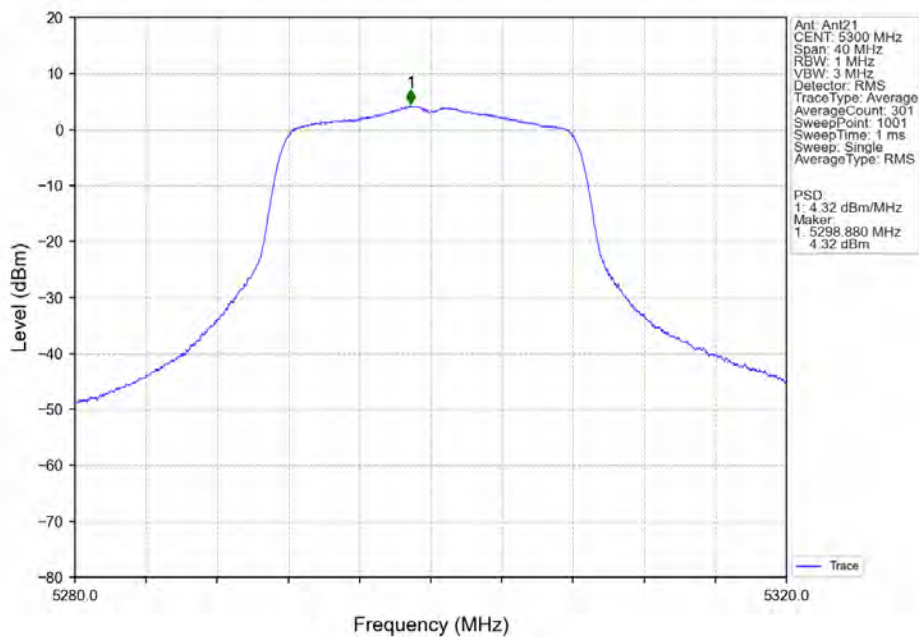
802.11a_MCH_5300MHz_Ant21_NTNV
