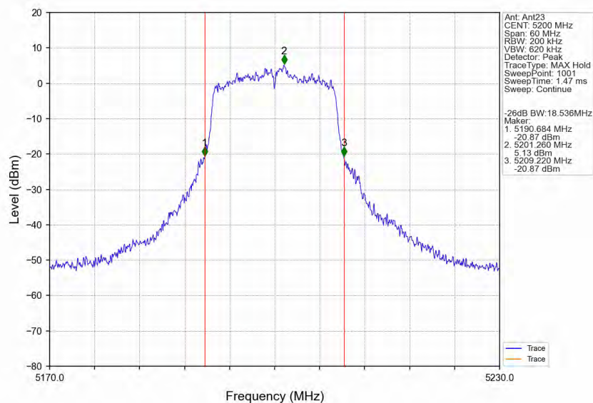
802.11a_MCH_5200MHz_Ant23_NTNV
