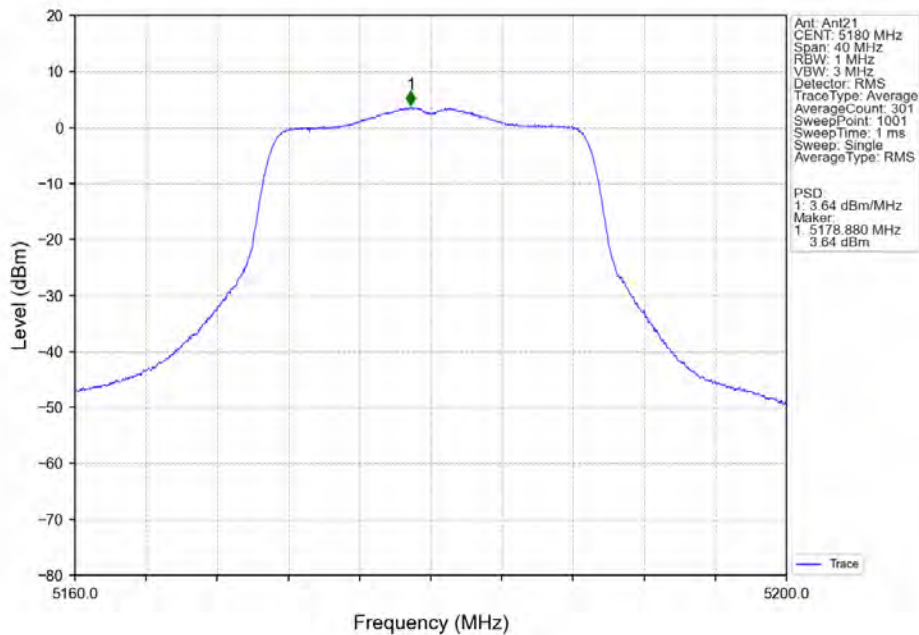
802.11n(HT20)_LCH_5180MHz_Ant21_NTNV
