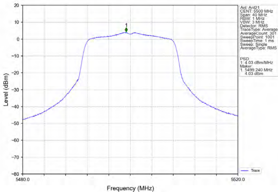
802.11a_LCH_5500MHz_Ant21_NTNV
