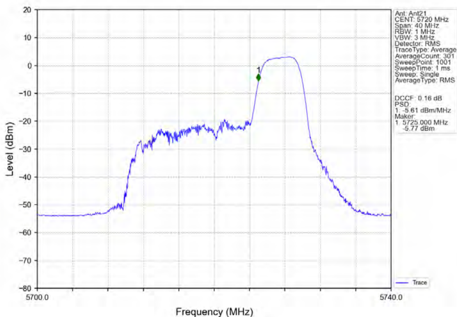
802.11ax(HEW20)_HCH_5720MHz_RU52_Right_Ant21_NTNV
