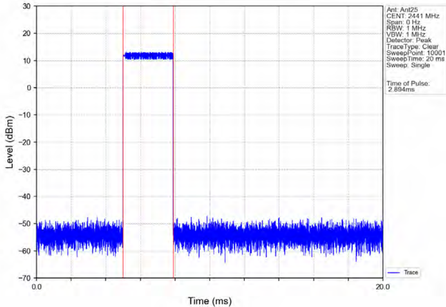
Pi/4DQPSK_2DH5_HOPP_Ant25_NTNV
