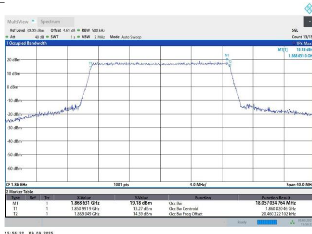
Band2-20MHz-QPSK-18700-100RB#0-18.06-20.02
