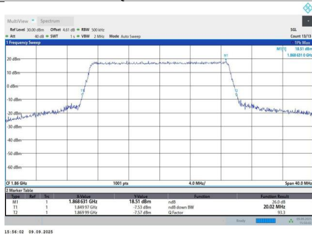
Band2-20MHz-QPSK-18700-100RB#0-18.06-20.02
