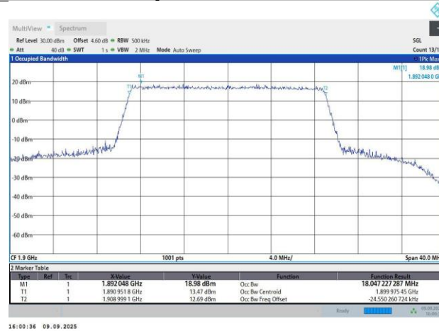
Band2-20MHz-QPSK-19100-100RB#0-18.05-20.06
