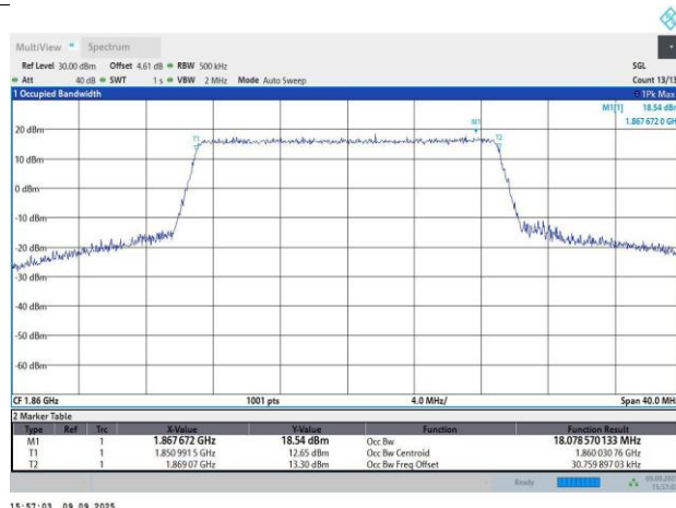
Band2-20MHz-16QAM-18700-100RB#0-18.08-20.02
