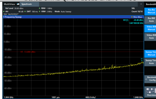
Band2-3MHz-QPSK-18615-1RB#0-PASS
