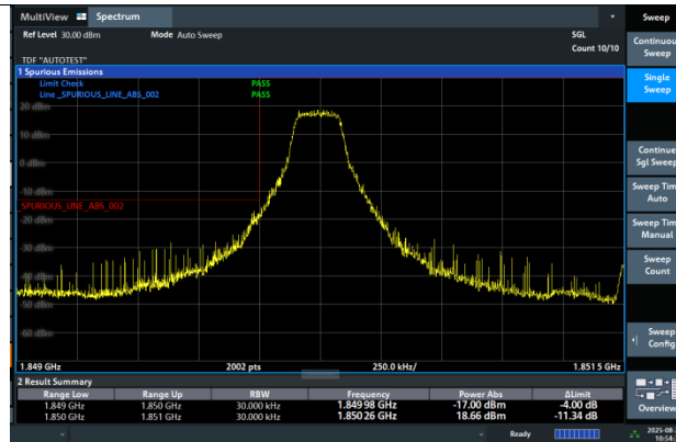
Band2-3MHz-QPSK-18615-1RB#0-PASS
