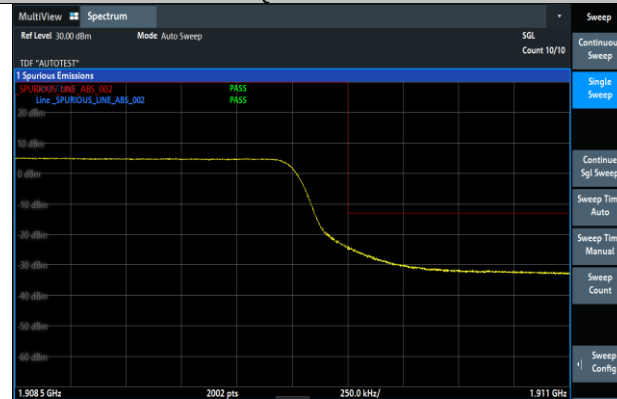
Band2-5MHz-16QAM-19175-12RB#13-PASS
