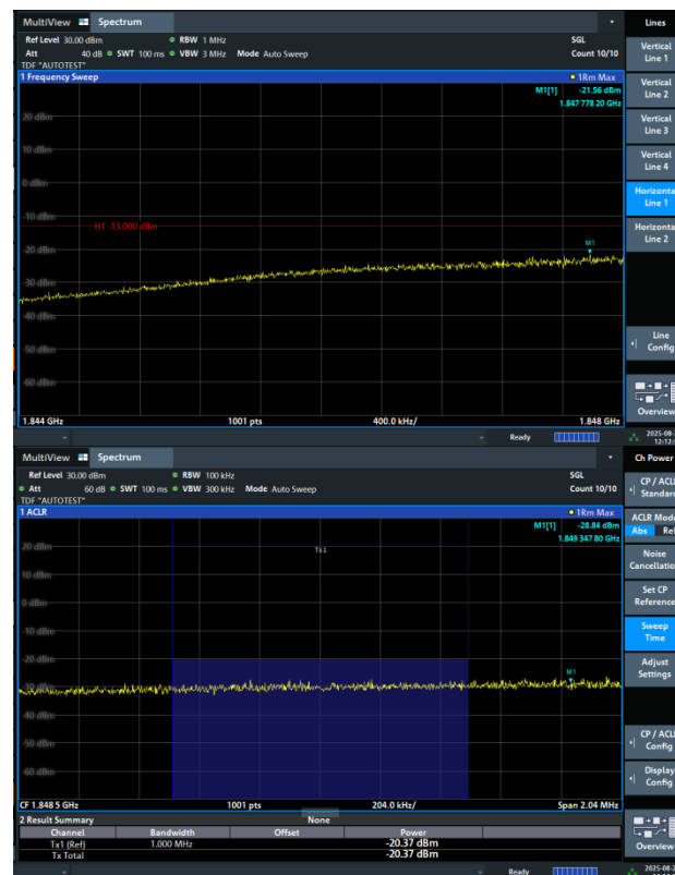
Band2-5MHz-QPSK-18625-12RB#0-PASS
