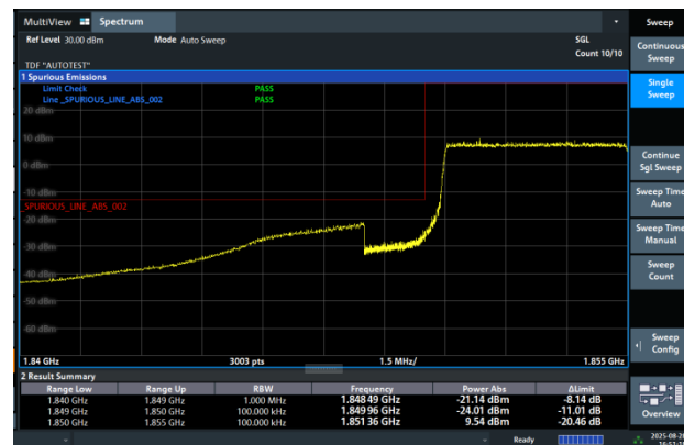
Band2-10MHz-QPSK-18650-25RB#0-PASS
