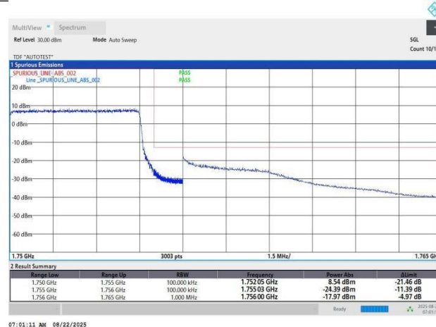
Band4-10MHz-QPSK-20350-25RB#25-PASS
