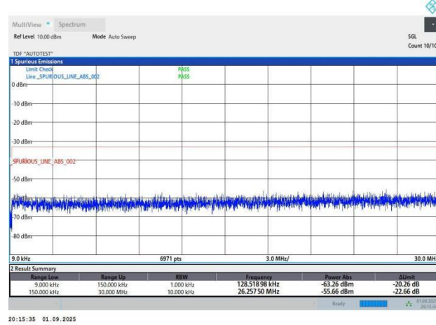
Band4-10MHz-QPSK-20000-1RB#0-PASS
