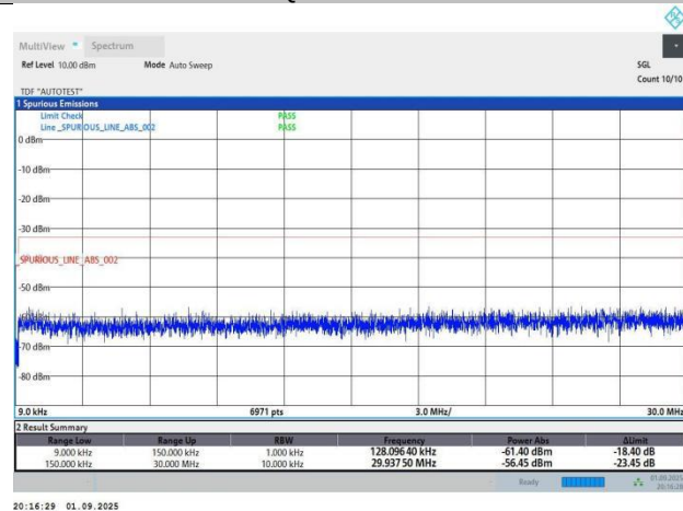
Band4-10MHz-QPSK-20350-1RB#0-PASS
