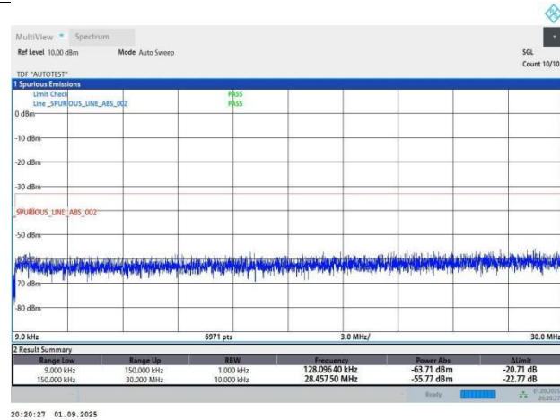
Band4-20MHz-QPSK-20175-1RB#0-PASS
