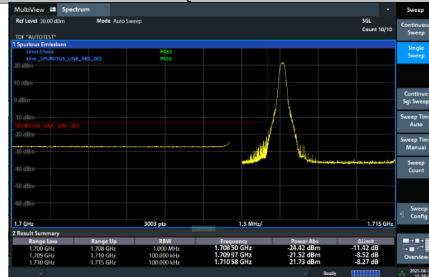
Band4-10MHz-QPSK-20000-1RB#0-PASS
