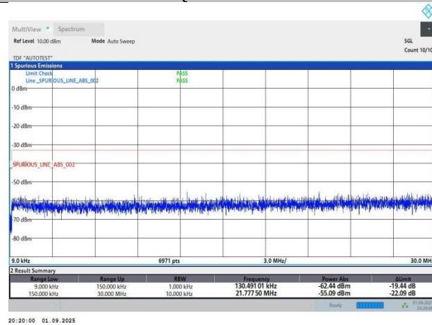
Band4-20MHz-QPSK-20050-1RB#0-PASS
