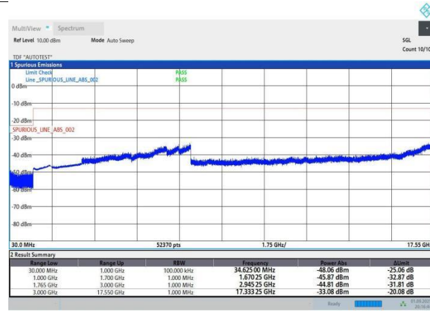
Band4-10MHz-QPSK-20350-1RB#0-PASS
