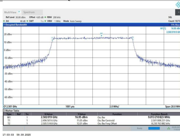
Band41-10MHz-QPSK-39700-50RB#0-9.01-10.07
