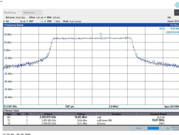
Band41-10MHz-QPSK-39700-50RB#0-9.01-10.07
