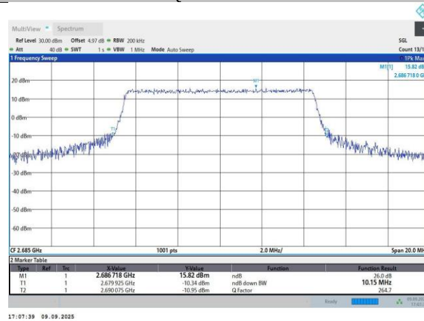
Band41-10MHz-16QAM-41540-50RB#0-9.02-10.15
