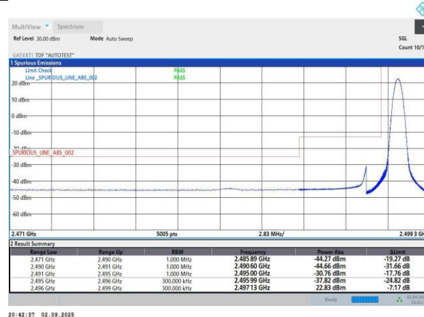
41-41-5MHz-20MHz-QPSK-QPSK-39683-39800-1#0-0#0-PASS
