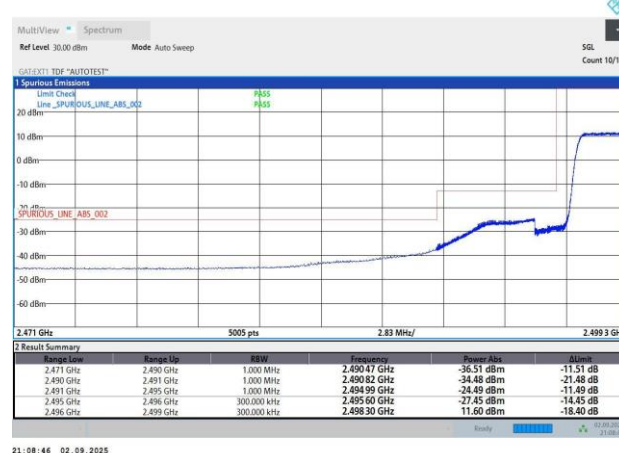
41-41-5MHz-20MHz-QPSK-QPSK-39683-39800-25#0-0#0-PASS
