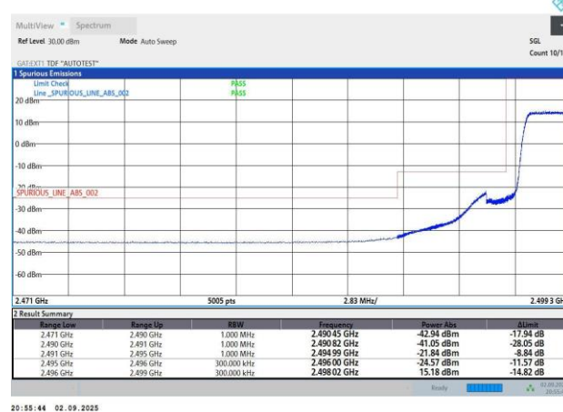
41-41-5MHz-20MHz-QPSK-QPSK-39683-39800-12#0-0#0-PASS
