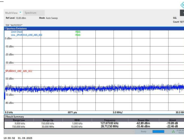
WCDMA BAND 4-1312-PASS
