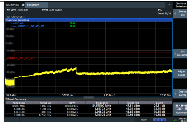
WCDMA BAND 4-1413-PASS
