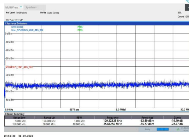
WCDMA BAND 4-1513-PASS
