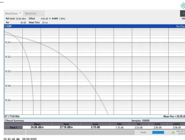
WCDMA BAND 4-1312-2.9-13-PASS
