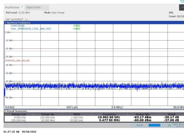
N26-15KHz-10MHz-CP-OFDM QPSK-167300-1RB#0-PASS
