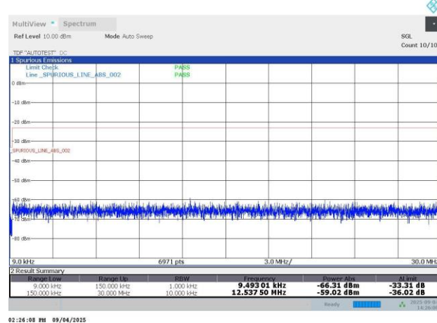
N26-15KHz-20MHz-CP-OFDM QPSK-166800-106RB#0-PASS
