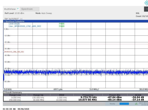
N26-15KHz-20MHz-CP-OFDM QPSK-167800-1RB#0-PASS
