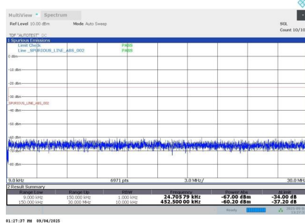
N26-15KHz-10MHz-CP-OFDM QPSK-165800-1RB#51-PASS
