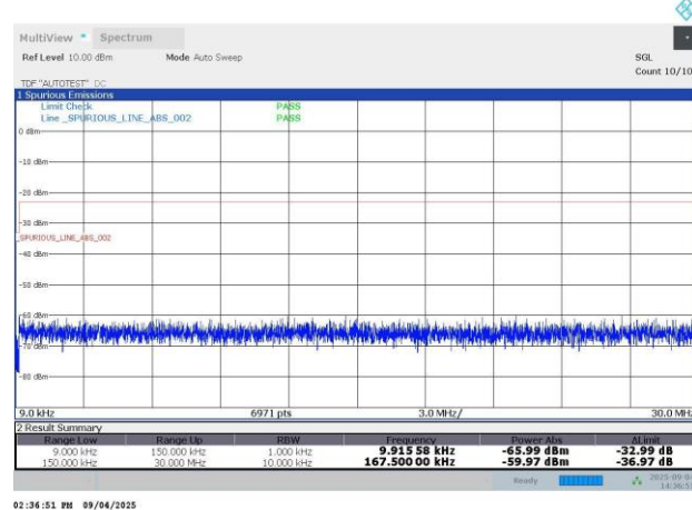
N26-15KHz-20MHz-CP-OFDM QPSK-167300-106RB#0-PASS
