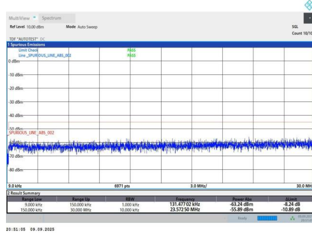
N41-30KHz-60MHz-CP-OFDM QPSK-518598-162RB#0-PASS
