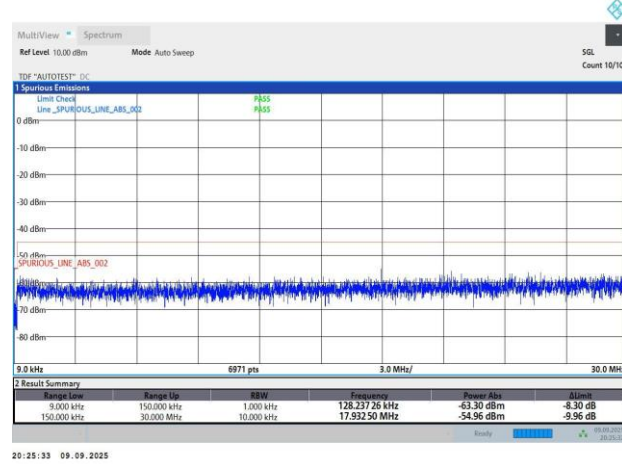
N41-30KHz-10MHz-DFT-s-OFDM PI/2 BPSK-500202-24RB#0-PASS
