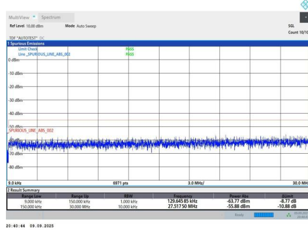
N41-30KHz-10MHz-DFT-s-OFDM PI/2 BPSK-537000-1RB#0-PASS
