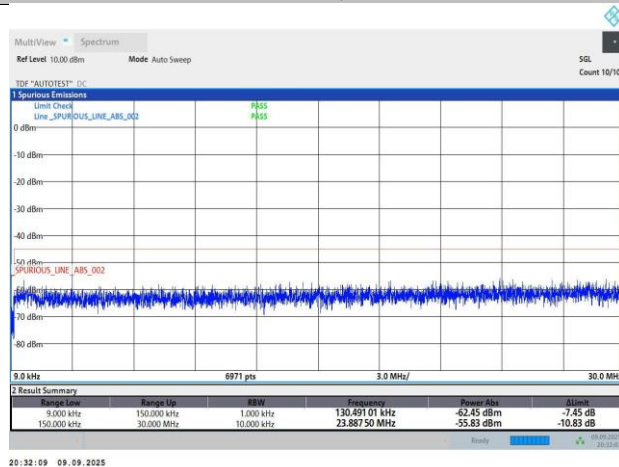
N41-30KHz-10MHz-DFT-s-OFDM PI/2 BPSK-518598-24RB#0-PASS
