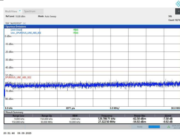
N41-30KHz-60MHz-DFT-s-OFDM QPSK-518598-162RB#0-PASS
