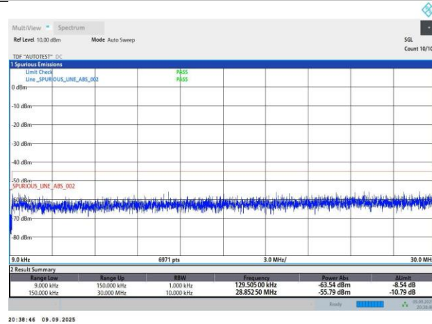
N41-30KHz-10MHz-DFT-s-OFDM PI/2 BPSK-537000-24RB#0-PASS
