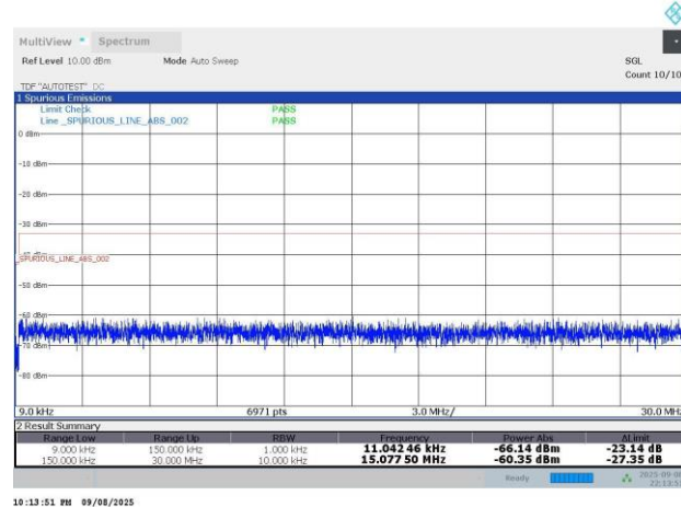
N66-15KHz-20MHz-CP-OFDM QPSK-349000-1RB#105-PASS
