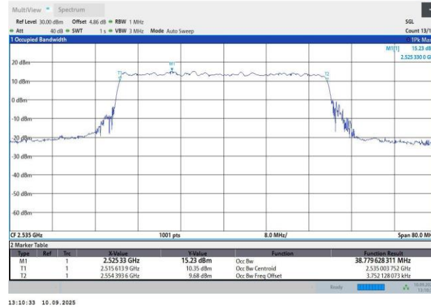
N7-15KHz-40MHz-DFT-s-OFDM QPSK-507000-216RB#0-38.78-42.2
