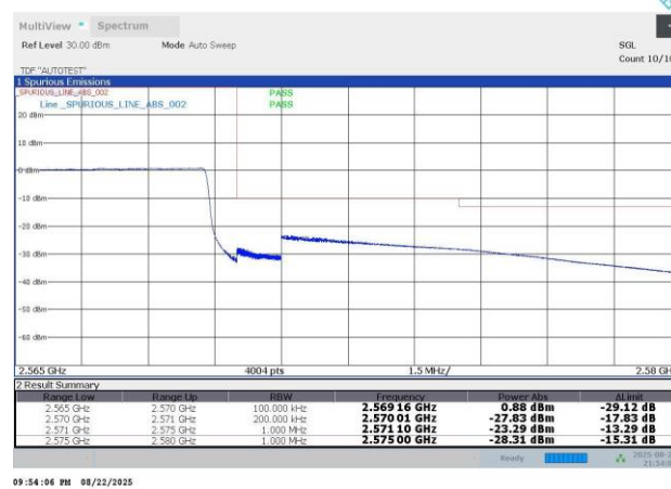
N7-15KHz-10MHz-DFT-s-OFDM QPSK-513000-50RB#0-PASS
