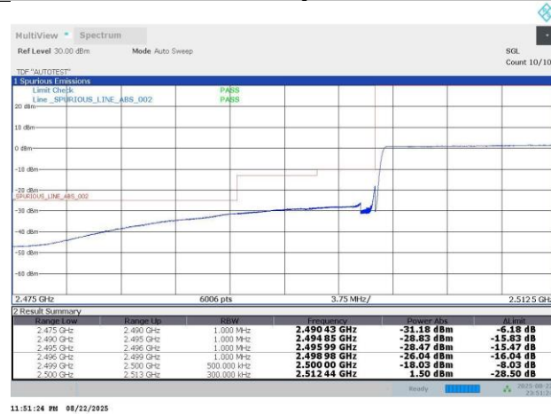
N7-15KHz-25MHz-CP-OFDM QPSK-502500-133RB#0-PASS
