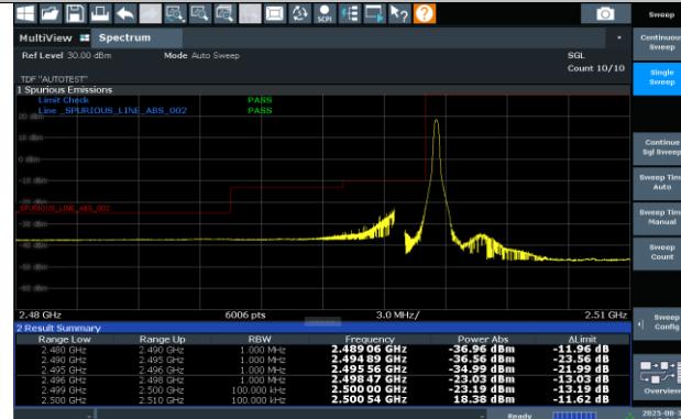
N7-15KHz-20MHz-DFT-s-OFDM QPSK-502000-1RB#0-PASS
