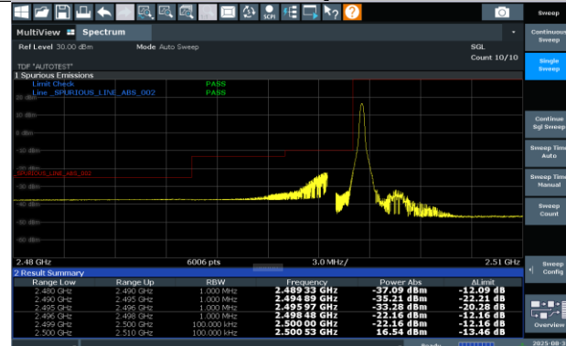
N7-15KHz-20MHz-CP-OFDM QPSK-502000-1RB#0-PASS
