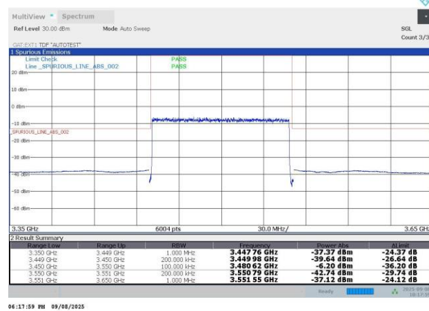
N77-30KHz-100MHz-DFT-s-OFDM PI/2 BPSK-633334-270RB#0-PASS
