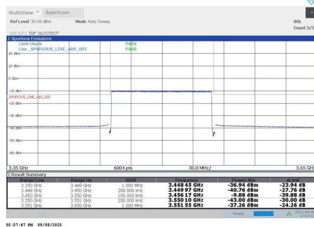
N77-30KHz-100MHz-DFT-s-OFDM QPSK-633334-270RB#0-PASS
