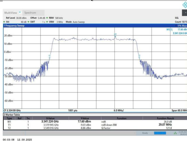
N78-30KHz-30MHz-DFT-s-OFDM PI/2 BPSK-635666-75RB#0-26.92-29.07
