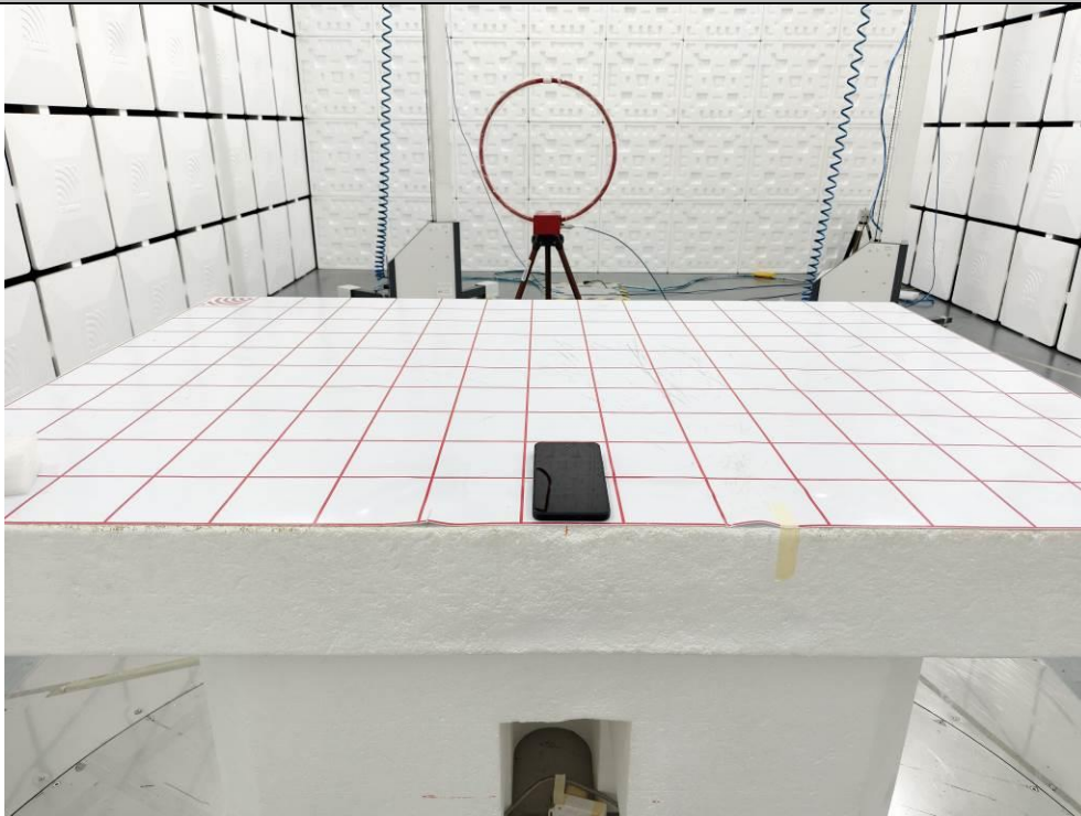
9kHz-30MHz
