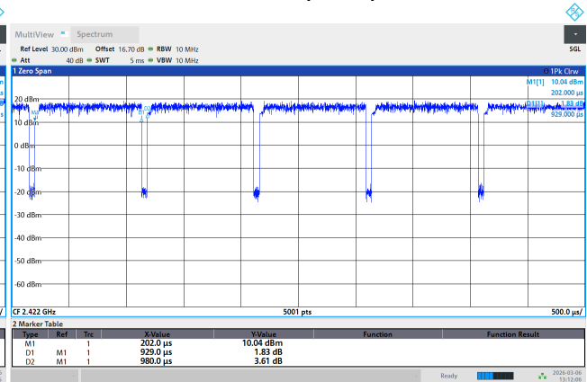
802.11n(HT40)
