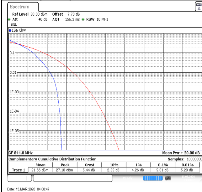
Band26(824-849)-10MHz-QPSK-26990-1RB#0-PASS
