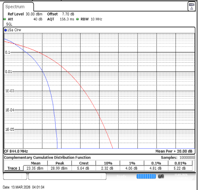
Band26(824-849)-10MHz-QPSK-26990-50RB#0-PASS
