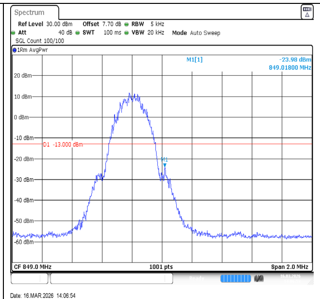
GSM850-251-5-PASS
