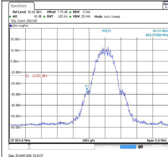
GPRS850-128-5-PASS
