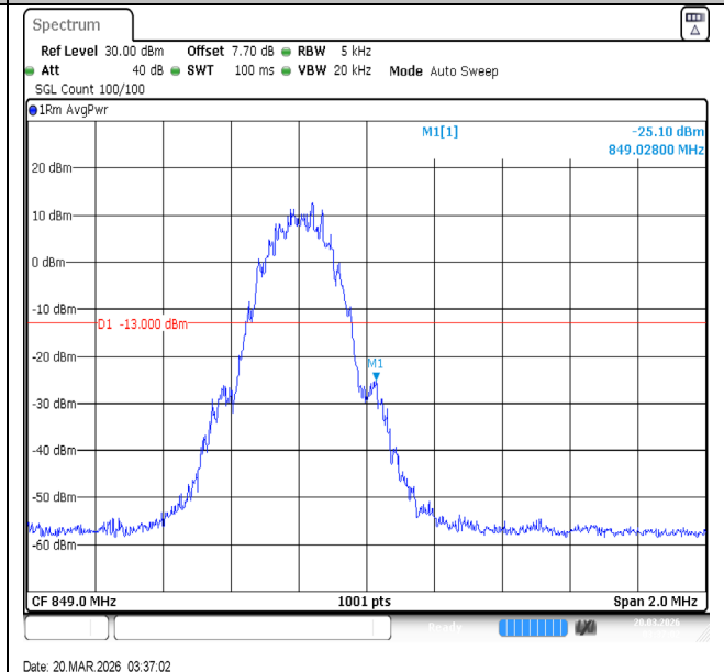
GPRS850-251-5-PASS
