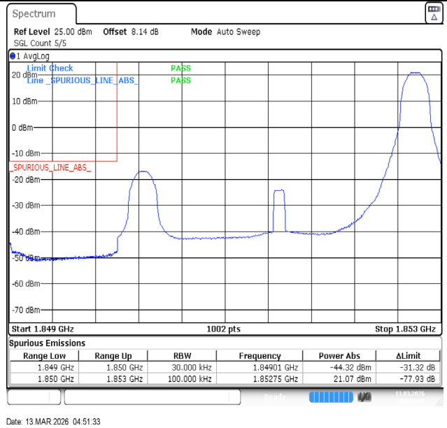
Band2-3MHz-QPSK-18615-1RB#14-PASS
