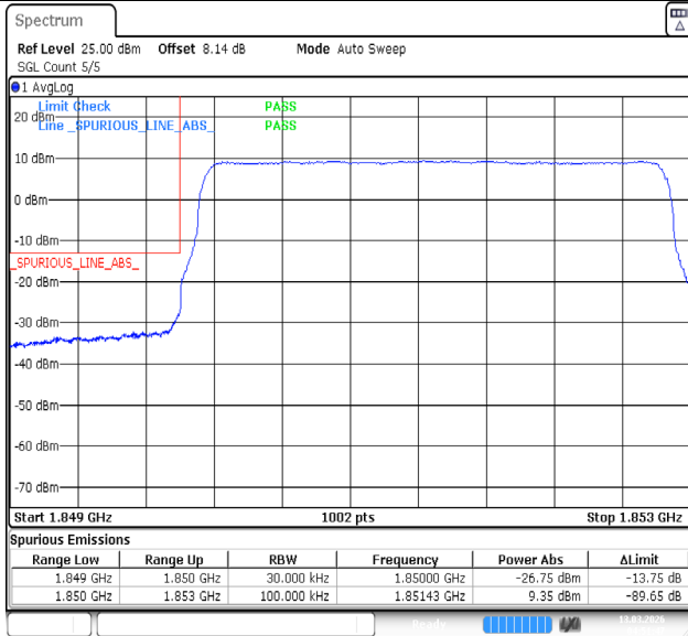
Band2-3MHz-QPSK-18615-15RB#0-PASS
