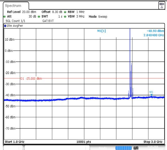
Band38-20MHz-QPSK-37850-1RB#0-1000~3000-PASS
