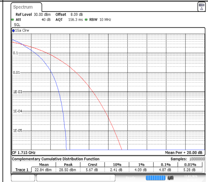
Band4-10MHz-QPSK-20000-50RB#0-PASS
