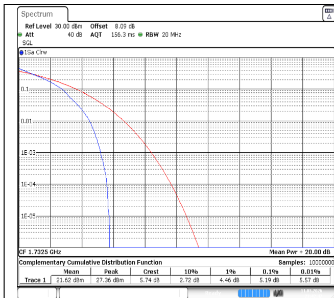
Band4-20MHz-QPSK-20175-1RB#0-PASS
