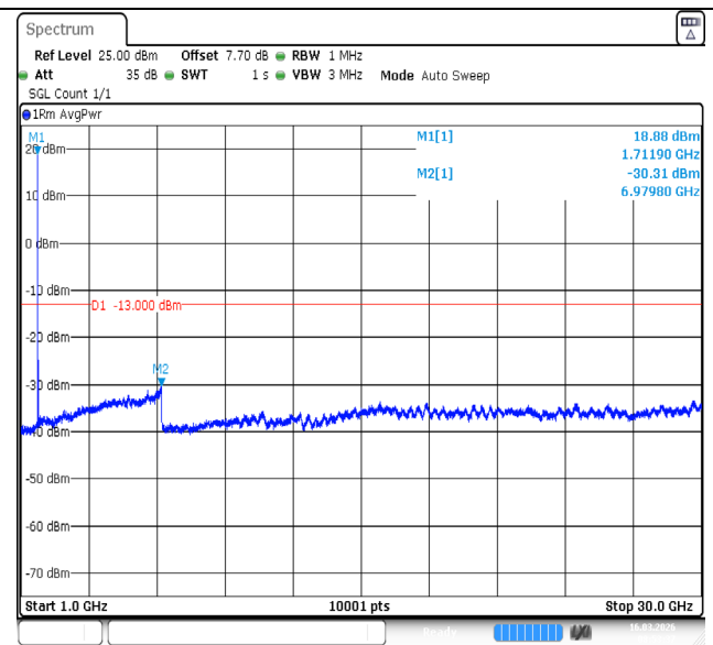
Band4-1312-1000~30000MHz-PASS
