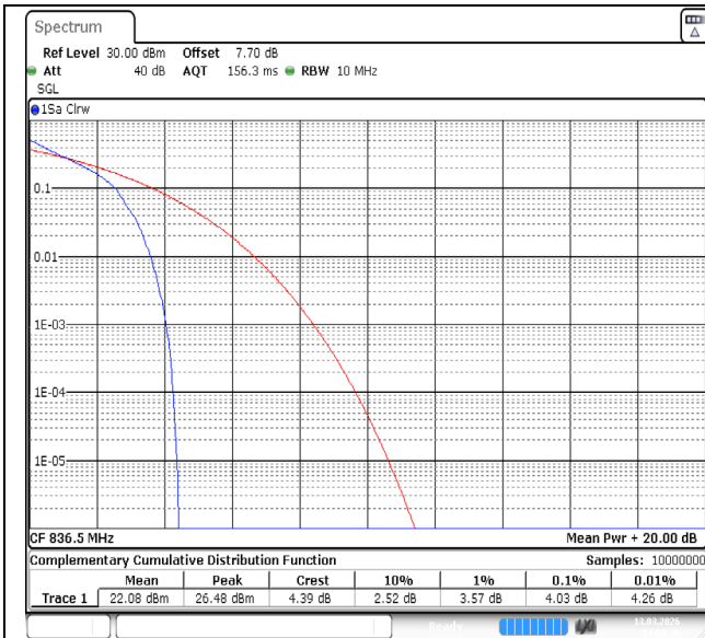
Band26(824-849)-10MHz-QPSK-26915-1RB#0-PASS
