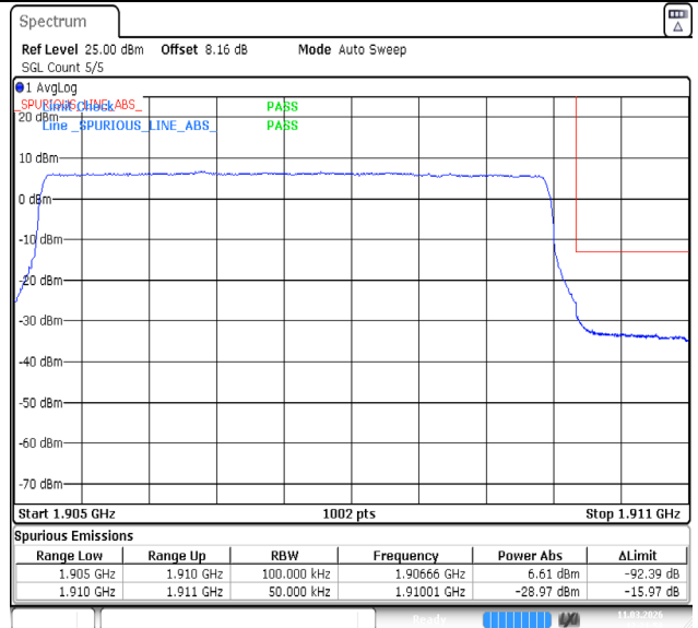
Band2-5MHz-QPSK-19175-1RB#0-PASS
