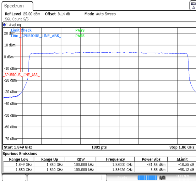
Band2-10MHz-QPSK-18650-50RB#0-PASS
