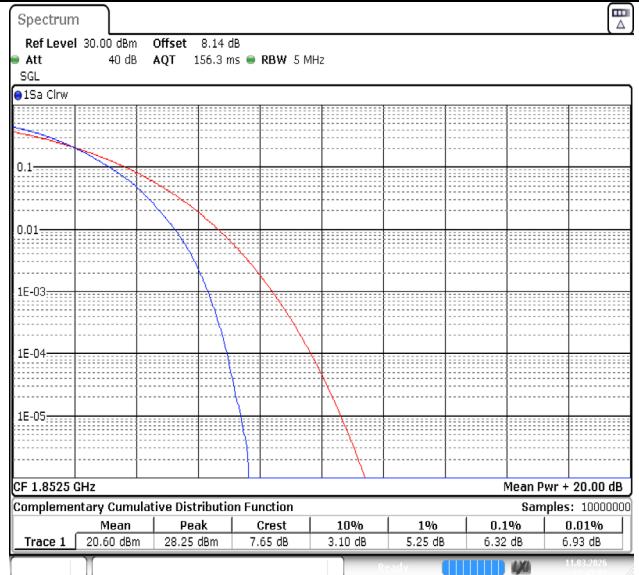
Band2-5MHz-QPSK-18625-25RB#0-PASS
