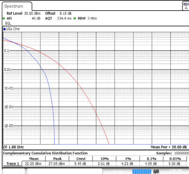
Band2-3MHz-QPSK-18900-1RB#0-PASS
