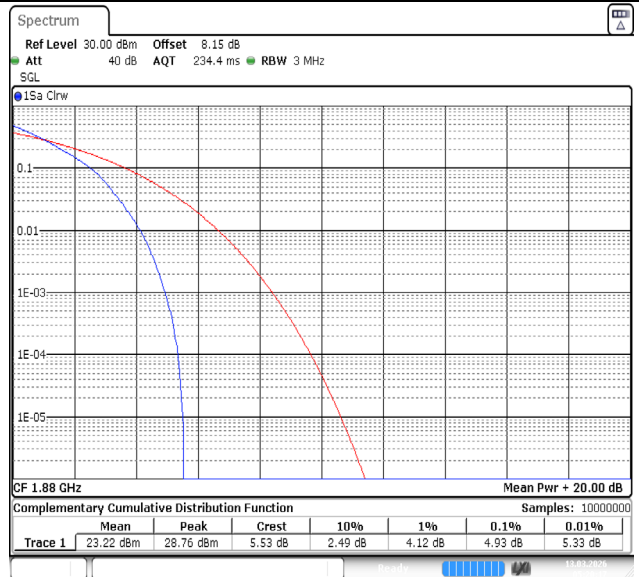
Band2-3MHz-QPSK-18900-15RB#0-PASS
