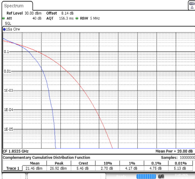
Band2-5MHz-QPSK-18625-1RB#0-PASS
