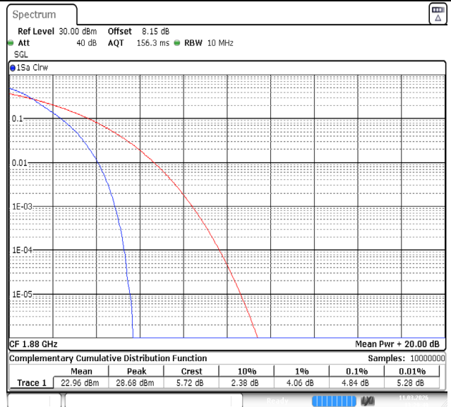
Band2-10MHz-QPSK-18900-50RB#0-PASS
