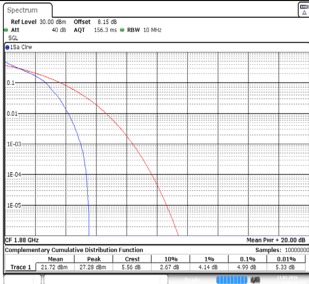
Band2-10MHz-QPSK-18900-1RB#0-PASS
