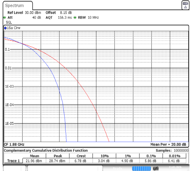
Band2-10MHz-16QAM-18900-50RB#0-PASS
